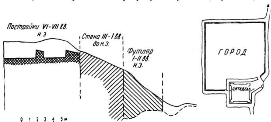
Рис. 6. Дэльверзинтепа. Разрез стены цитадели и схематический план.
