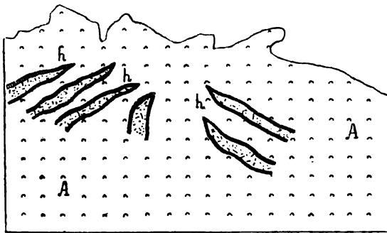
A — фельзитовый порфиръ съ кварцевыми и баритовыми жилами hh, пропитанными свинцовымъ блескомъ.
