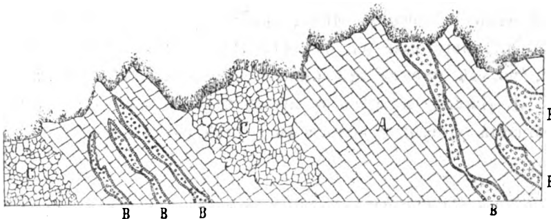
А — тонкослонстые известняки; В — рудныя жилы; С — осипь.
