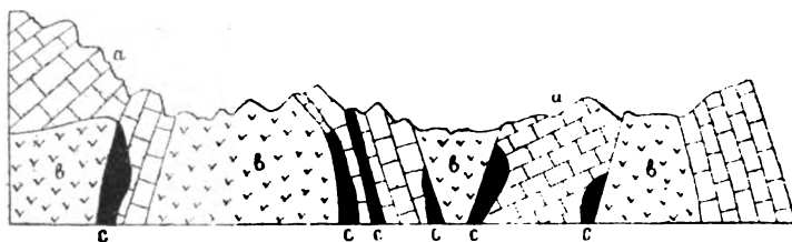
a — палеозойскій известнякъ, переходящій близъ контакта въ офикальцитъ; b — діоритъ c — рудныя жилы.
