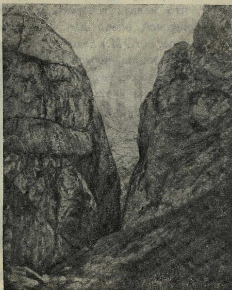
Алайский хребет. Ущелье в известняках.
