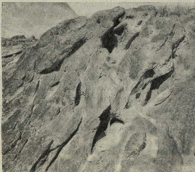
Формы ячеистого выветривания. Западный Памир. Алтын-мазар.
