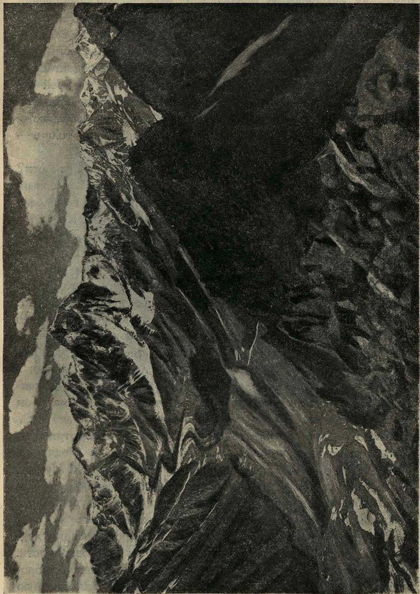
Типично-высокогорный рельеф хр. Петр I (около 5 900 м абс. выс.). Левее — пики Агасиц и Сахарной Головы. Ледник Финстервальдера — ледник туркестанского типа.
