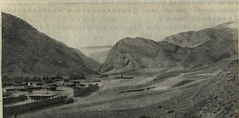
Вход в теснину р. Шахмардан.
