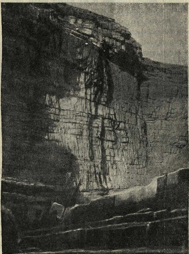
Толстоплитчатые известняки Кугитанг-тау.
