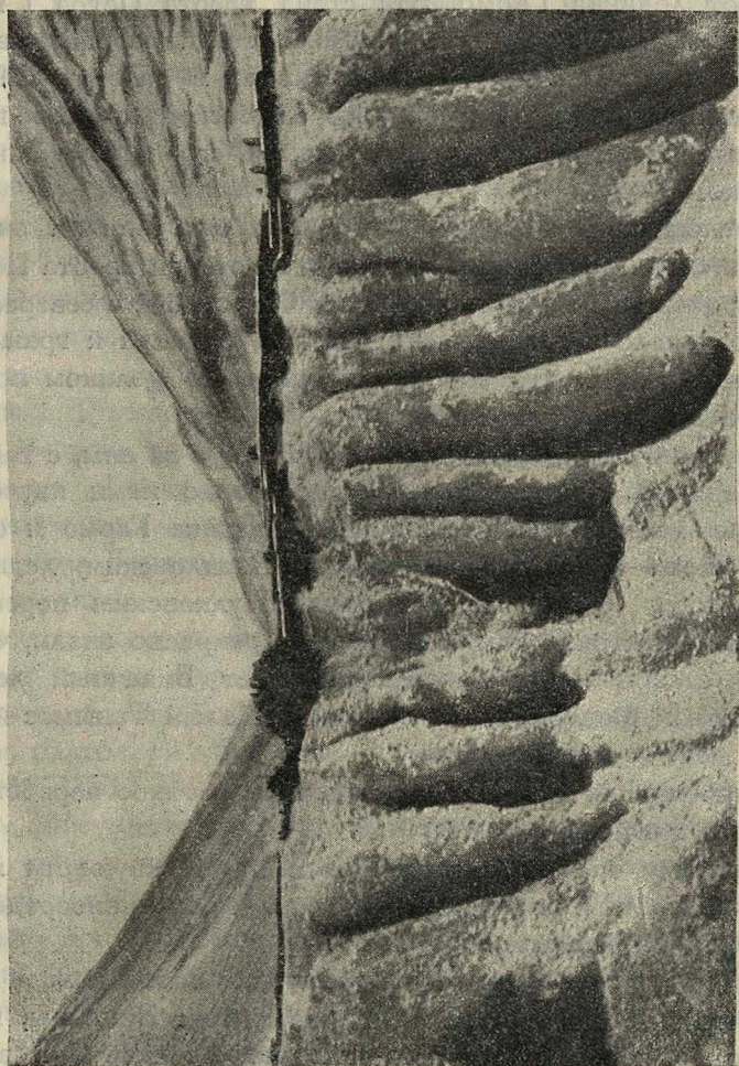
Террасы верховья р. Зеравшан.
