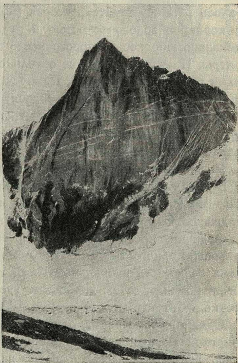
Сеть пегматитовых жил в гранитном пике Ак-су.
