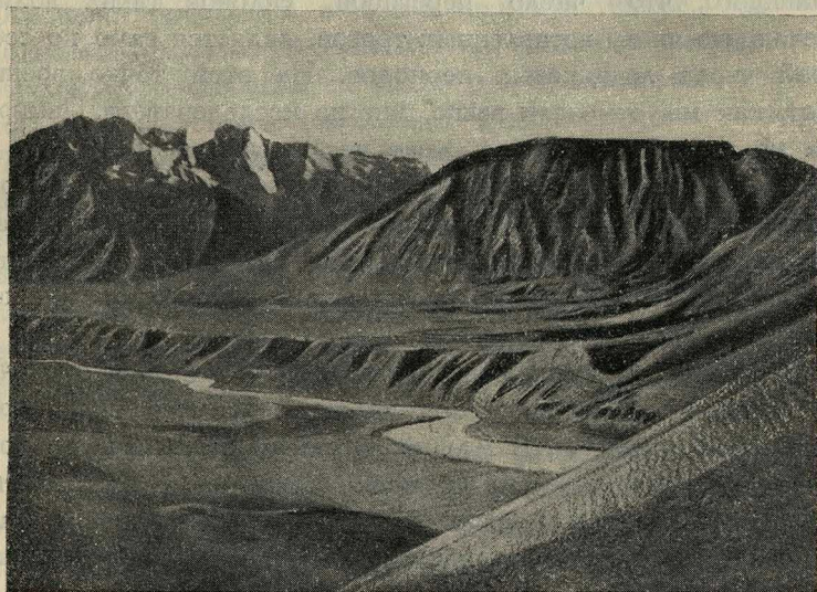
Останец высокой денудационной поверхности. Долина Сары-джага.
