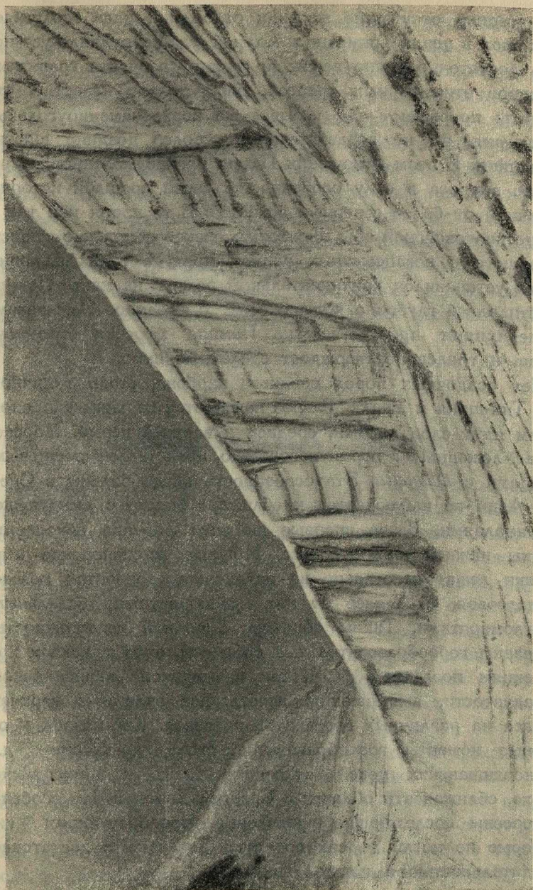
Ледник Ванч-дара, приток ледника Гармо.
