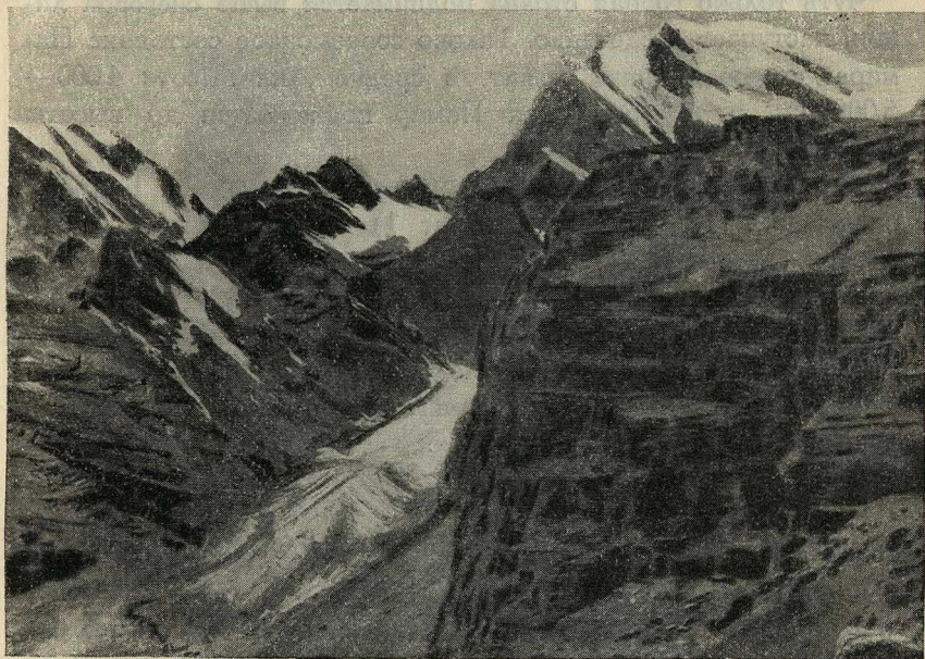
Ледник, стекающий с хр. Чимторга.
