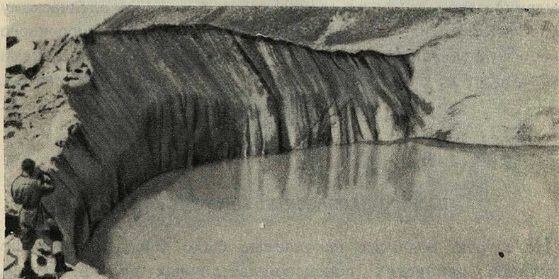
Ледниковое озеро у впадения ледника Фарахноу в Зеравшанский.
