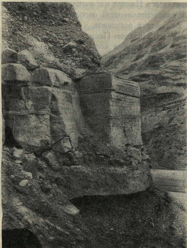
Слоистые озерные отложения в долине р. Мук-су.
