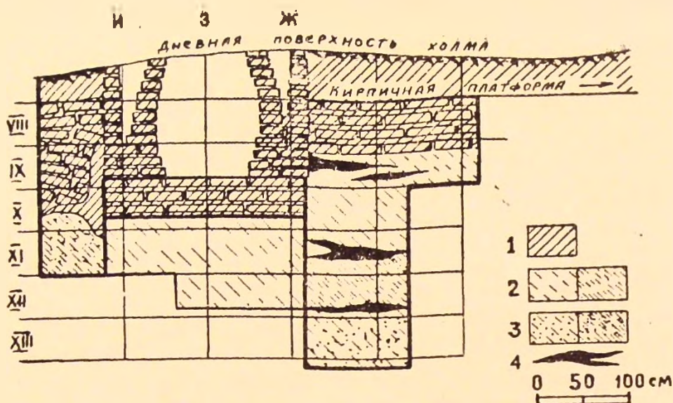
Рис. 2. Разрез парфянской керамической печи Мерва III в. н. э. 1—сырцовый кирпич /разрушенный и в кладках/; 2—глина с зольными отвалами и фрагментами керамики и костей; 3—глино-песчаный слой с фрагментами керамики; 4—зольно-угольные слои.
