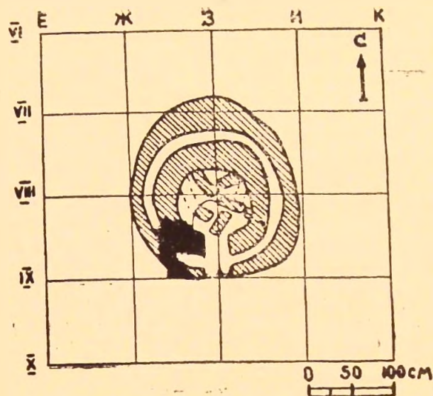
Рис. 1. Нарфинская керамическая печь Мериа III в. н. э. План в уровне дневной поверхности. (Обмер И. Ахрарова).
