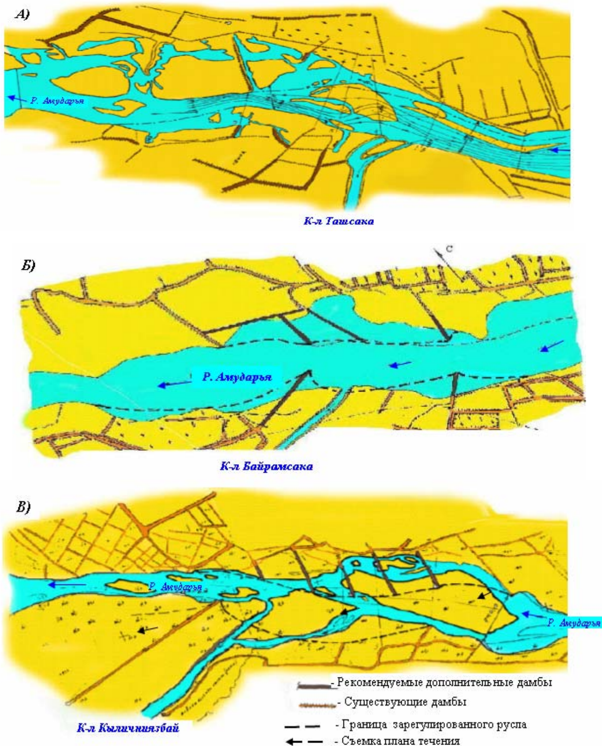
Рис.5 План – схемы исследуемых участков реки Амударьи: А- План течения потока на участке Ташсака; Б, В - Рекомендуемые варианты регулирования русла реки на участках Байрамсака и Кыличнийзбай.
