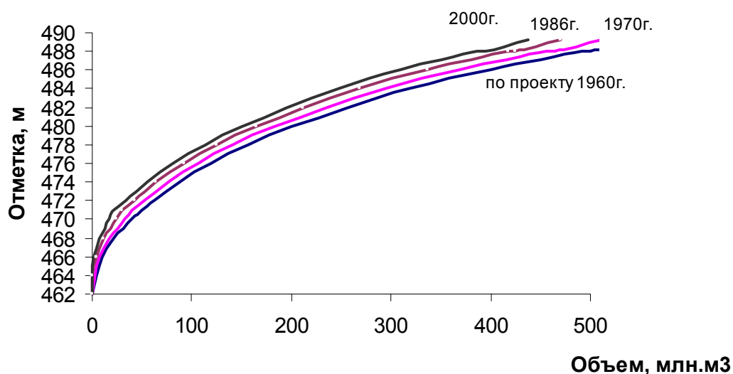
Рис. 3. Кривые зависимости объема Чимкурганского водохранилища от отметки уровня в нем на различные годы.
