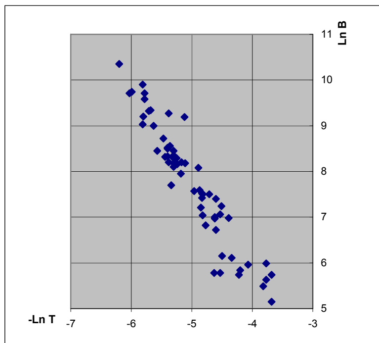
Рис. 4 - Зависимость сопротивления В от водопроводимости по данным откачек из скважин вертикального дренажа в долине р.Нижний Евфрат
