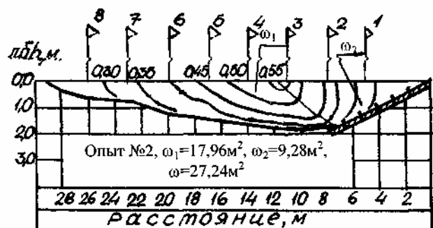
Рис.2. Распределение продольных скоростей потока в изотах (левая ветка Георгиевского магистрального канала, ПК91+50, ПК114)
