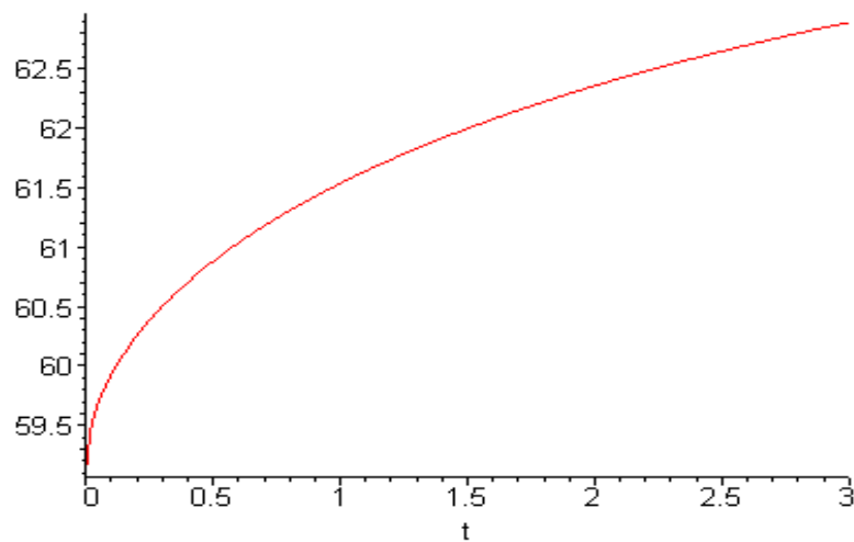
Рис. 3. Изменение грунтовой массы в течение времени
