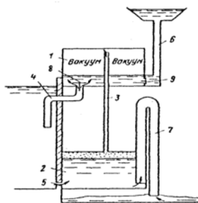
1 расм - Сифонли сув кўтаргич схемаси
