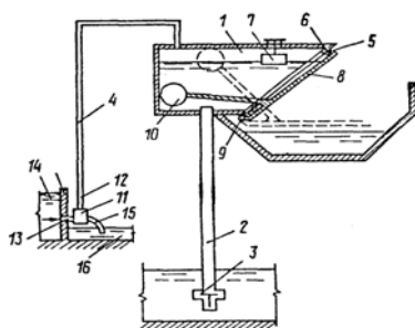
2 расм – Шиберли сув кўтаргич схемаси
