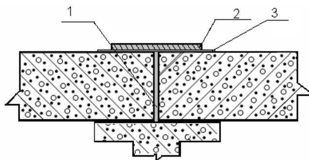
Рис. 1. Варианты уплотнения стыков-лотков
