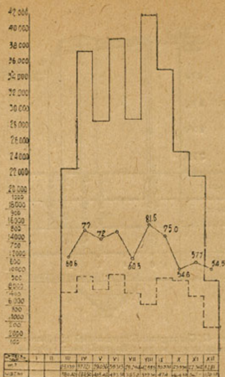
Черт. 44. График месячной выработки, чистого рабочего времени и часовой производительности экскаватора кл. 50—В № 9737 за 1929 г.
