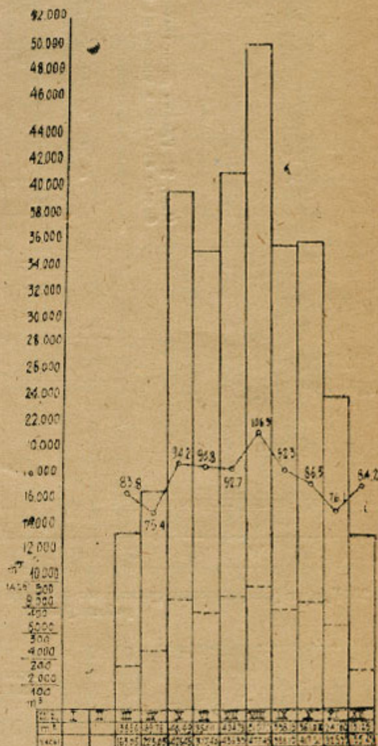
Черт. 19. График месячной выработки, чистого рабочего времени и часовой производительности экскаватора Бьюсайрус класс 50--В № 9736 за 1980 г.
