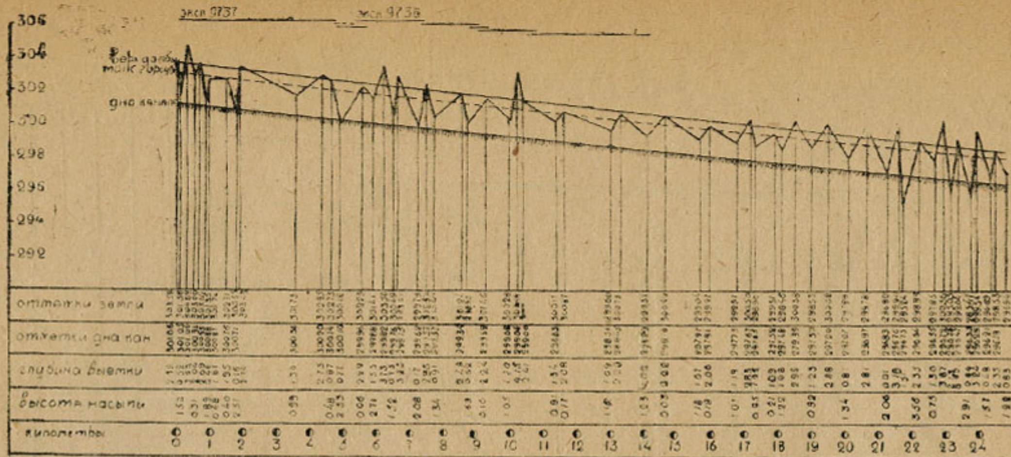
апр. 6. Сохранившийся профиль Правой ветви Маньчжурского канала. н. у. 0—250.
