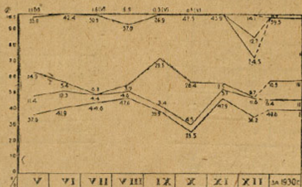
Черт. 73. График баланса суммарного рабочего времени по экскаватору кл. 7 М 851 по месяцам в 1930 г. и за все время работы по группам: I—чистое рабочее время; II—простой, свя- занные с производством работ (нормальная передвигка, холо- стой ход); III—оргпростой (планировка и расчистка, отсутствие горючего, воды, освещения); IV—простой, связанные с кон- струкцией машины (ремонт, набор воды и топлива, смазка, про- мывка котла и проч.) V—прочие простои; VI—дни отдыха
