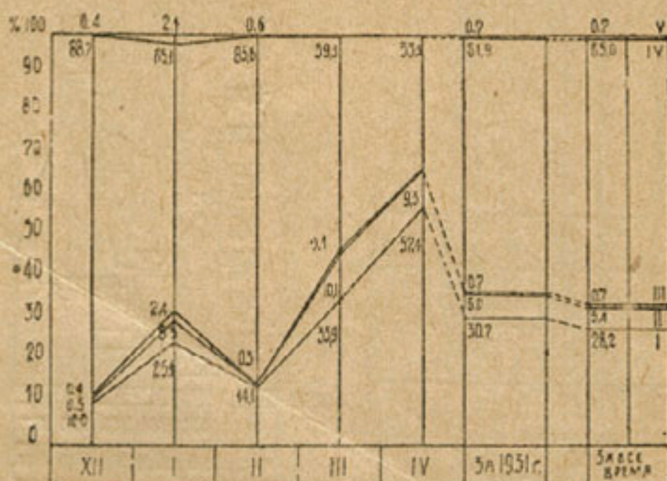
Черт. 87. График баланса суммарного рабочего времени по экс. Остип по месяцам в 1930-31 г и за все время работы по группам: I—чистое рабочее время; II—простой, связанные с производством работ (нормальная передвижка, холостой ход); III—оргпростой (планировка и расчистка, отсутствие горючего, воды, освещения); IV—простой, связанные с конструкцией машины (ремонт, набор воды и топлива, смазка, промывка котла и проч.); V—прочие простои; VI—дни отдыха
