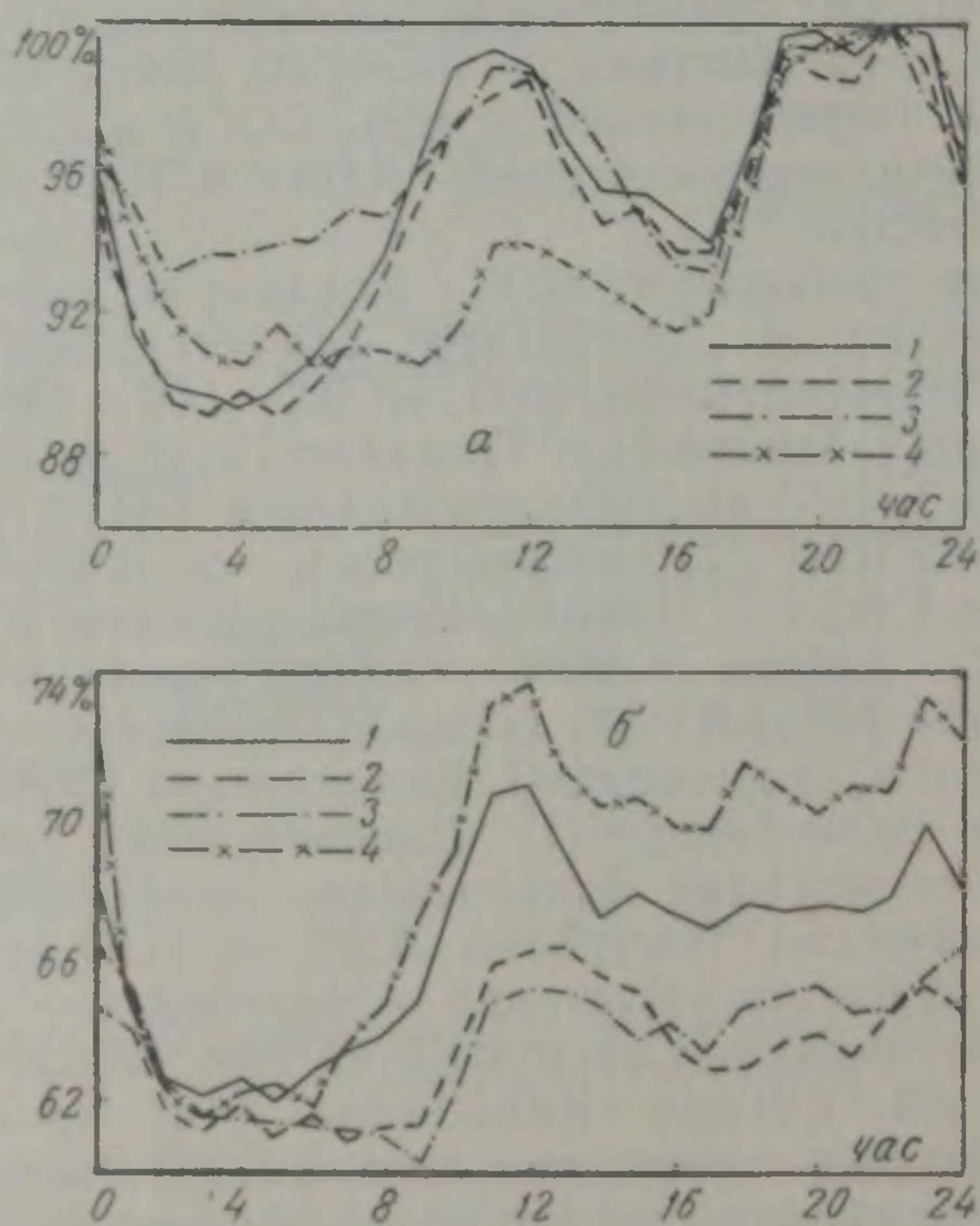
Рис. 4. Графики электрических нагрузок ОЭС Казахстана: а — за декабрь, б — июнь 1986 г. по средним характерным дням недели: 1 — рабочий день, 2 — суббота, 3 — воскресенье, 4 — понедельник.
