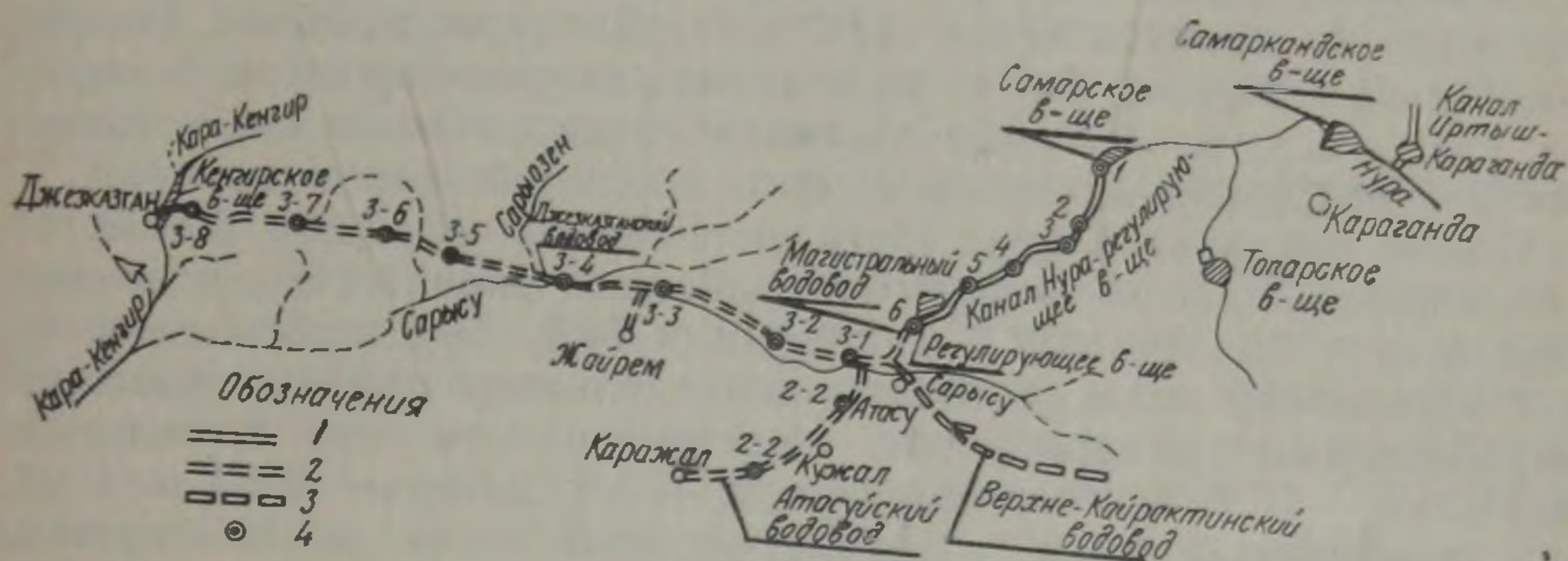
Рис. 6. Схема Джезказганской ветки канала Иртыш—Караганда: 1 — канал; 2 — водовод (трубопровод) на каналах и водоводах I очереди; 3 — водовод (трубопровод) второй очереди; 4 — насосные станции
