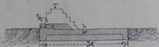
Черт. 29. — Поперечное сѣченіе плотины.
