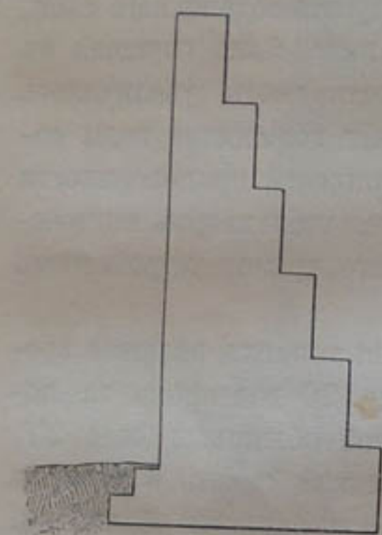
Черт. 140. — Поперечное сѣченіе подпорной стѣнки.
