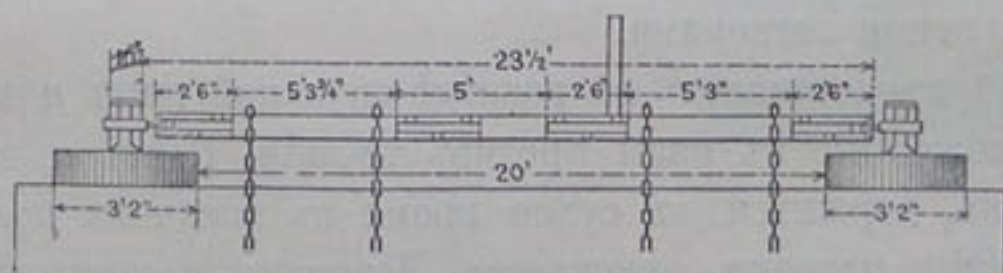
Черт. 59. — Ворота для подниманія затворовъ.
