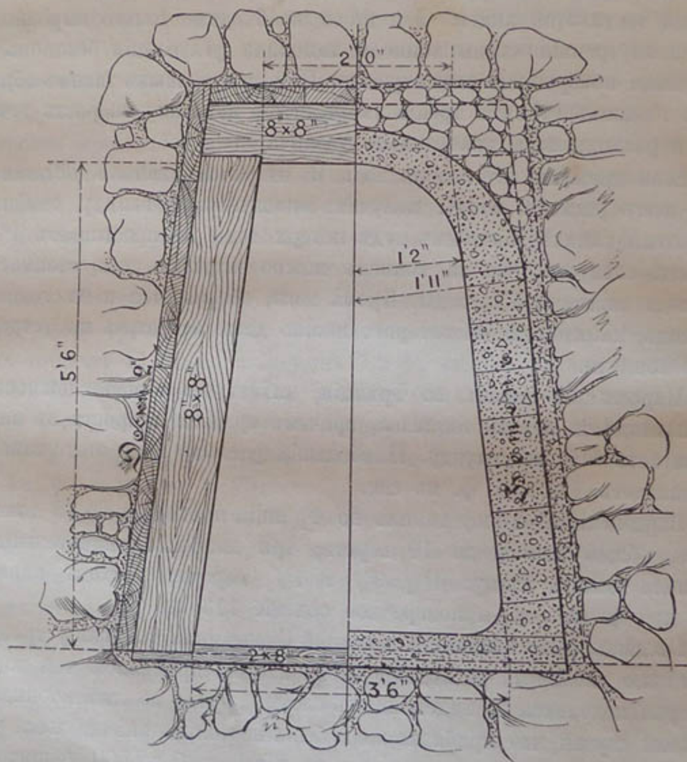
Черт. 139. — Поперечное сѣченіе туннеля Санъ-Антоніо.
