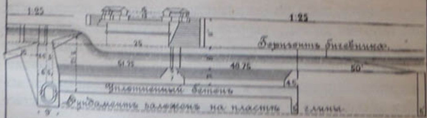
Черт. 120.—Вертикальный водослив на каналъ Basse Doab.
