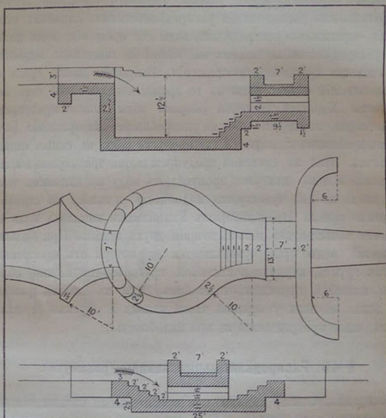
Черт. 144, 145 и 146. — Детали каналовъ-распределителей.
