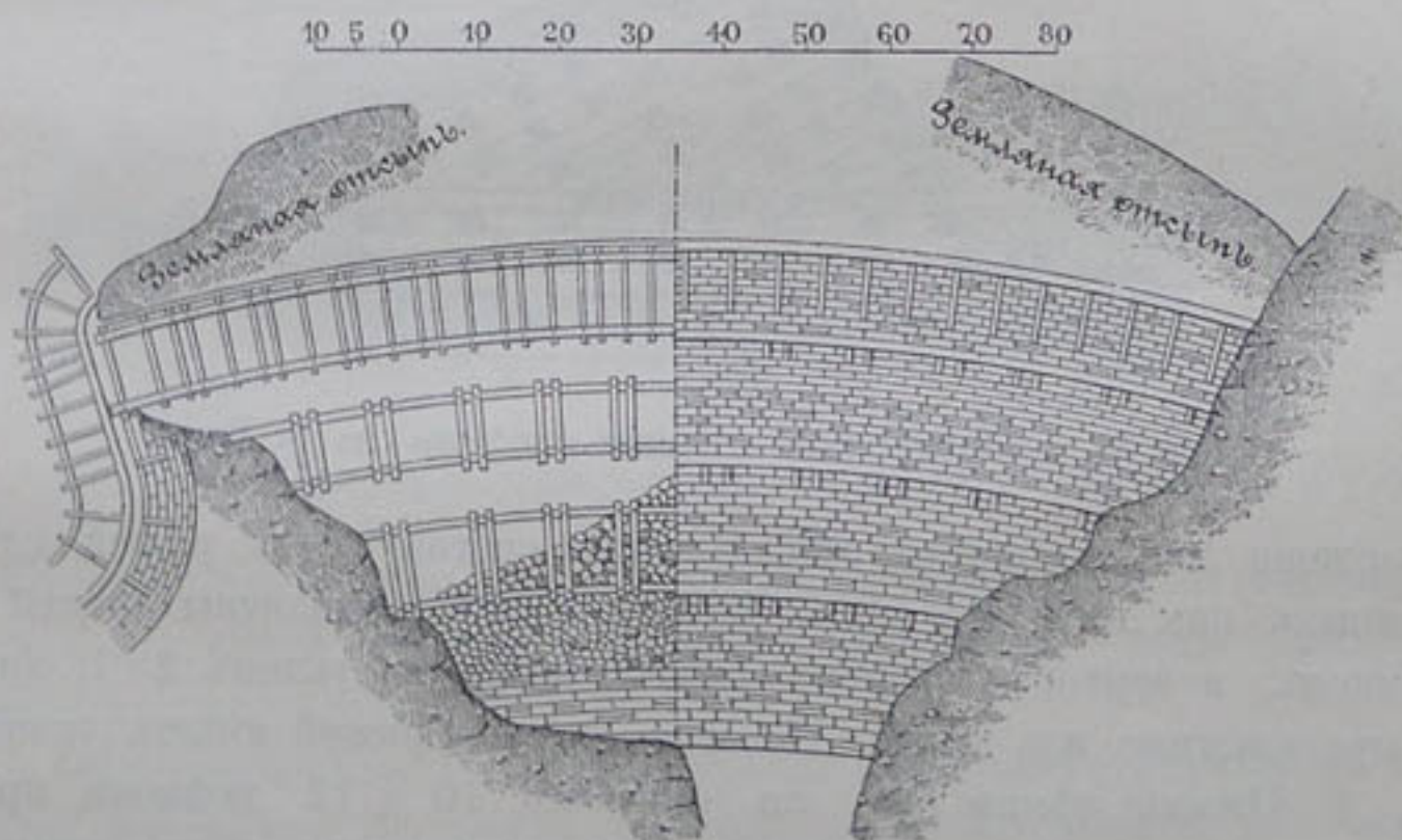
Черт. 23. — Планъ и горизонтальное сѣченіе.
