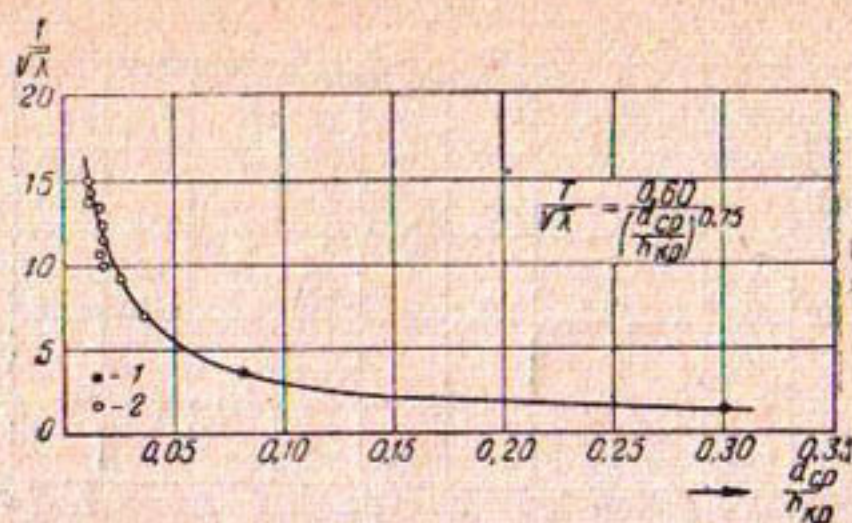
Рис. 9. График зависимости \frac{T}{\sqrt{\lambda}} = f\left(\frac{d_{cp}}{h_{кр}}\right) :
