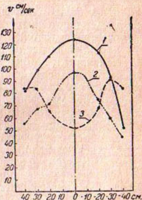
Рис. 6. Эпюры скоростей на удалении x = 350 м от сооружения при постоянном расходе и бытовых глубинах: 1 — при 12,8 м; 2 — при 15,0 м; 3 — при 16,0 м.
