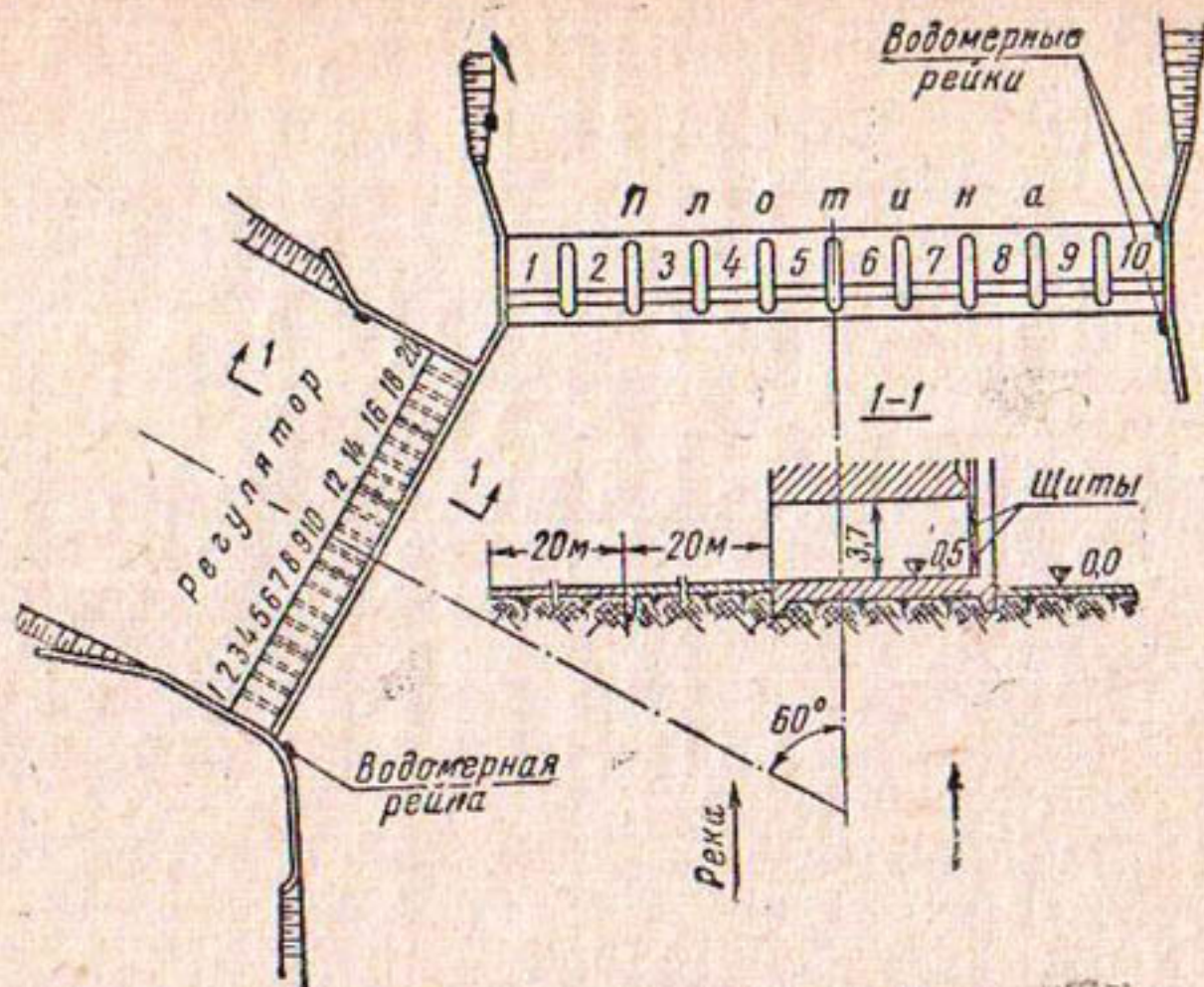
Рис. 2. Схема вододельного узла.
