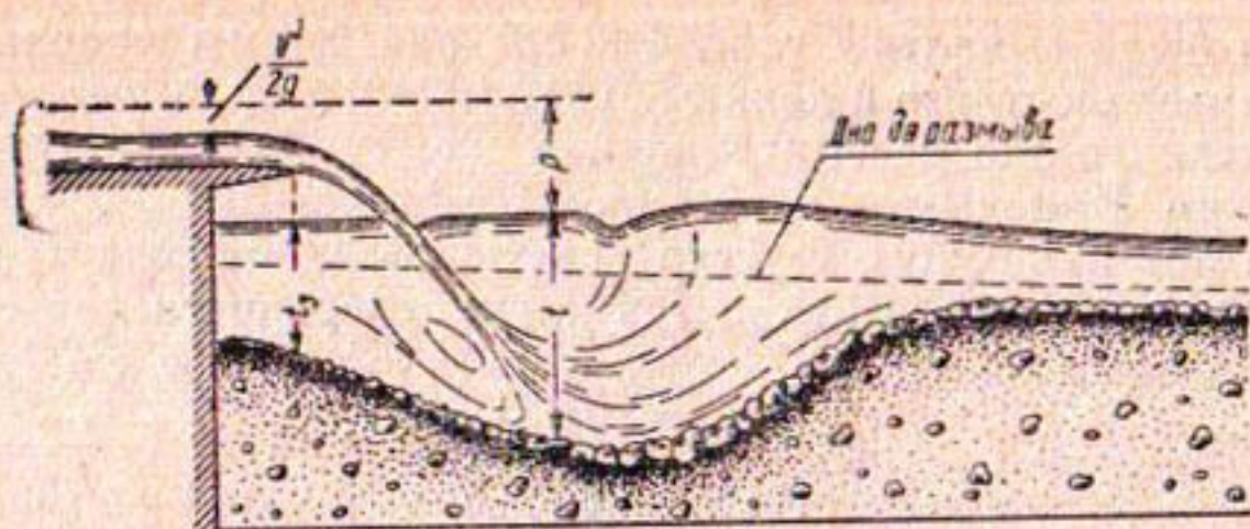
Рис. 2. Схема сопрягающего сооружения, исследованного в лабораторном лотке.
