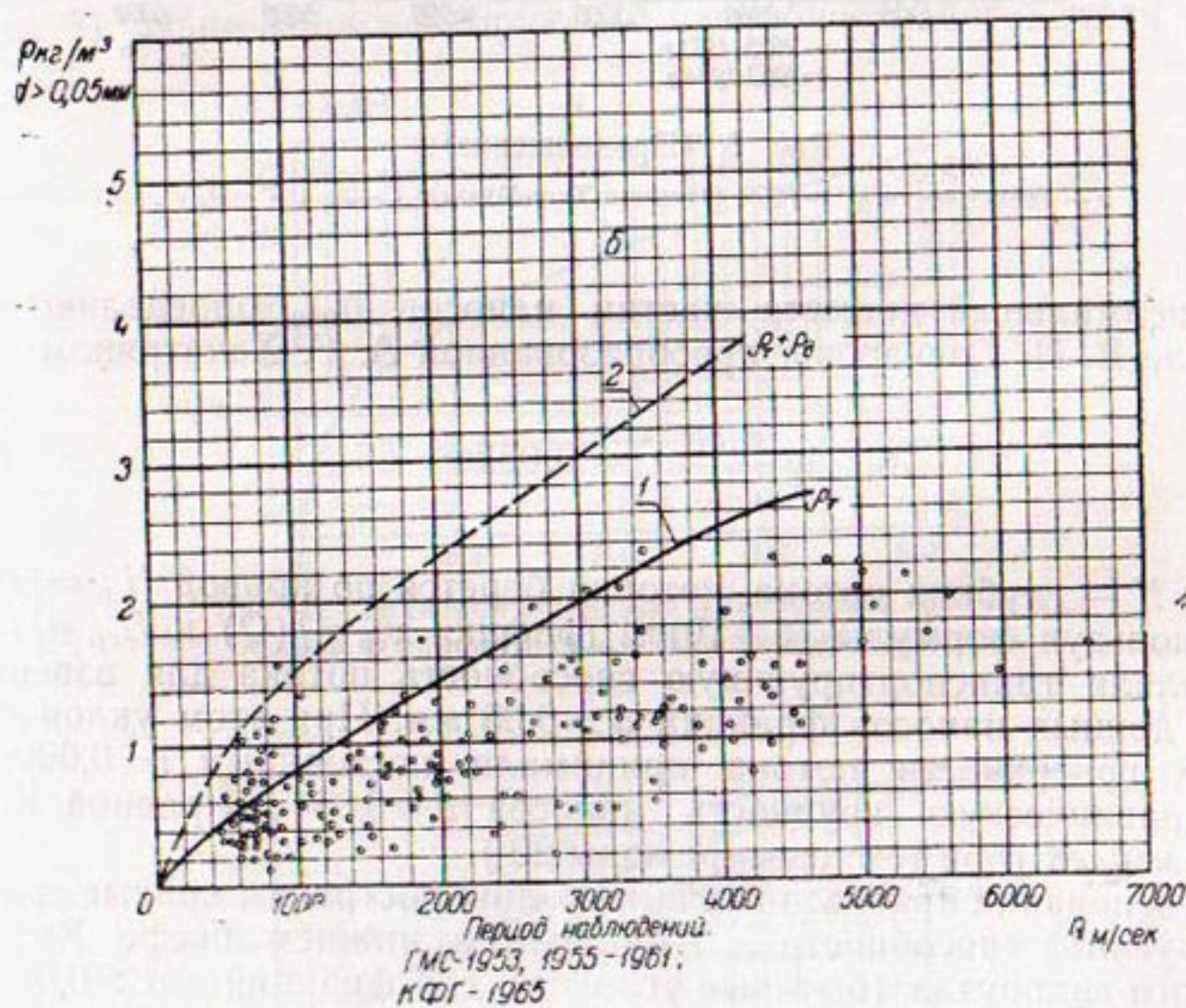
Рис. 5. Транспортирующая способность р. Амударьи для фракций d > 0,05 мм и данные наблюдений:
