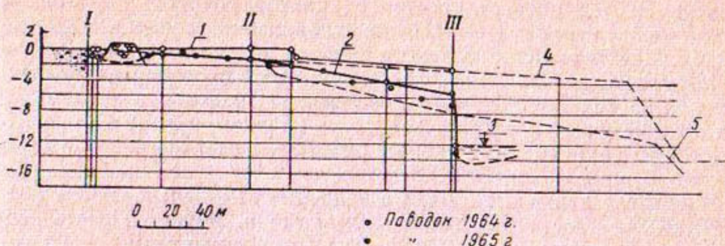
Рис. 2. Продольные профили отводящего канала и русло реки за ним:
