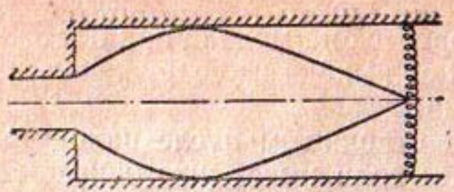
Рис. 4. Фронт гидравлического прыжка ниже «листа» растекающегося бурного потока.
