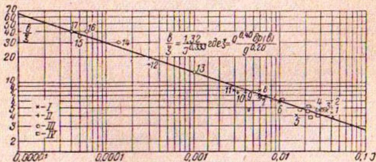
Рис. 12. Зависимость относительной ширины русла \frac{b}{z} от гидравлического уклона потока i :
