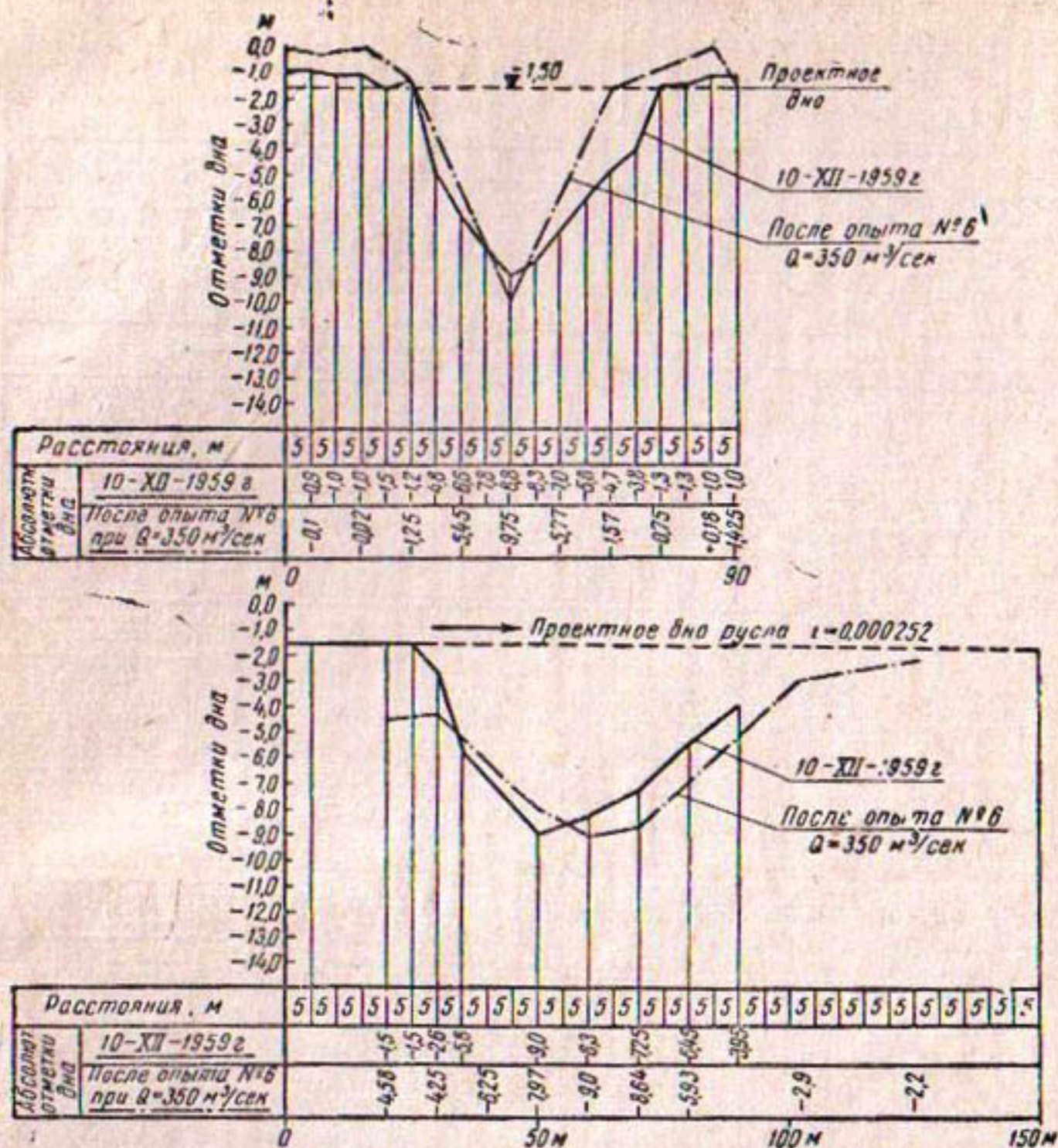
Рис. 5. Сопоставление лабораторных данных с натурными (при пропуске расхода через 8 центральных пролетов):
