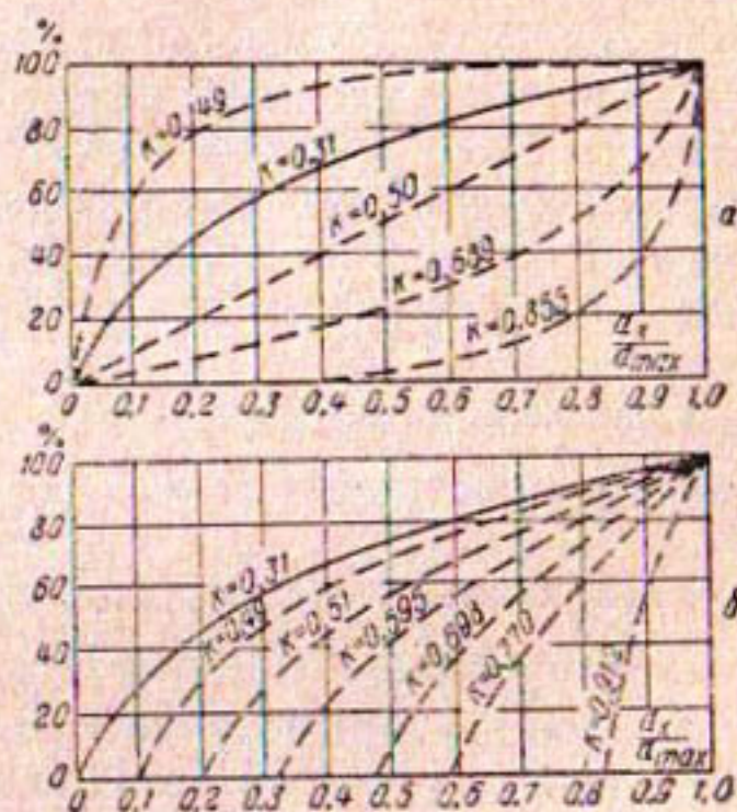
Рис. 3. Смеси частиц грунта, испытанные в опытах ( d_x — диаметр сита, через которое прошла данная фракция; d_{max} — максимальный диаметр частиц данной смеси грунта):
