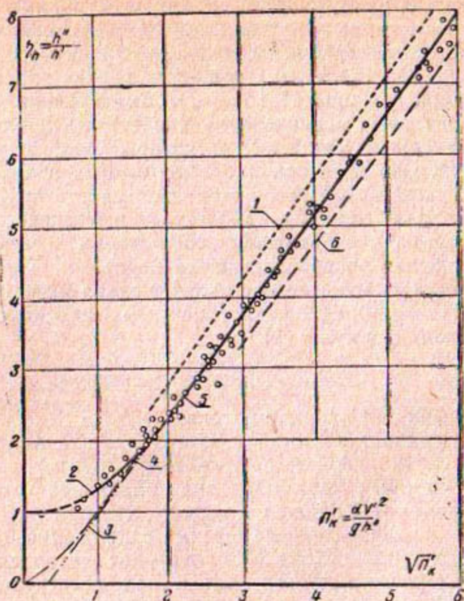
Рис. 1. Сравнение точности определения коэффициента сопряжения взаимных глубин \eta_k = \frac{h''}{h'} по различным формулам (опытные данные Бахметева, Гибсона, Эйнвахтера, Сметаны и др.):
