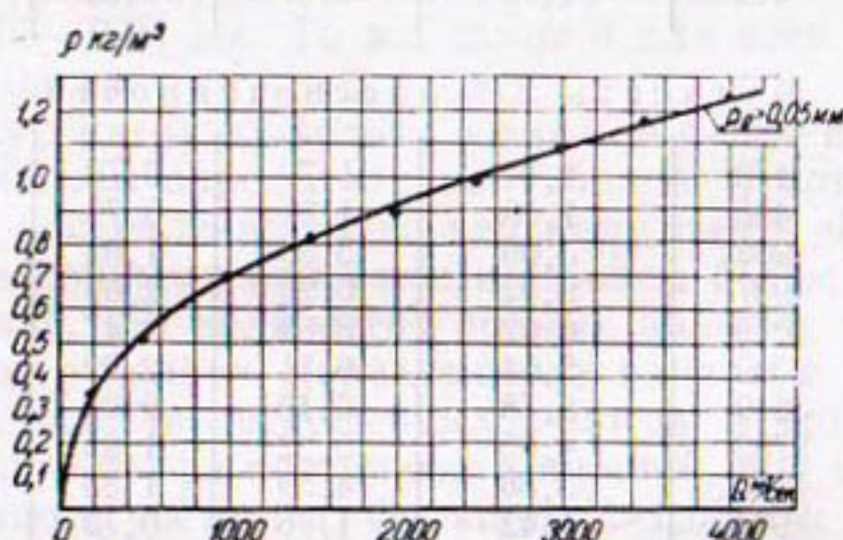
Рис. 6. Транспортирующая способность р. Амударьи в районе Кизыл-Аяка (донные наносы).
