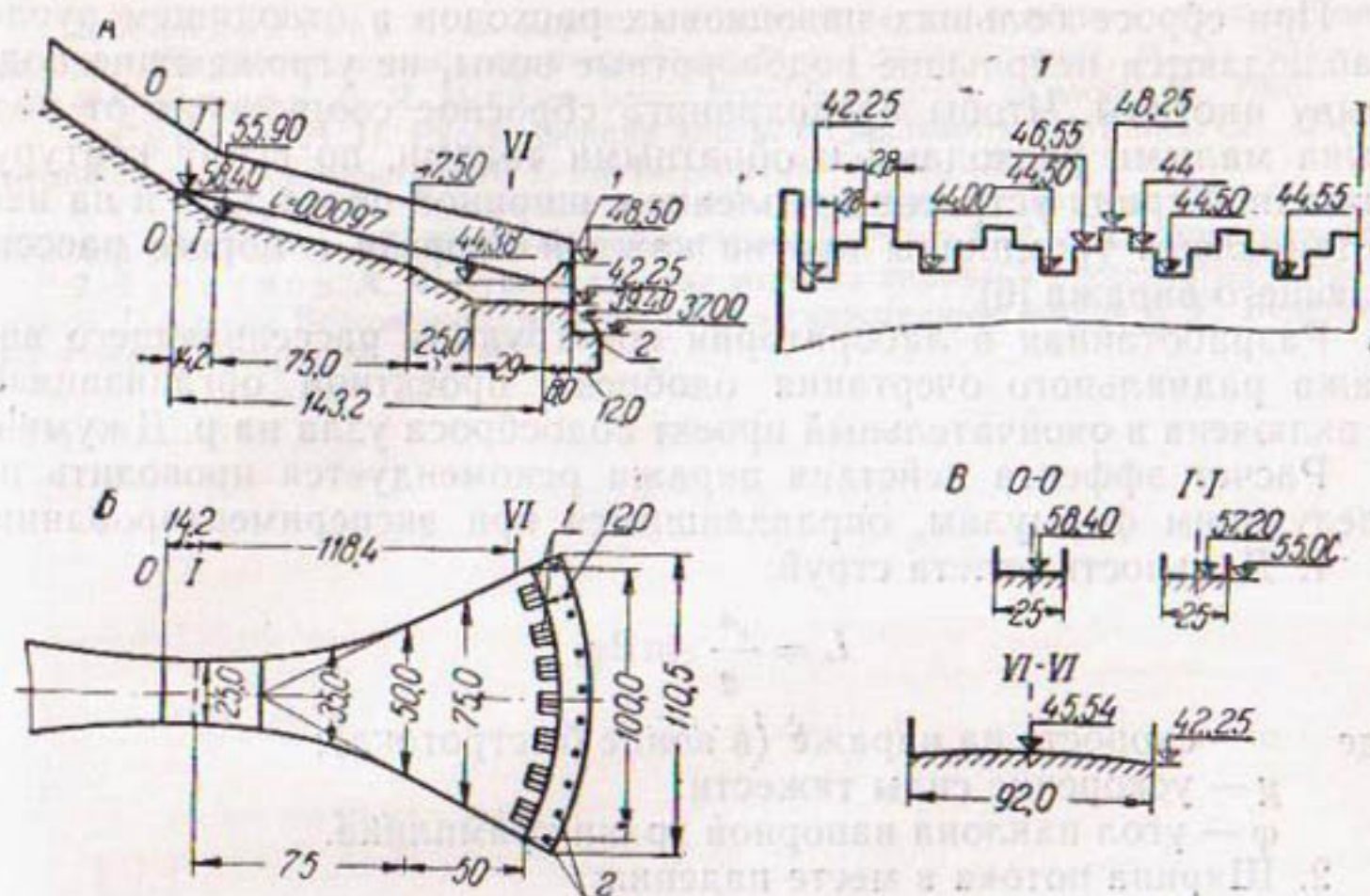
Рис. 3. Конструкция рассеивающего виажа водохранилища на р. Джумин: А — продольный разрез; Б — план; В — поперечные сечения.
