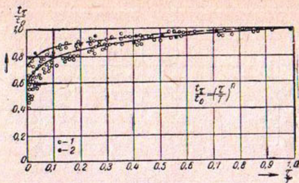
Рис. 10. График зависимости \frac{t_\tau}{t_0} = f\left(\frac{\tau}{T}\right) :
