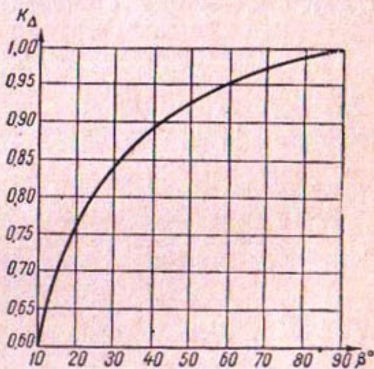
Рис. 1. Кривая зависимости относительной величины допускаемой (неразмывающей) донной скорости в воронке размыва K_\Delta от угла наклона входа струи \beta .
