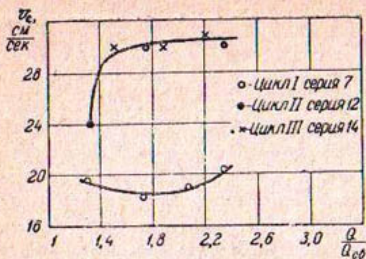
Рис. 5. График зависимости v_c от \frac{Q}{Q_{сб}} на период полуразмыва при d = 0,24 мм.
