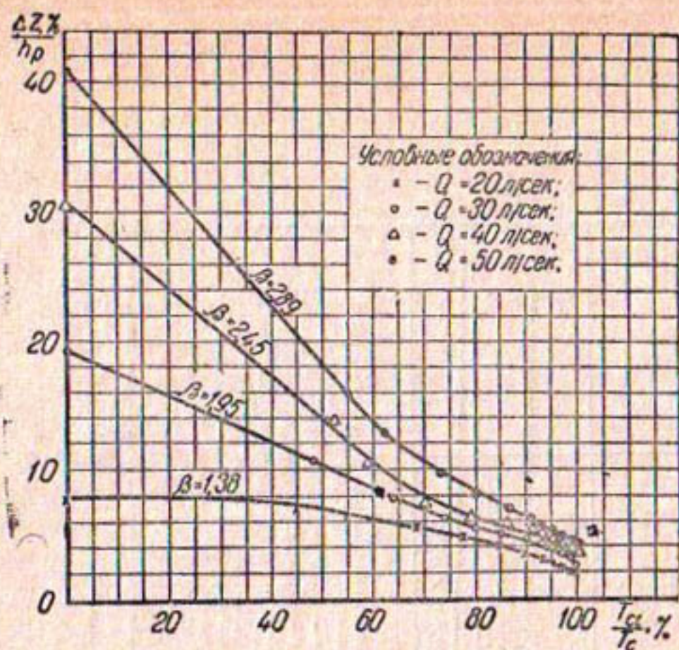
Рис. 3. График зависимости \frac{\Delta z}{h_p} от относительной глубины размыва \frac{T_{ct}}{T_c} при различных значениях стеснения
