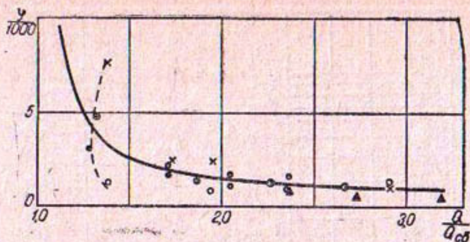
Рис. 9. График \varphi = \varphi \left( \frac{Q}{Q_{сб}} \right) .
