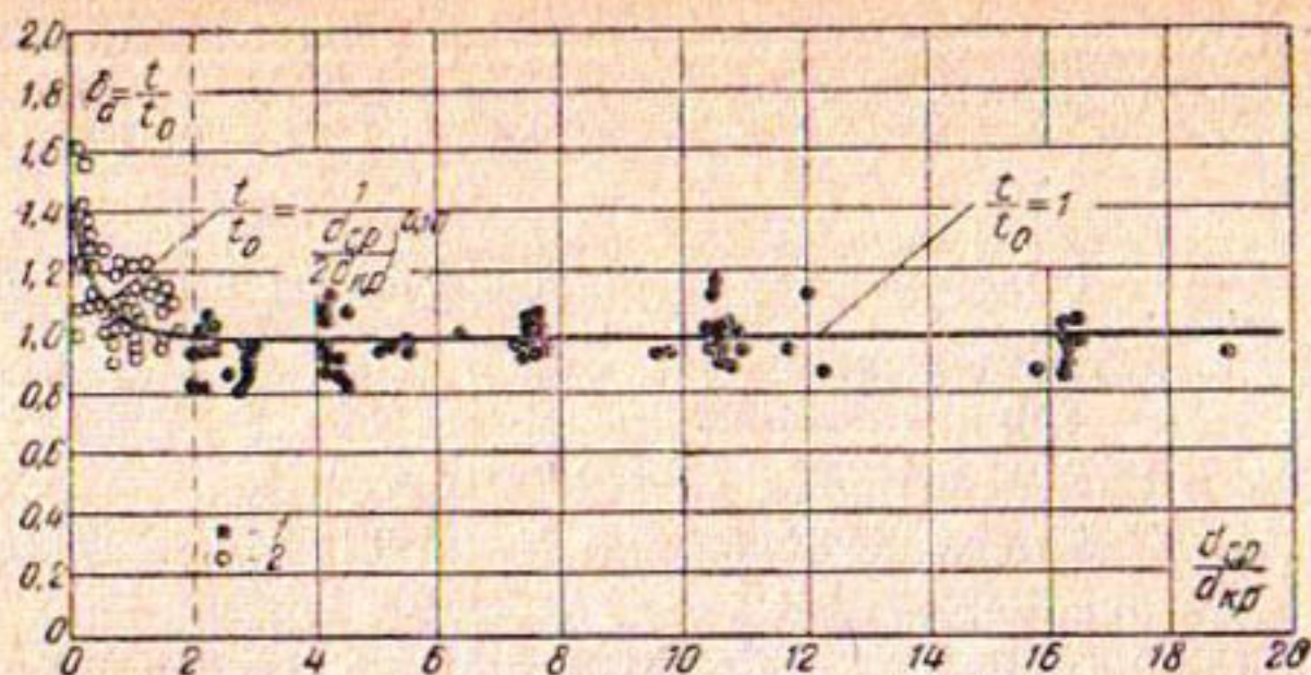
Рис. 6. График зависимости \frac{t}{t_0} = f\left(\frac{d_{cp}}{d_{кр}}\right) \cdot t — среднее значение фактической глубины, полученной в опытах на модели в условиях плоской задачи; t_0 — расчетная глубина, определенная по формуле (14): 1 — опыты при d_{cp} > 2 мм; 2 — опыты при d_{cp} < 2 мм.
