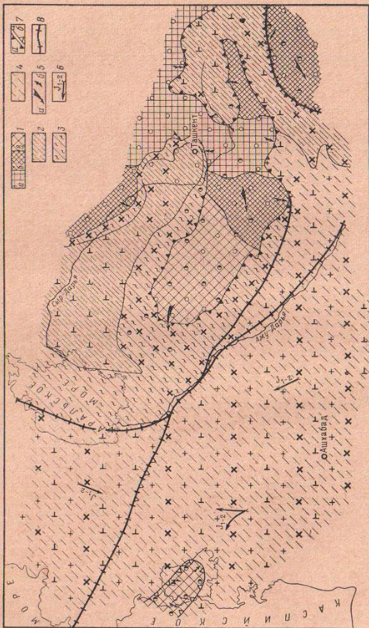
Рис. 6. Палеогеологическая схема ашг-альба
