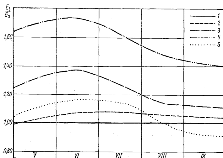
Рис. 11. Сезонное изменение переходных коэффициентов от показаний испарителей E_i к показаниям бассейна-эталоны E_э . 1 — бассейн-эталон, 2 — испаритель ГГИ-3000 в грунте, 3 — испаритель класса «А» на брусьях, 4 — испаритель ГГИ-3000 на брусьях, 5 — испаритель класса «А» в грунте.
