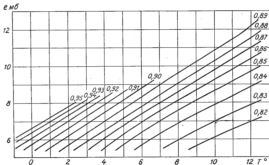
Рис. 64. График для расчета средних величин переходного (редукционного) коэффициента r = \frac{E_{20}}{E_{0.3}} (за теплый период) от показаний испарителя ГИ-3000 к показаниям испарительного бассейна площадью 20 м 2 по средним годовым значениям температуры и влажности воздуха, измеренным на высоте 2,0 м.
