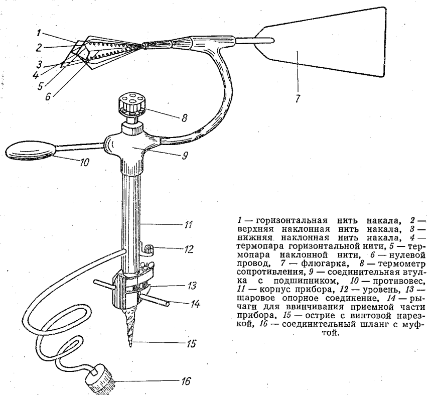
Рис. 14. Схема приемной части термоанемографа.
