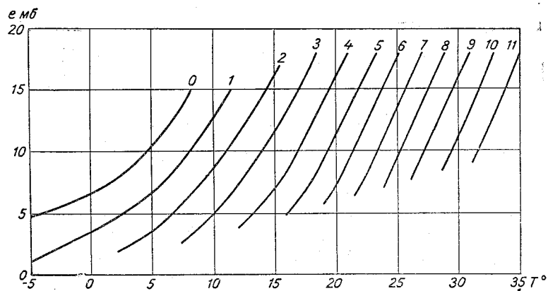
Рис. 60. График для расчета среднесуточных величин испарения (мм/сут.) с водноиспарительного бассейна площадью 20 м 2 по исправленным средним значениям температуры и влажности воздуха (т. е. с учетом величин \Delta T_v и \Delta e_v , отличных от величин \Delta T и \Delta e ).
