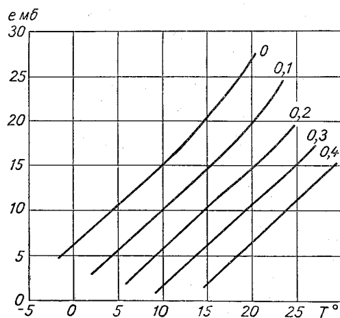
Рис. 59. Зависимость интенсивности испарения (мм/час) с водной поверхности бассейна площадью 20 м 2 от исправленных срочных значений температуры и влажности воздуха (т. е. с учетом величин \Delta T_v и \delta T_v , \Delta e_v и \delta e_v ).
