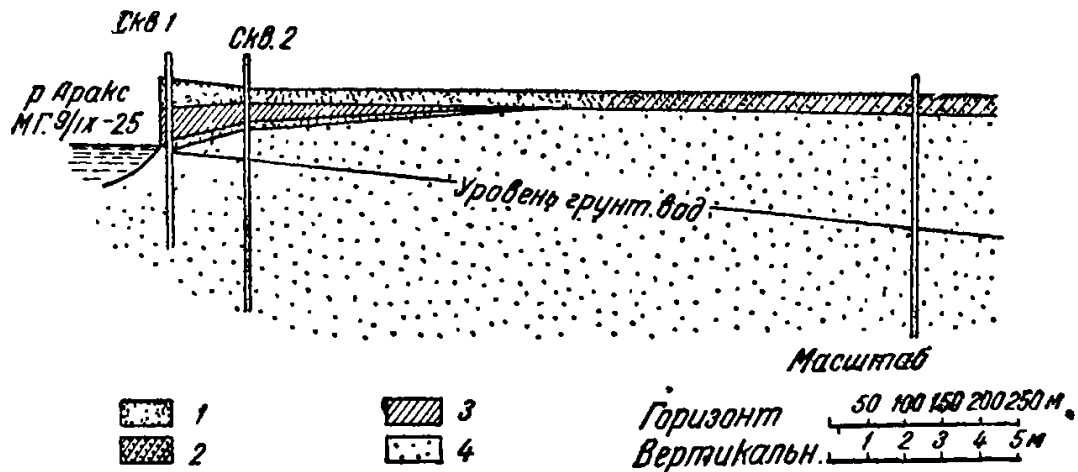
Рис. 1. Влияние р. Аракс на питание грунтовых вод прилегающих территорий (по Ф. П. Саваренскому):
