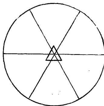
Рис. 4. Проекция элементов симметрии ( g_3P ) дитригональной пирамиды
