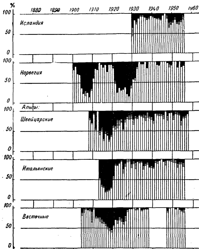
Рис. 105. Колебания ледников некоторых районов Европы в XX веке (по А. В. Шнитникову).
