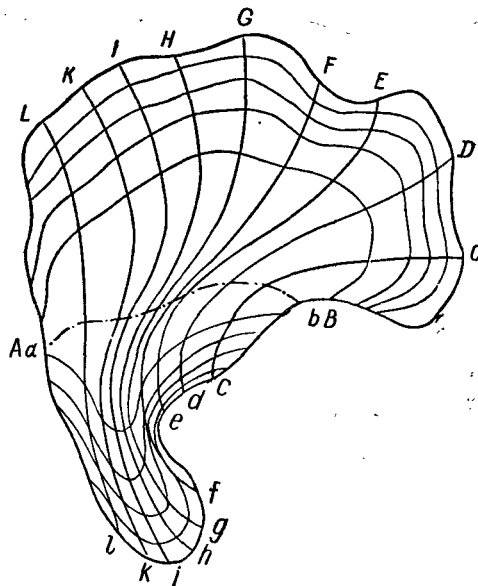
Рис. 62. Проекция линий течения на поверхность ледника (по С. Финстервальдеру):
