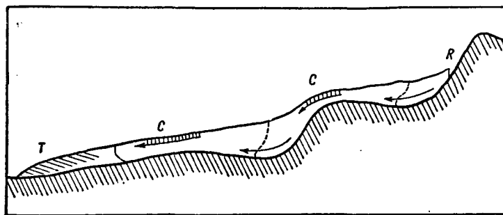
Рис. 52. Гипотетическое распределение наибольших скоростей в леднике (по Ф. Мэтису и др.):
