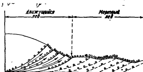
Рис. 130. Продольный профиль конца ледника. Перенос донной морены к поверхности ледника путем движения льда кверху вдоль плоскостей скалывания. В мертвом льду плоскости скалывания становятся недействующими (прерывистые линии) (по Р. Флинту)
