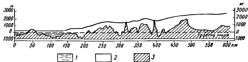
Рис. 143. Профиль ледникового щита в районе ст. Модхейм:
