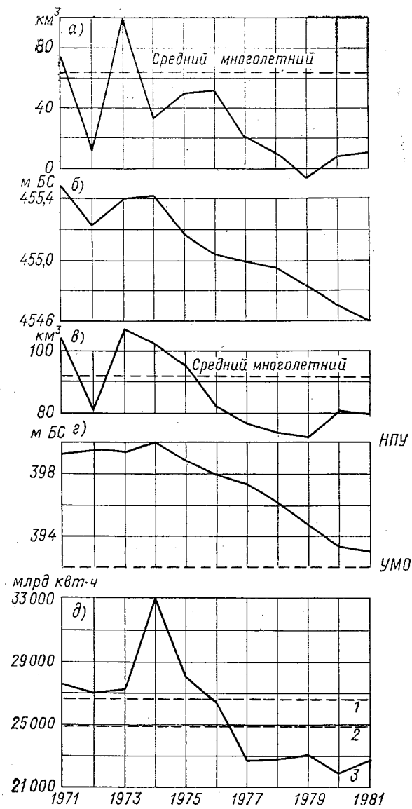
Рис. 7.4. Полезный приток (а, е) и ход уровня воды (б, г) оз. Байкал (а, б) и Братского водохранилища (е, г) и суммарная выработка электроэнергии Иркутской и Братской ГЭС (д).
