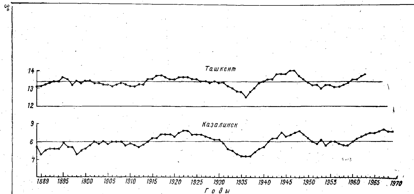
Рис. 3. Многолетний ход средних годовых скользящих 10-летних температур воздуха
