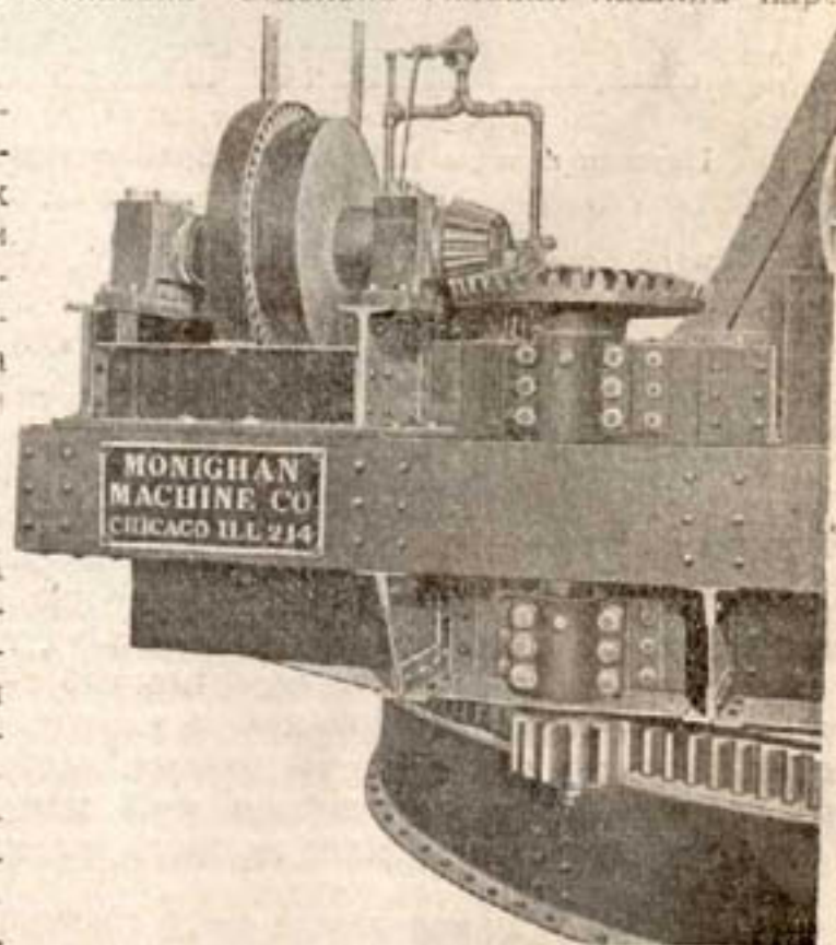
Рис. 15. Поворотный механизм экскаватора системы „Monighan“. Наверху вверху видна вращающаяся машина, показанная отдельно на рис. № 16.
