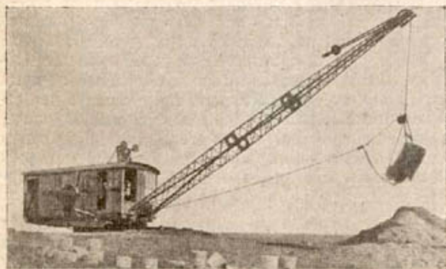
Рис. 12. Экскаватор фирмы „Monaghan“ на дренажных работах в штате Миннесота. Емкость черпака 1 куб. ярд. Длина стрелы 40 футов. Машина внутреннего сгорания.
