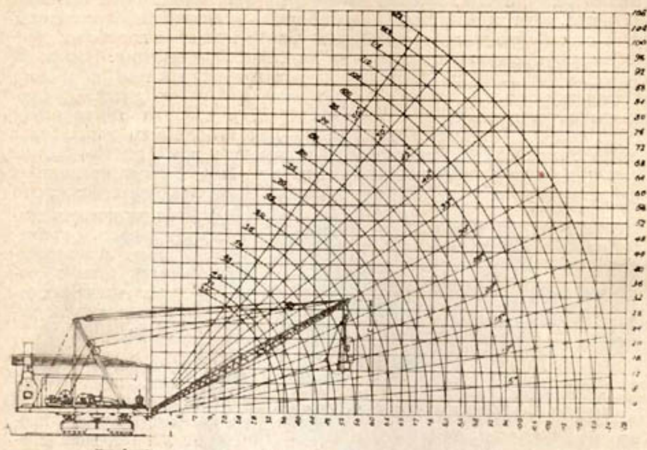
Черт. 26. Диаграмма для определения радиуса действия и предельной высоты кавальера для экскаваторов системы „Monighan“, для различных типов снарядов и различных углов наклона стрелы.
