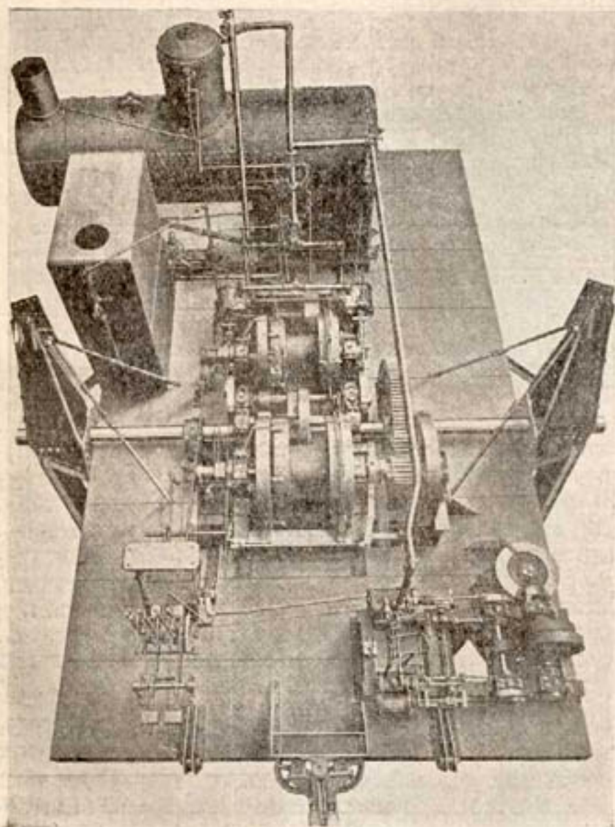
Рис. 13. Общее расположение механизмов парового экскаватора системы Мониган.
