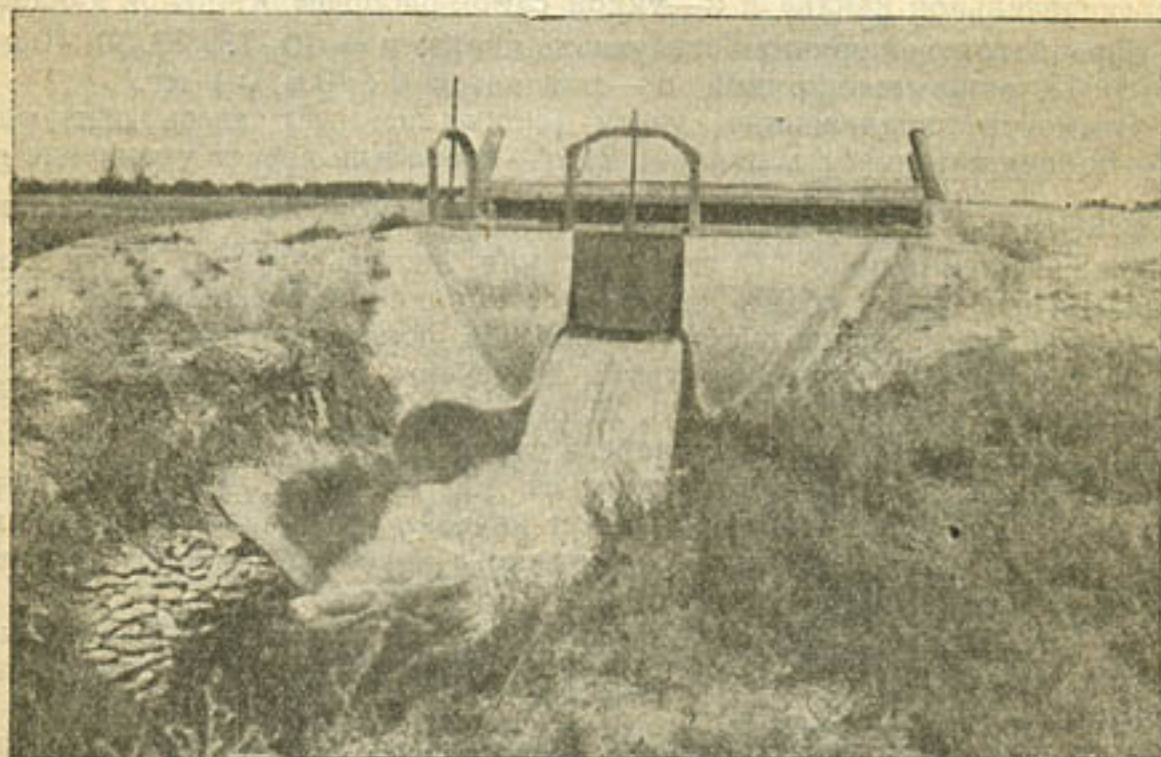
Подпорное сооружение в голове участка № 4.
