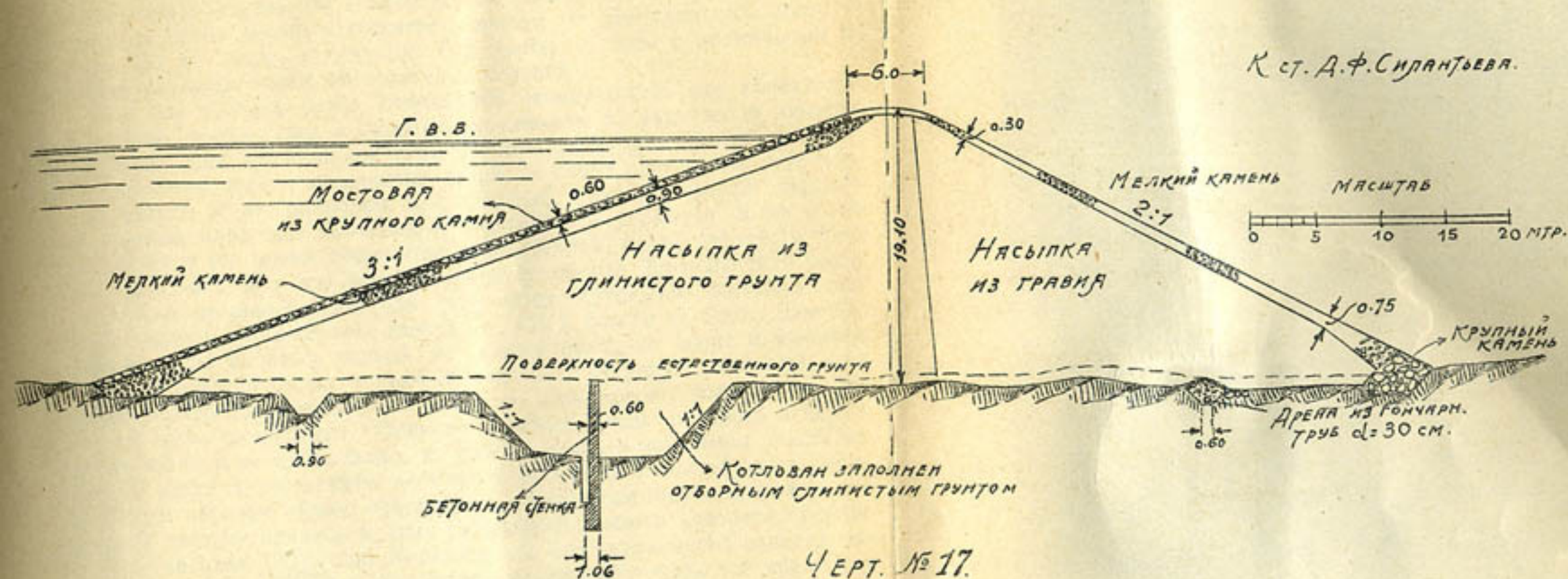
ПОПЕРЕЧНЫЙ РАЗРЕЗ ПЛОТИНЫ Kachess, Washington.
