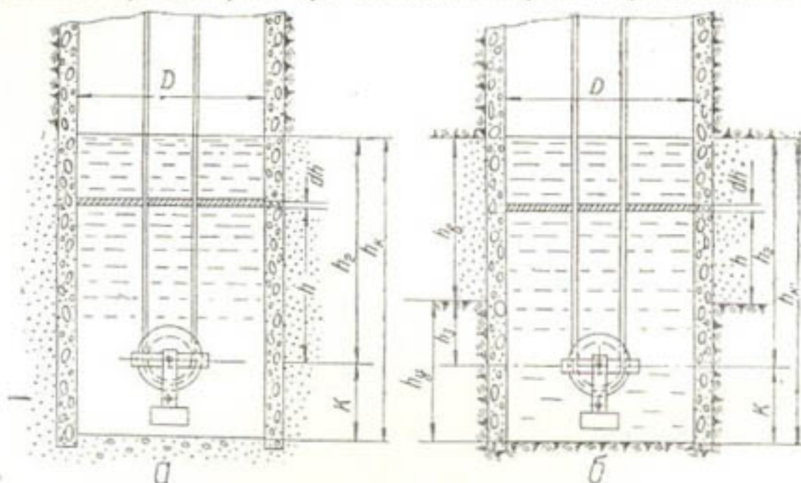
Рис. 1. Расчетные схемы.
