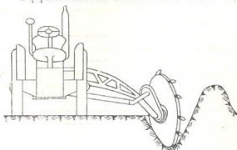
Рис. 9. Схема каналоочистителя Британского института сельскохозяйственной механики.
