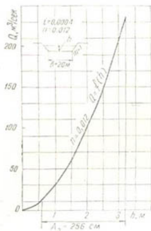
Рис. 3. Кривая зависимости расхода от наполнения в пункте установки теледатчика уровня на магистральном оросительном канале.
