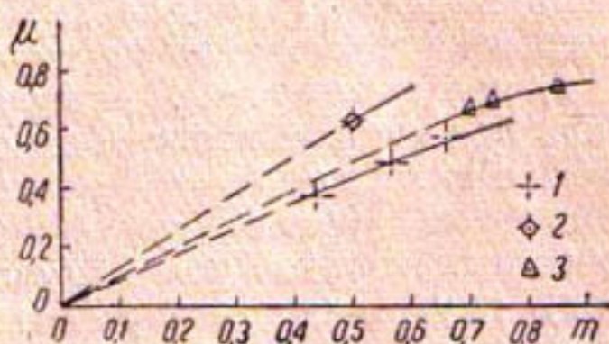
Рис. 4. Кривые зависимости коэффициента расхода \mu = f(m) системы от m : 1 — ТВР с кольцом; 2 — сужение типа Вентури; 3 — получилиндр.
