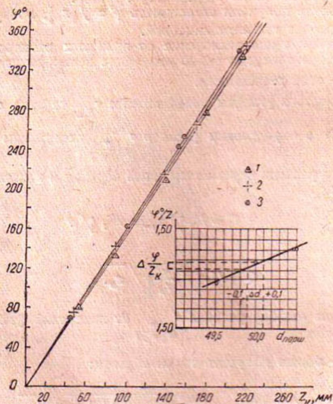
Рис. 4. График \varphi^\circ = f(z_k) при допусках в диаметре поршня \Delta d = \pm 0,5 мм:
