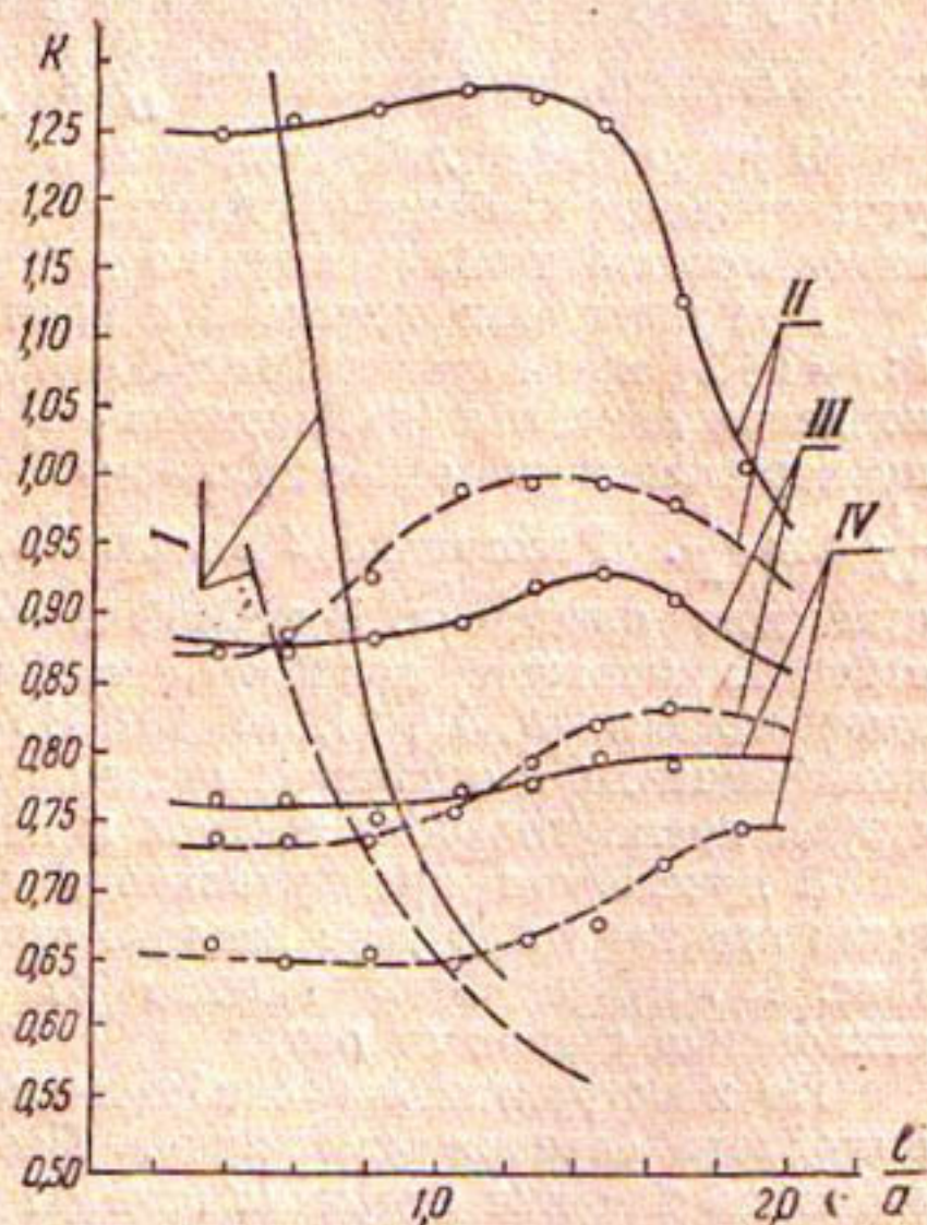
Рис. 3. График K = f\left(\frac{l}{a}\right) для прямоугольных приставок при различных \gamma^\circ (пунктиром для 12^\circ , прямой линией для 18^\circ ) и \theta = 45^\circ : I — зоны K = \text{const} , II — b:a=1 ; III — b:a=2 ; IV — b:a=3 .
