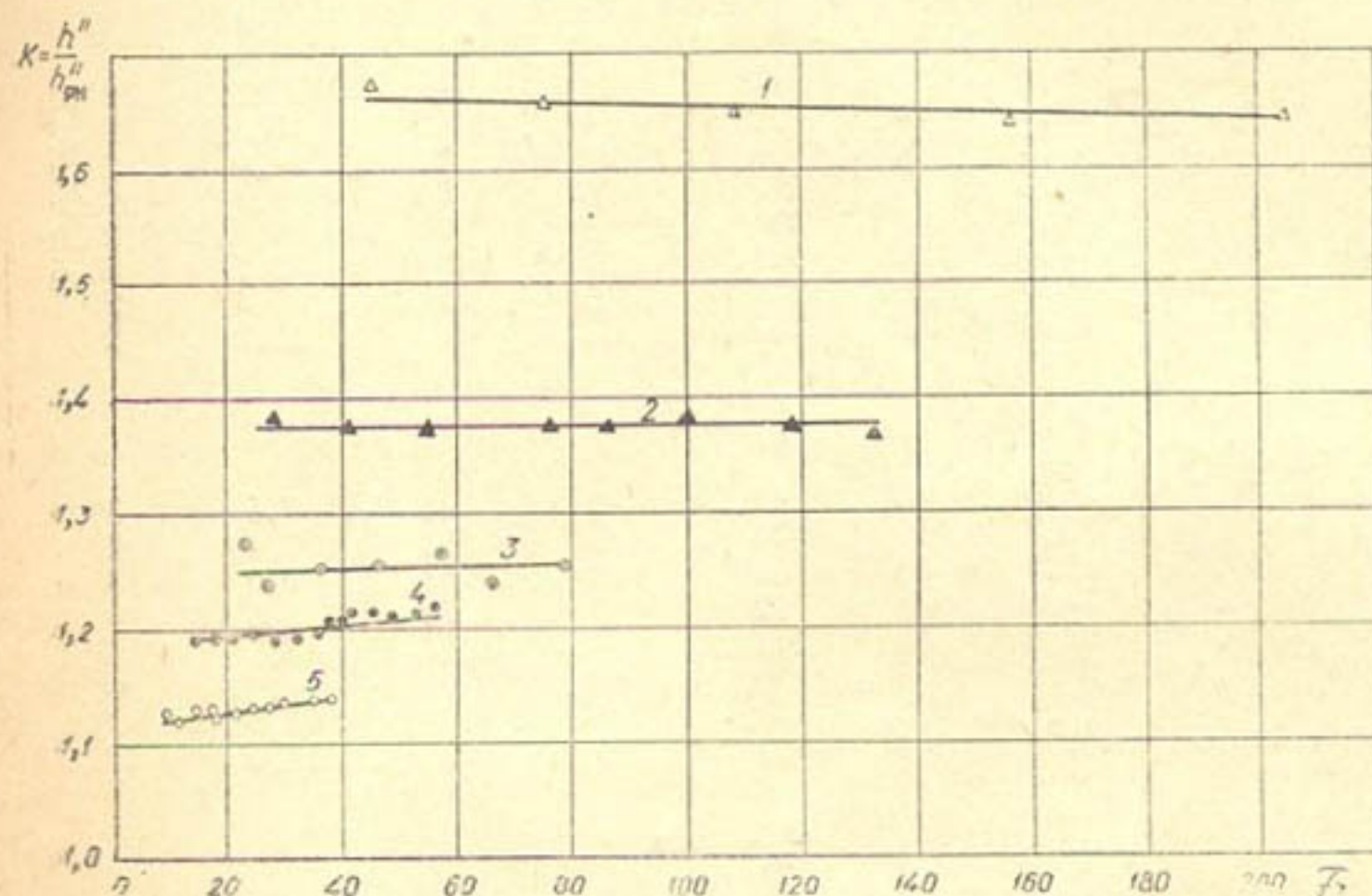
Рис. 3. Зависимость уменьшения сопряженной глубины гидравлического прыжка от числа Фруда.
