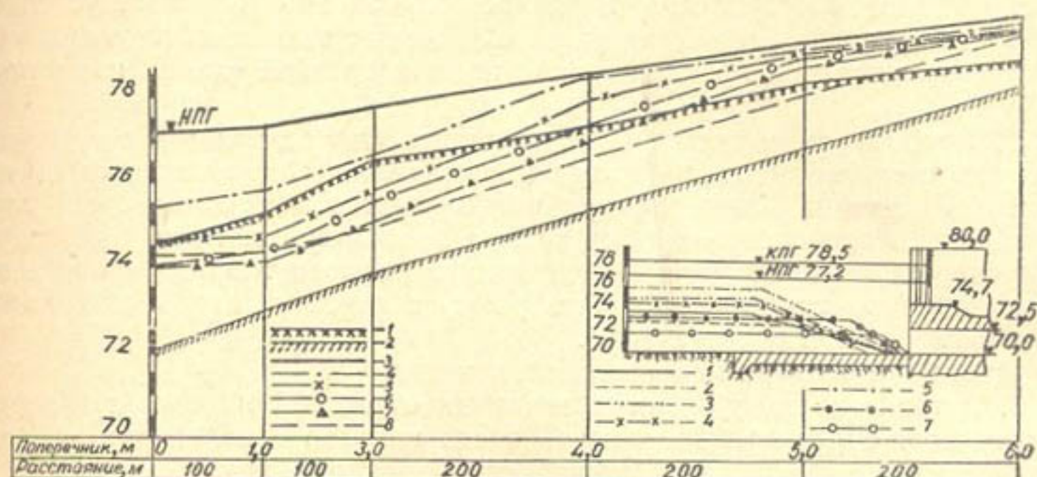
Рис. 4. Продольные профили верхнего бьефа во время промыва при Q = 400 \text{ м}^3/\text{сек} .
