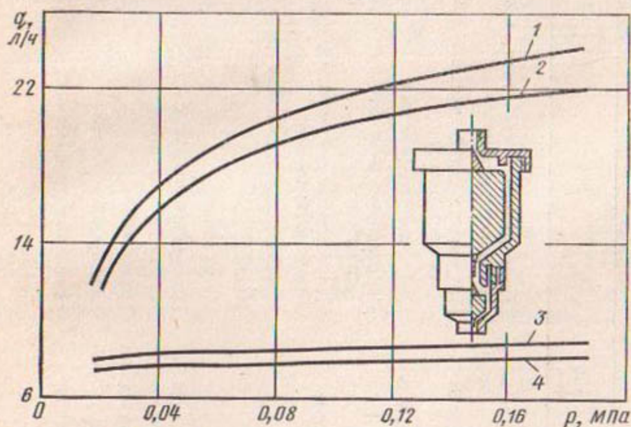
Рис. 13.6. Зависимость расхода от давления и транзитного расхода для капельниц: «ВНИИводполимер» — 1, 2 — Q_T = 0,025 л/с; 0,06; «Узгипроводхоз-2»: 3, 4 — Q_T = 0,025 л/с; 0,06.
