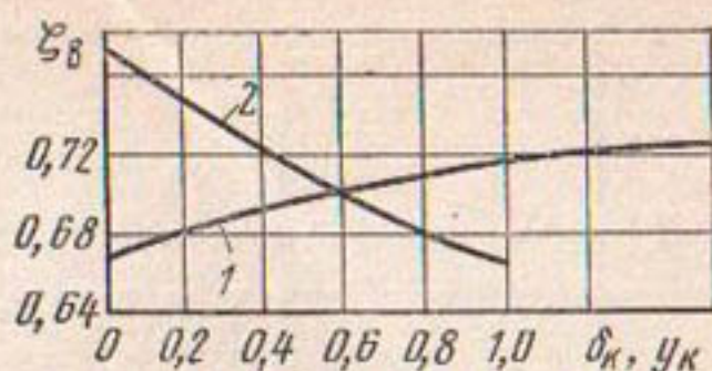
Рис. 8.4. Зависимость \zeta_b от y_{\text{кр}} и \delta_{\text{кр}} : 1 — \zeta_b = f_1(y_{\text{кр}}) ; 2 — \zeta_b = f_2(\delta_{\text{кр}}) .
