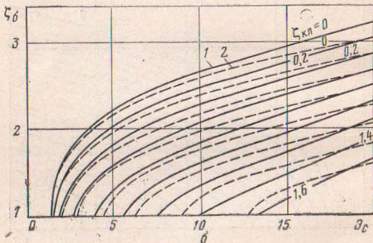
Рис. 8.8. Зависимость \zeta_\delta от \alpha и \zeta_{\kappa\lambda} для призматических русл трапецидального сечения: а— y_k = 0,05 и 0,1 ; б— y_k = 0,15 и 0,25 (кривые даны через 0,2 ).
