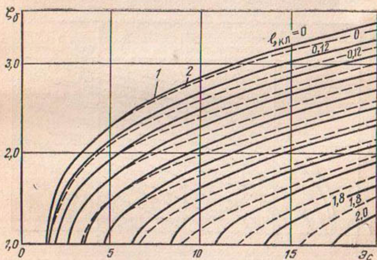
Рис. 8.7. Зависимость \zeta_{\delta} от E_c и \zeta_{кл} призматических русл прямоугольного и трапецидального сечений: 1— y_k=0 ; 2— y_k=0,025 (кривые даны через 0,2).
