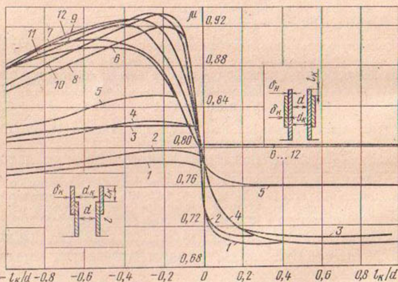
Рис. 5.14. Зависимость \mu от l_K/d для внутренних цилиндрических насадков при истечении в атмосферу: 1...12— d_K/d=1,022 ; 1,028; 1,022; 1,028; 1,062; 1,138; 1,2; 1,38; 1,164; 1,296; 1,148; 1,18; \delta_K/d_K=0,02 ; 0,022; 0,15; 0,098; 0,11; 0,099; 0,11; 0,12; 0,1; 0,15; 0,106; 0,108; \delta_H/d=0,066 ; 0,0045; 0,006; 0,0045; 0,028; 0,065; 0,099; 0,184; 0,077; 0,145; 0,082; 0,094.
