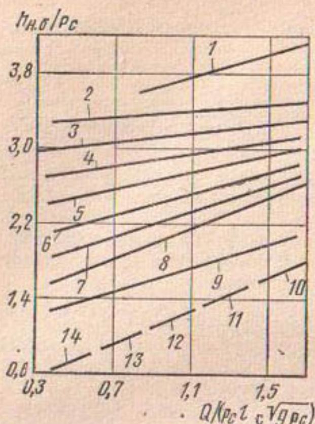
Рис. 9.7. Зависимость h_{н.6}/l от Q/(l_c l_{вс} \sqrt{g l_c}) : 1...14 — h_{вых}/h_{н.6} = 1,02; 1,03; 1,04; 1,05; 1,06; 1,07; 1,08; 1,09; 1,1; 1,3; 1,4; 1,5; 1,6; 1,7 .
