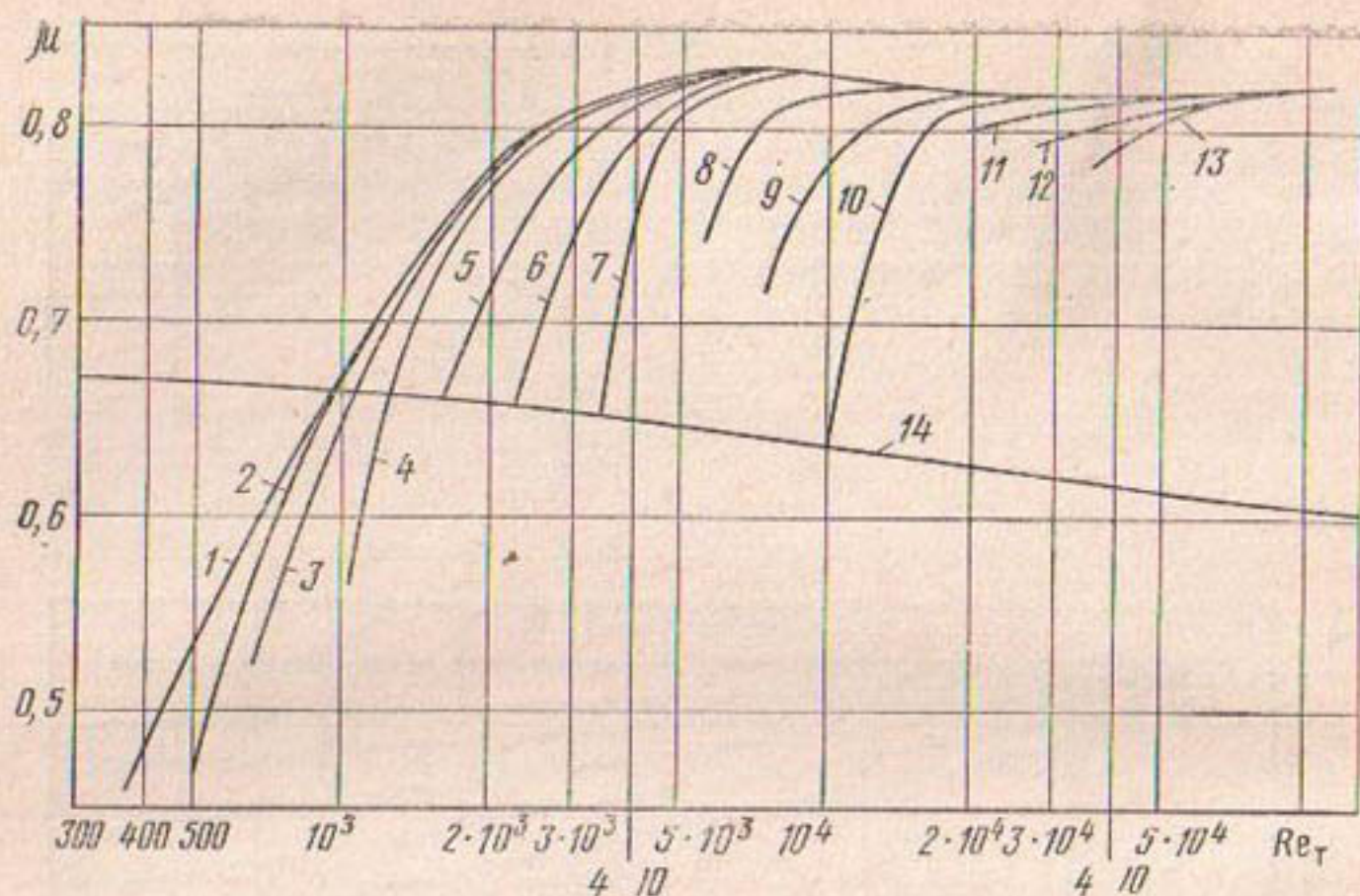
Рис. 5.27. Зависимость \mu от d , H_{\text{ж}} , \text{Re}_{\tau} при n_v=1 ; f=40 Гц: d — 1...4—0,3 мм; 5...7—1; 8...10—4; 11...13—10; H_{\text{ж}} —2, 5, 8, 11 — 100 мм; 3, 6, 9, 12—200; 4, 7, 10, 13—400; 1— n_v=0 .
