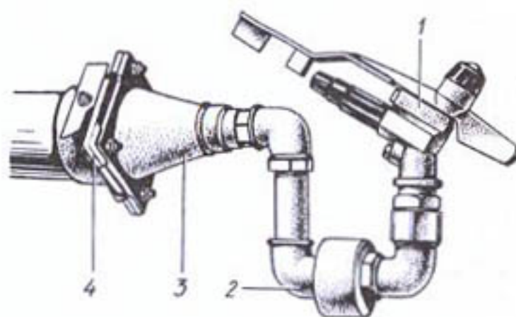
Рис. 3.15. Механизм самоустановки концевой дождевальной машины ДКН-80:
