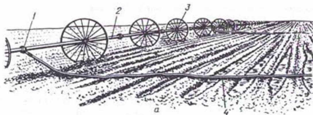
Рис. 2.13. Поливной трубопровод ТКП-90: a — общий вид; 1 — муфта; 2 — водопроводящий пояс; 3 — опорное колесо; 4 — гибкий поливной шлейф; б — муфта со шлейфом для полива по бороздам; 1 — муфта; 2 — диафрагма; 3 — гибкий шланг; 4 — водовыпускные отверстия (20 шт.); 5 — заглушка-зажим для промывки шлейфа
