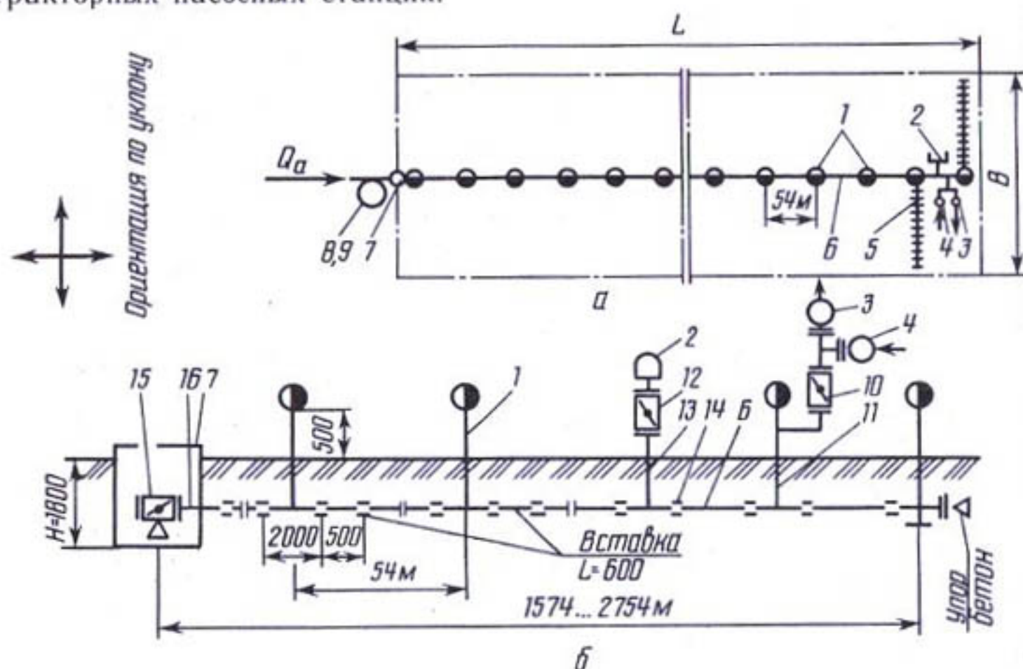
Рис. 3.21. Схема поливного модуля с машиной ДФ-120 «Днепр» (а) и его монтажа (б) (подвод воды к торцу участка, условные обозначения см. табл. 3.33)
