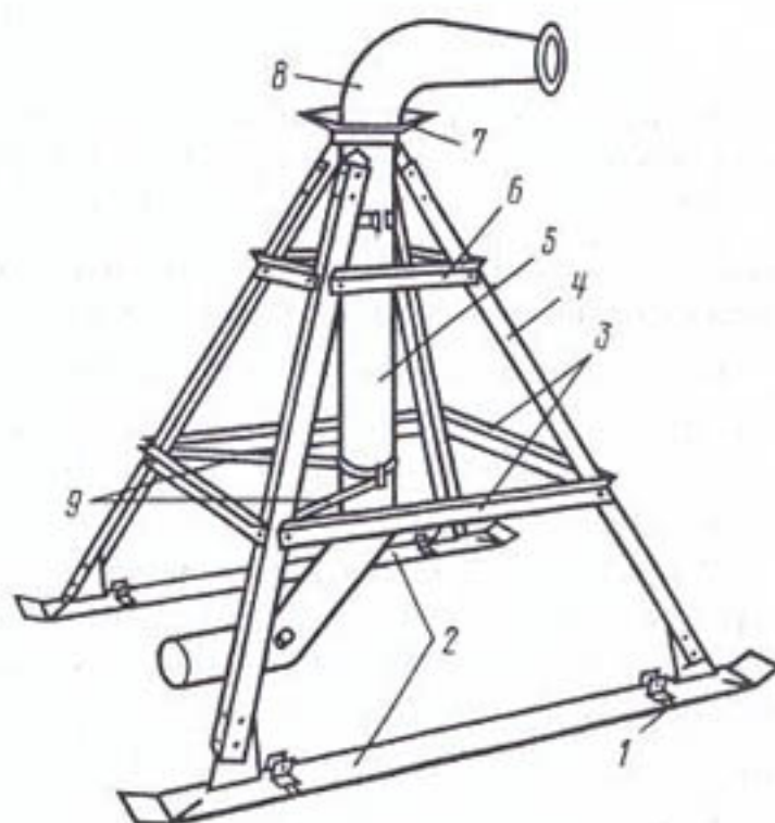
Рис. 3.34. Центральная неподвижная опора машины «Фрегат»:
