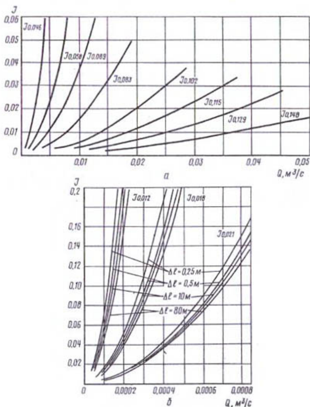
Рис. 4.5. Графики для определения удельных потерь давления в трубопроводах:
