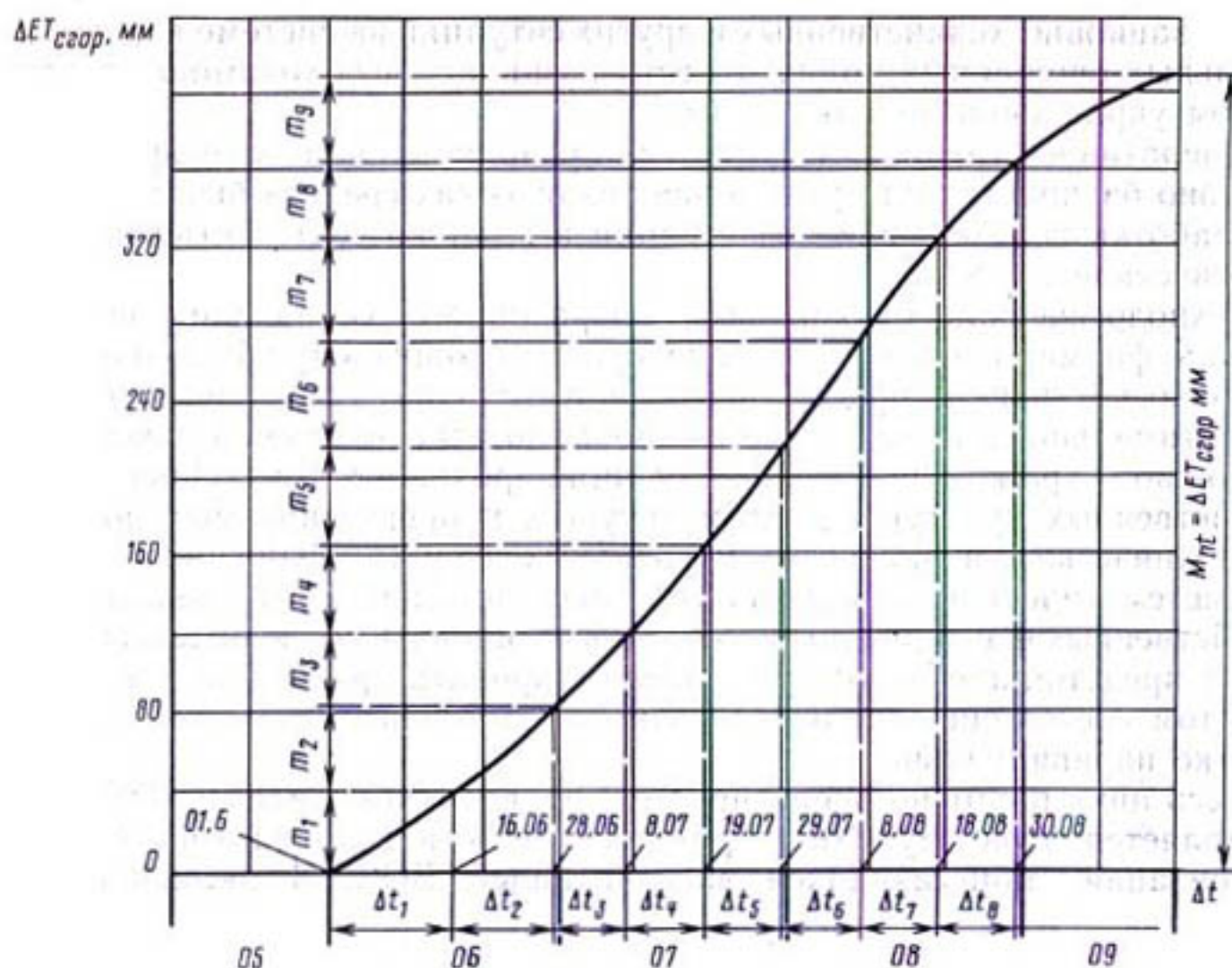
Рис. 1.25. Графоаналитический расчет поливного режима по интегральной кривой дефицита водопотребления: m — поливная норма; \Delta ET_{crop} — дефицит водопотребления; M_{нт} — оросительная норма, нетто; \Delta t — межполивной период, 16.06... 30.08 — средние даты поливов
