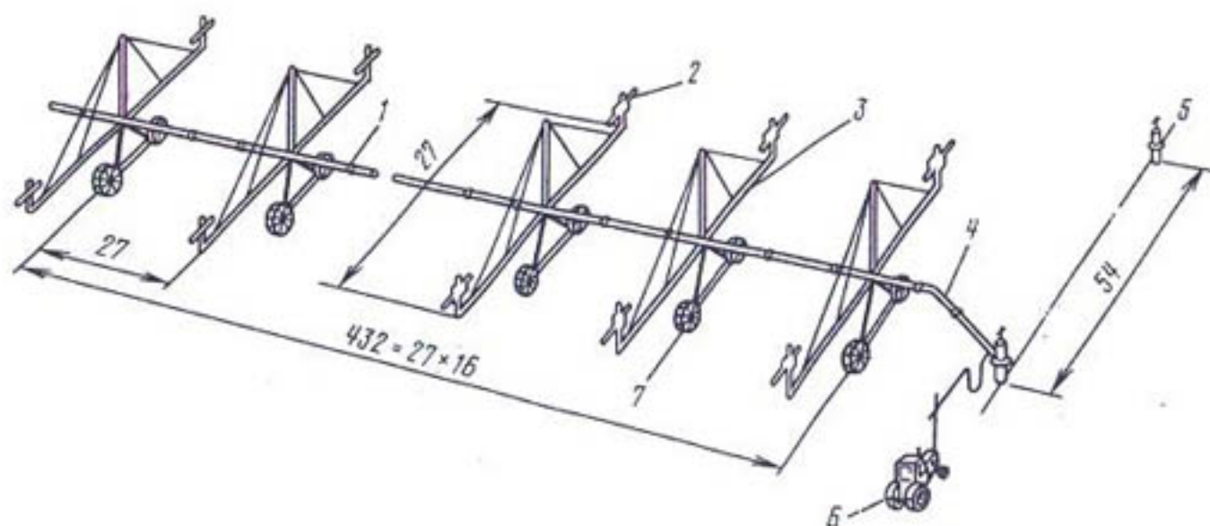
Рис. 3.19. Общий вид дождевальной машины «Днепр» ДФ-120: 1 — водопроводящий пояс; 2 — дождевальная машина «Роса-3»; 3 — открывок; 4 — соединительное устройство; 5 — гидрант; 6 — навесная тракторная электростанция; 7 — самоходная тележка (размеры в м)
