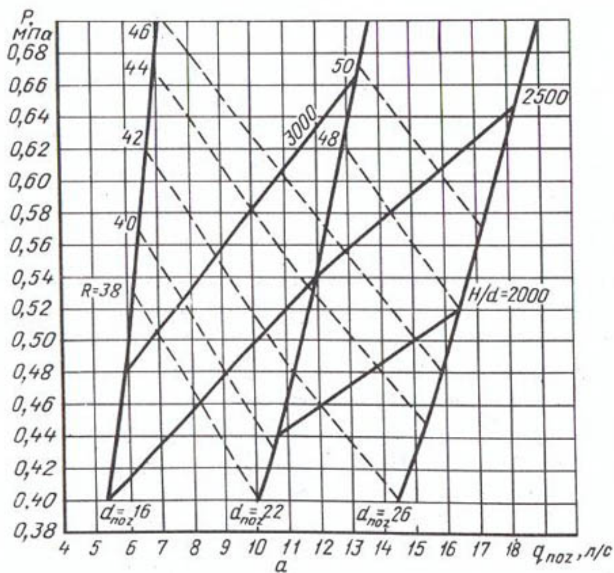
Рис. 3.5. Дальнейструйные дождевальные аппараты и их расходно-напорные характеристики: а — аппарат ДД-15: 1 — турбинка; 2 — сопло; 3 — ствол; 4 — механизм вращения; 5 — присоединительное устройство;
