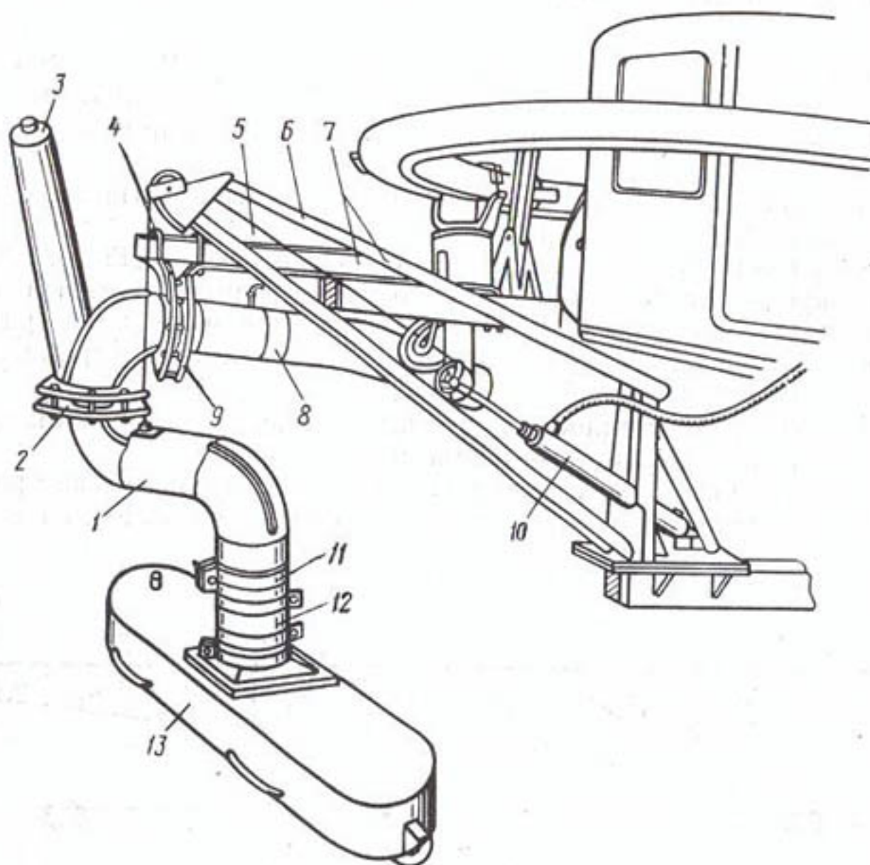
Рис. 3.49. Всасывающая линия:
