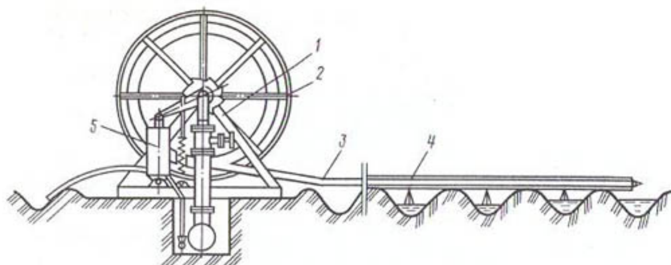
Рис. 2.15. Схема шлангового поливного устройства АШУ-32: 1 — рама; 2 — барабан; 3 — шланг поливной; 4 — водовыпускные отверстия; 5 — гидроцилиндр
