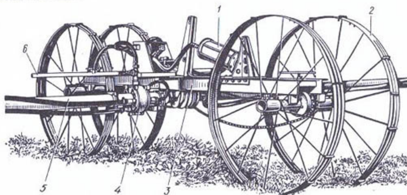
Рис. 3.10. Центральная тележка колесного трубопровода ДКГ-80 «Ока» с гидроприводом:
