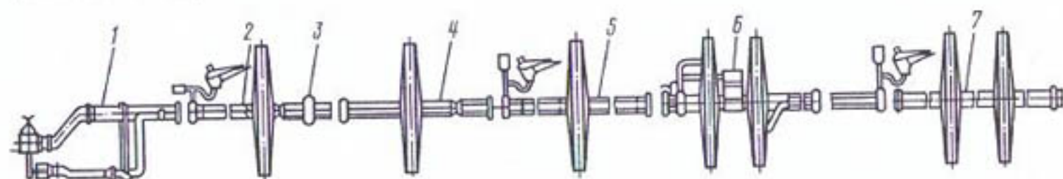
Рис. 3.9. Схема компоновки дождевального крыла машины ДКГ-80 «Ока»:
