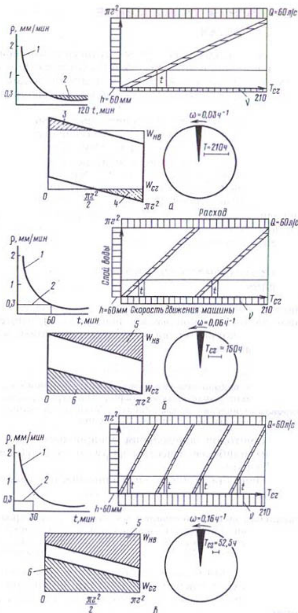
Рис. 1.19. Влияние технологий механизированного полива на параметры эксплуатационного режима орошения на примере использования дождевальную машины кругового действия ДМУ-Б463-60 при поливной норме 600 \text{ м}^3/\text{га} :
