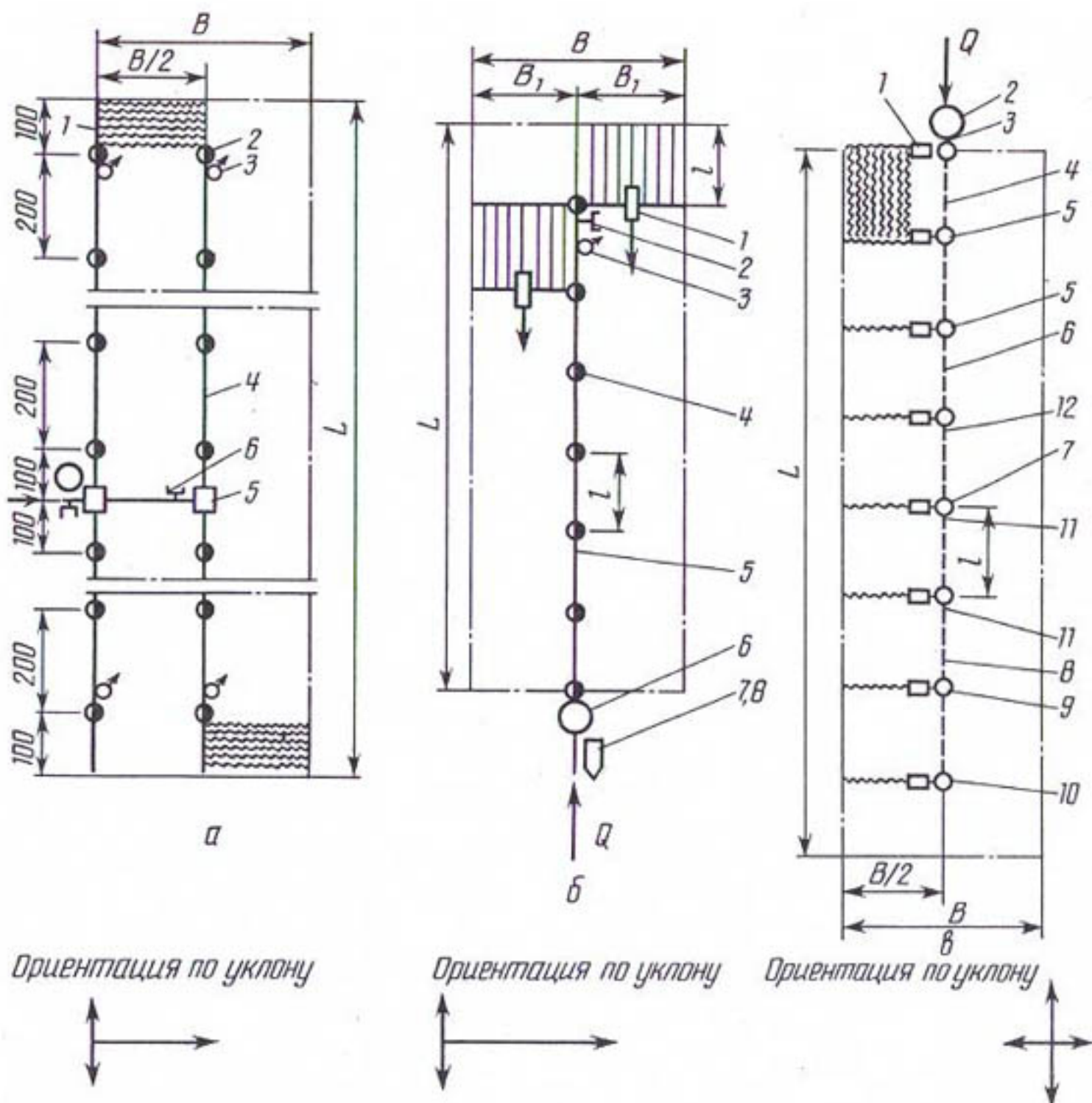
Рис. 2.17. Схема модульного участка с поливом: а — АПС-1 (обозначения см. табл. 2.13); б — ТКП-90 (обозначения см. табл. 2.14); в — АШУ-32 (обозначения см. табл. 2.15) (размеры в м)
