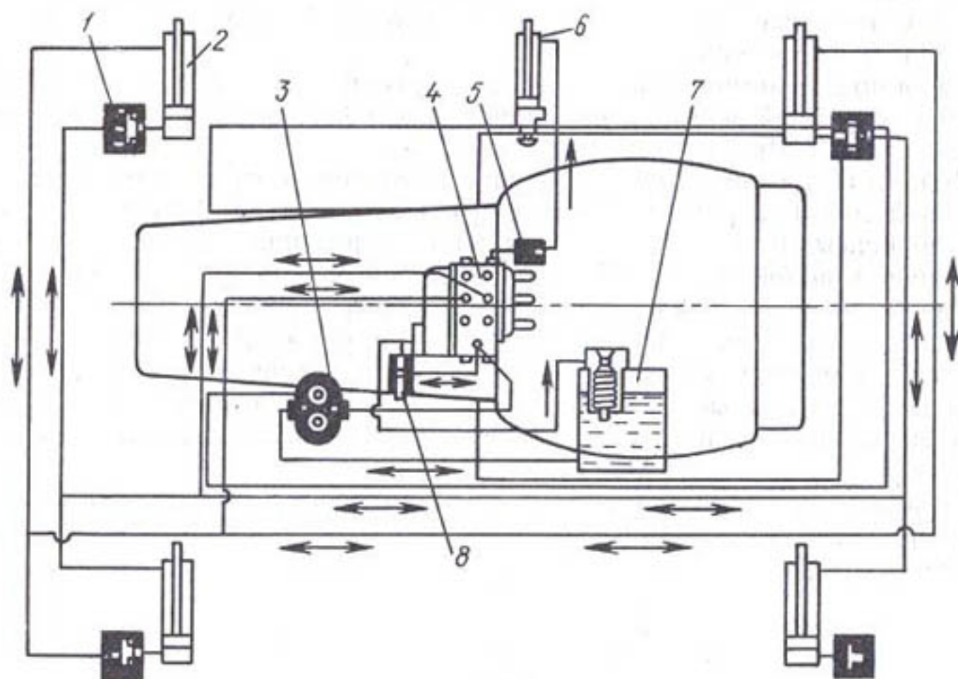
Рис. 3.51. Гидравлическая схема дождевального агрегата ДДА-100МА:
