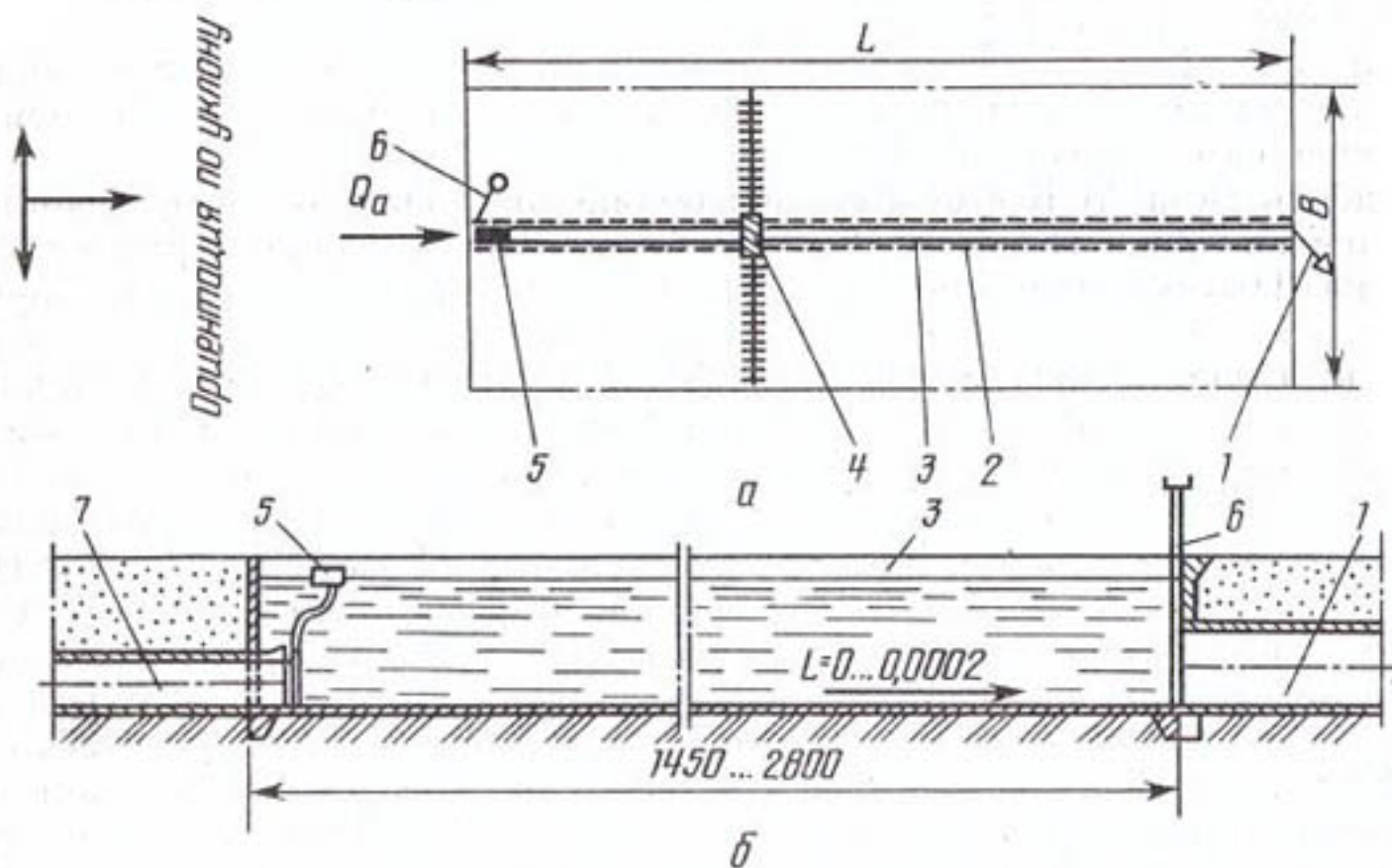
Рис. 3.46. Схема модульного участка с использованием машины «Кубань-Л» (а) и его монтажа (б) (условные обозначения см. табл. 3.59)
