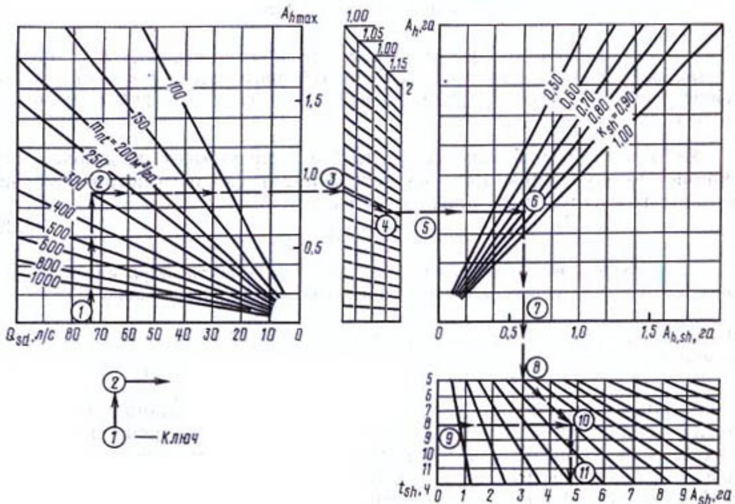
Рис. 3.56. Номограмма для определения сменной выработки дождевальных машин и установок:
