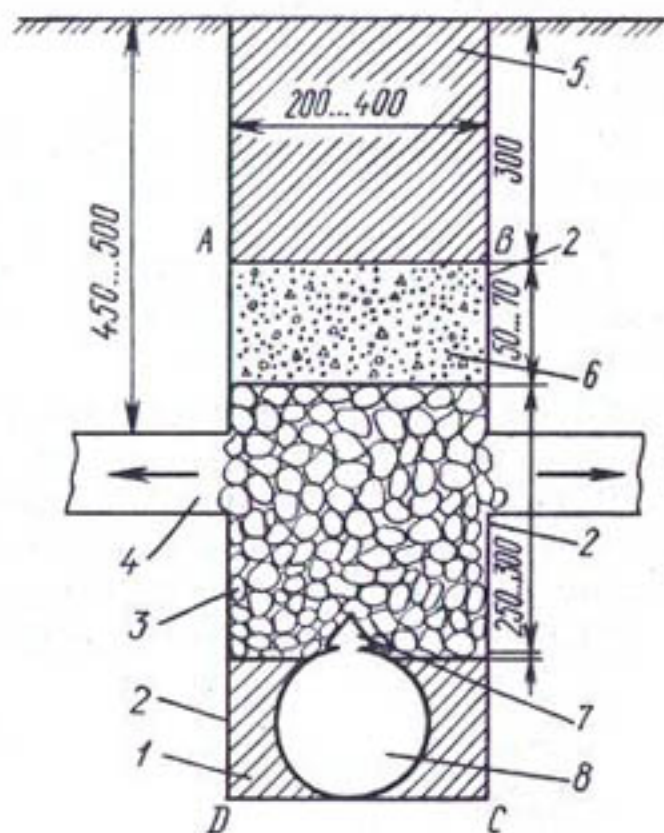
Рис. 4.16. Поперечный разрез траншеи оросительного трубопровода с пористой засыпкой:
