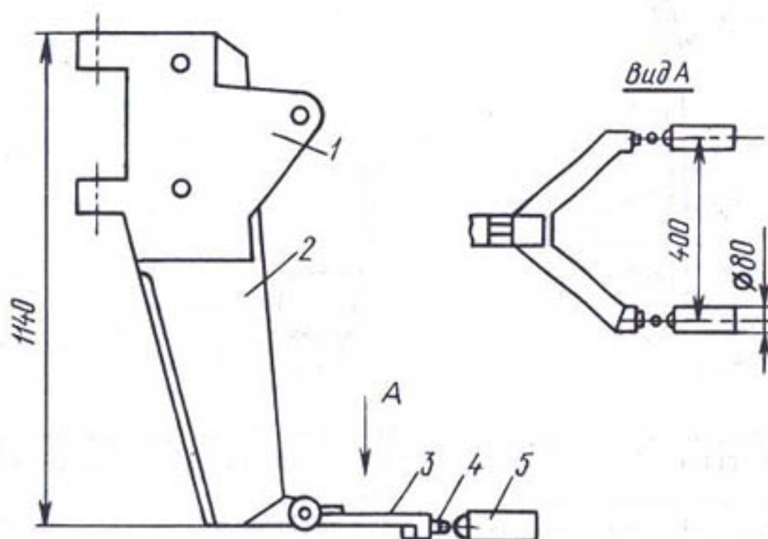
Рис. 4.17. Схема рабочего органа кротователя КТД-0,45 для нарезки кротовых увлажнителей в грунтах при влажности не менее 21...30 % от массы сухой почвы: 1 — серга; 2 — нож; 3 — дрениер; 4 — форсунка; 5 — уширитель
