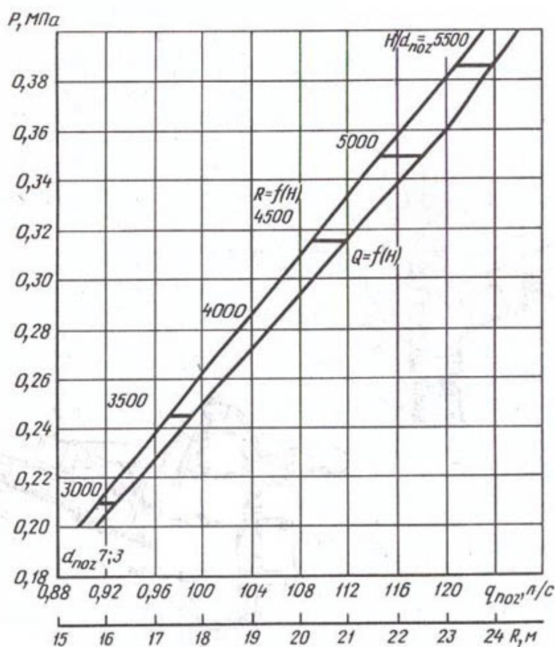
Рис. 3.3. Среднеструйный дождевальнй аппарат ДКШ-64.00.060 и его расходно-напорная характеристика: 1 — пружина возвратная; 2 — коромысло; 3 — сопло; 4 — корпус; 5 — пробка (остальные обозначения см. рис. 3.2)
