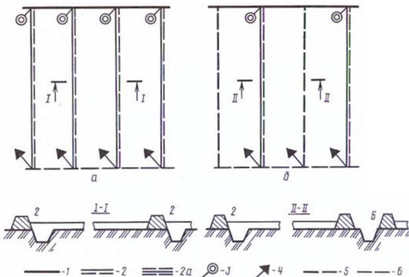
Рис. 2.22. Схема карты-чека:
