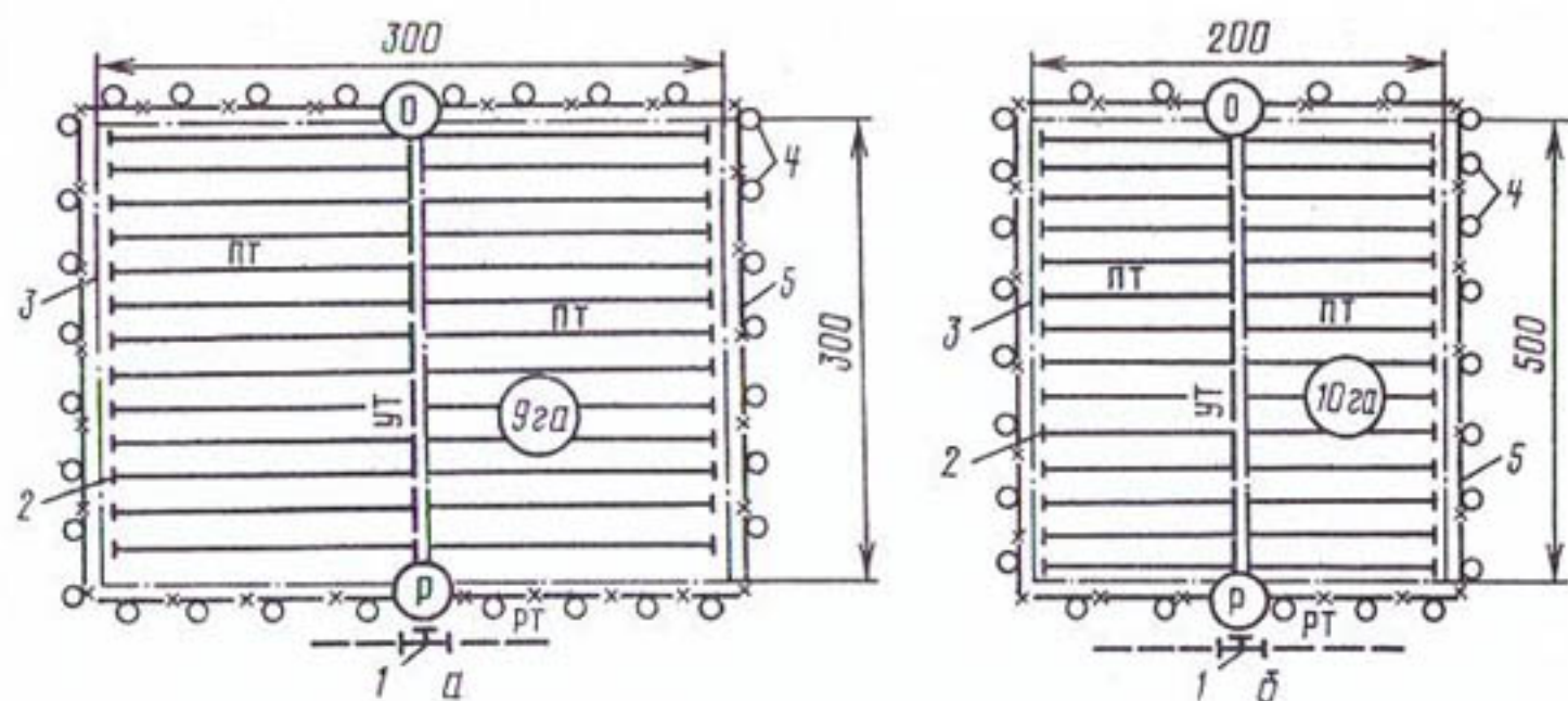
Рис. 4.8. Модульные участки капельного орошения для уклонов не более 0,05: а — сад; б — виноградник; РТ — распределительный трубопровод; УТ — участковый трубопровод; ПТ — поливной трубопровод с микроводовыпусками; Р — распределительный колодец; О — сбросной колодец; 1 — тройник; 2 — концевая заглушка на поливном трубопроводе; 3 — дорога; 4 — лесополоса; 5 — граница модульного участка
