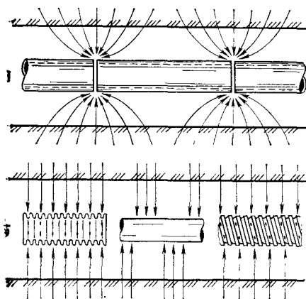
Рис. 5.8. Поступление воды в дренажную гончарную трубу (А) и трубу из ПВХ (Б).
