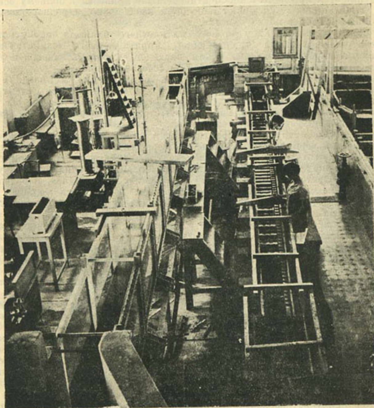
Рис. 16. Гидротехническая лаборатория. Производство замеров при испытании Вахшского быстрогока
