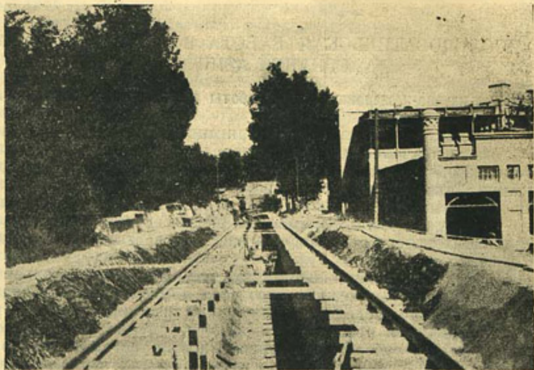
Рис. 13. Тарировочная станция. Общий вид тарировочного бассейна
