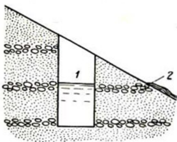
Рис. 8-4. Исследование фильтрационных ходов в теле сооружаемой земляной плотины. 1 — шурф; 2 — ключ.
