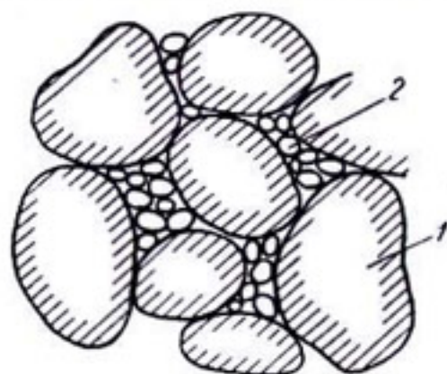
Рис. 7-5. Схема структуры грунта.
