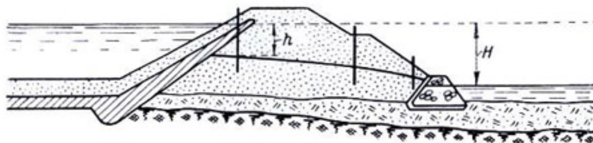
Рис. 3-10. Пьезометрический створ в земляной плотине с экраном.
