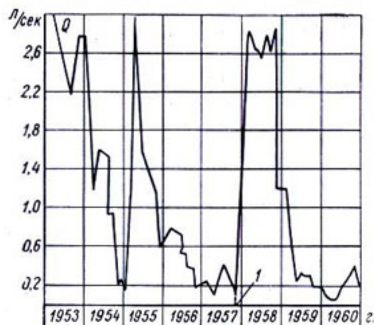
Рис. 8-15. График дебита скважины. I — момент смены фильтра.
