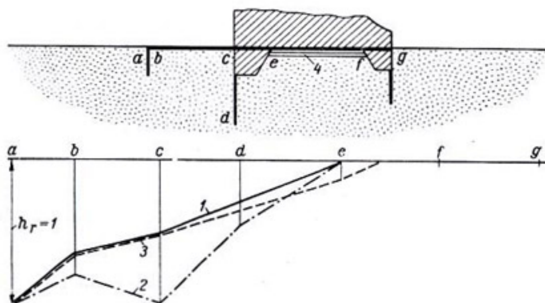
Рис. 8-21. Схема флотбета с дренажем и эпюры приведенных напоров.
