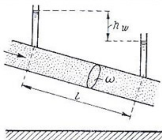
Рис. 2-4. Схема фильтрации в цилиндрической трубе.
