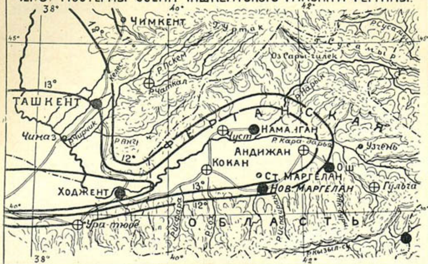
Чер.3. ИЗОТЕРМЫ ОСЕНИ ТАШКЕНТСКОГО РАЙОНА И ФЕРГАНЫ.
