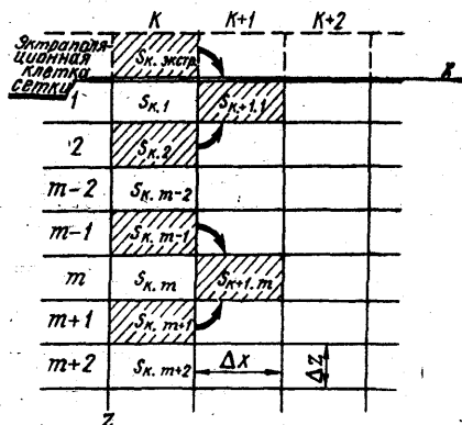
Рис. 7.9. Сетка к расчету турбулентной диффузии (плоская задача).
