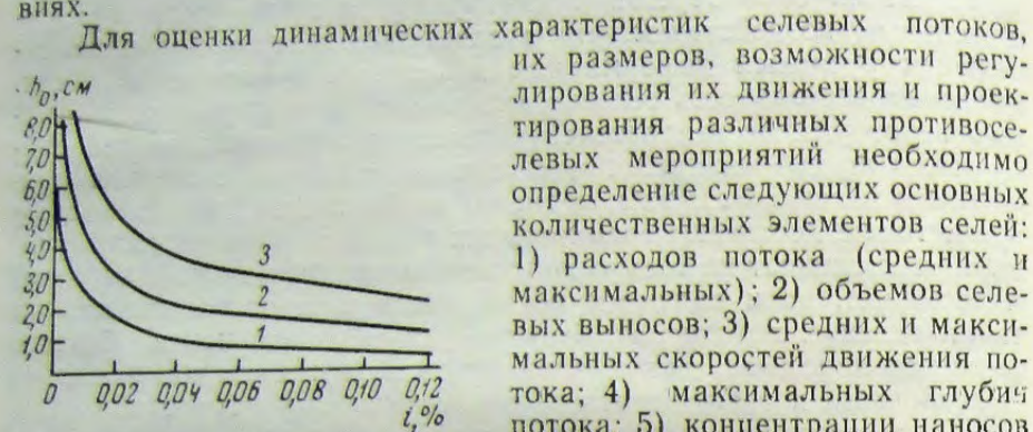
Рис. 35. Зависимость непередвигающегося слоя потока от уклона русла и вязкости селевой массы при h_0 = f(i, \eta) :
