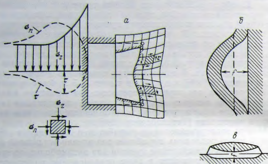
Рис. 30. Отслаивание льда в стенках туннеля в леднике: а — линии деформации; б — чашеобразный выступ; в — горизонтальное сечение через чашеобразный выступ ( f = 5-10 см)
