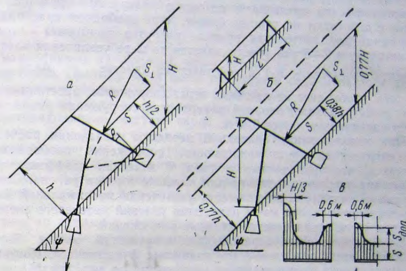
Рис. 27. Расчетная схема давления снега на удерживающие сооружения:
