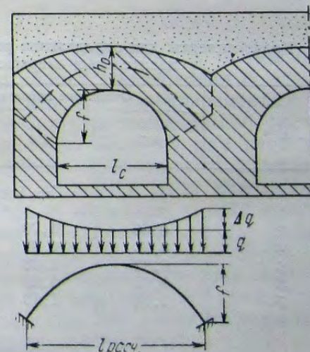
Рис. 11. Расчетная схема ледяного сводчатого перекрытия при l_c = l_{расч} - \frac{4h_0 f}{l_{расч}}
