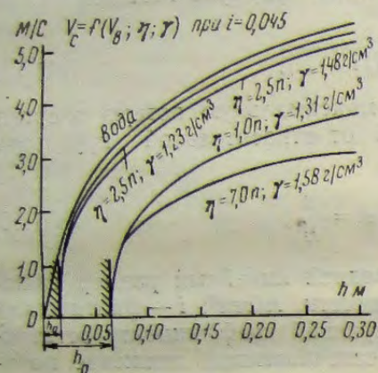
Рис. 36. Кривые зависимости скорости движения связанного селея от его структурно-механических характеристик и глубины потока при v_c = f(v_n; \eta; \gamma); i = 0,045
