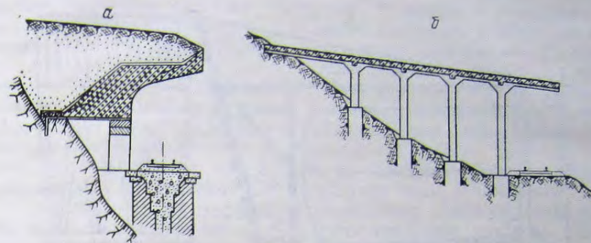
Рис. 24. Противолавинные железобетонные навесы: а — на Реттской ж. д. (Швейцария); б — на Офотенской ж. д. (Норвегия)
