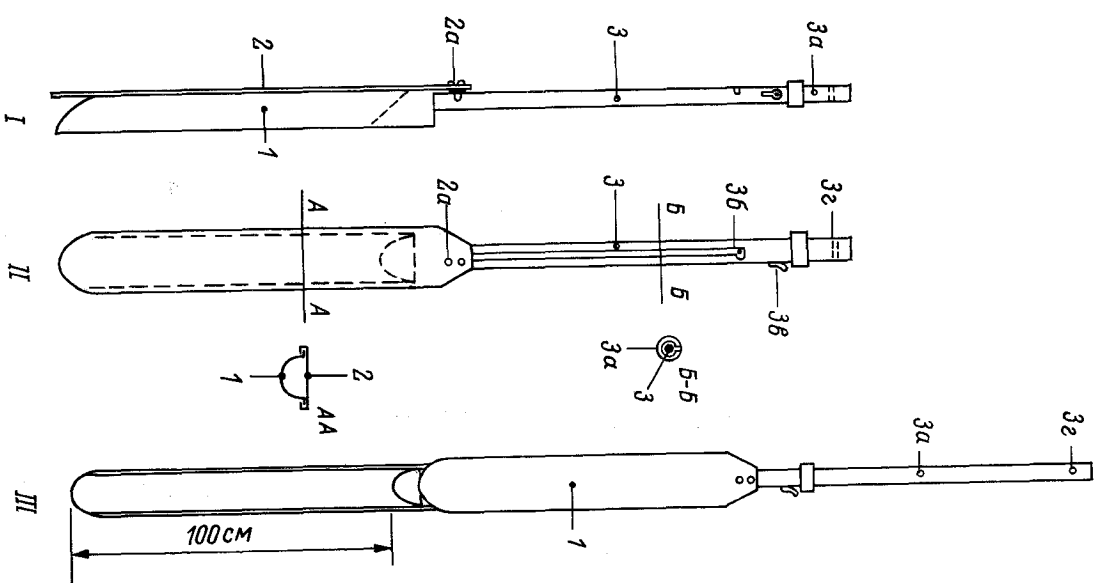
Рис. 7. Унифицированный бур Института торфа. I — вид сбоку; II — бур открыт; III — керна заборная желонка; 2 — крышка желонки; 2a — бур закрыт; 1 — керна заборная желонка; 3 — труба; 3a — крепление крышки к вращающемуся стержню (3a); 3b — кольцо для страховочной веревки; 3c — отверстие для соединения со штангами.
