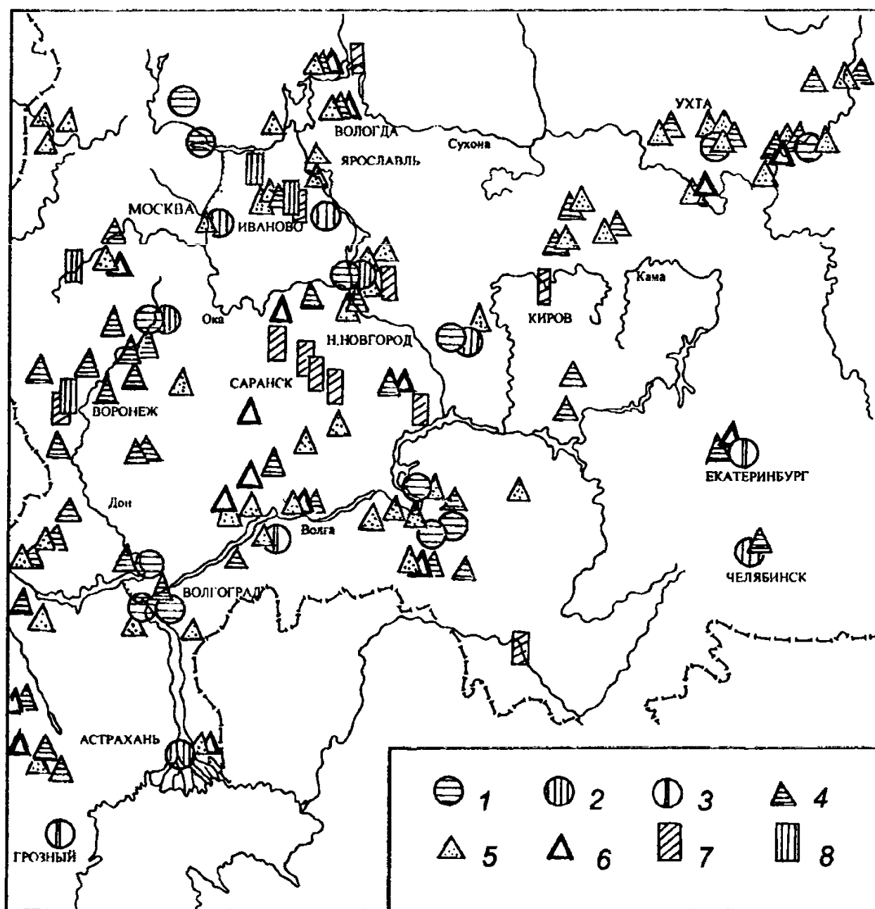
Рис. 5.2.6. Повышенные концентрации
