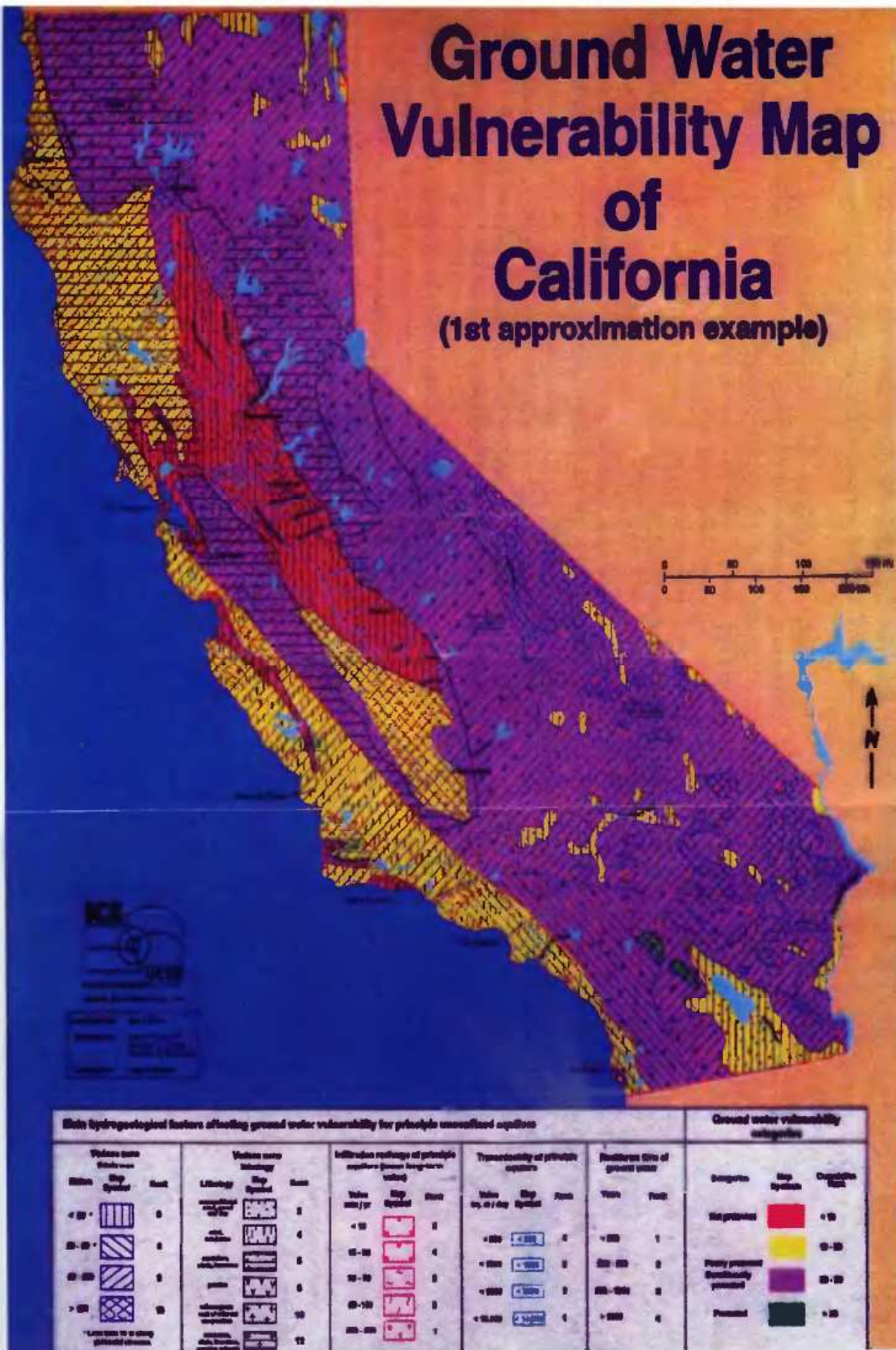
Рис. 6.2.1. Карта защищенности подземных вод от загрязнения штата Калифорния (США)
