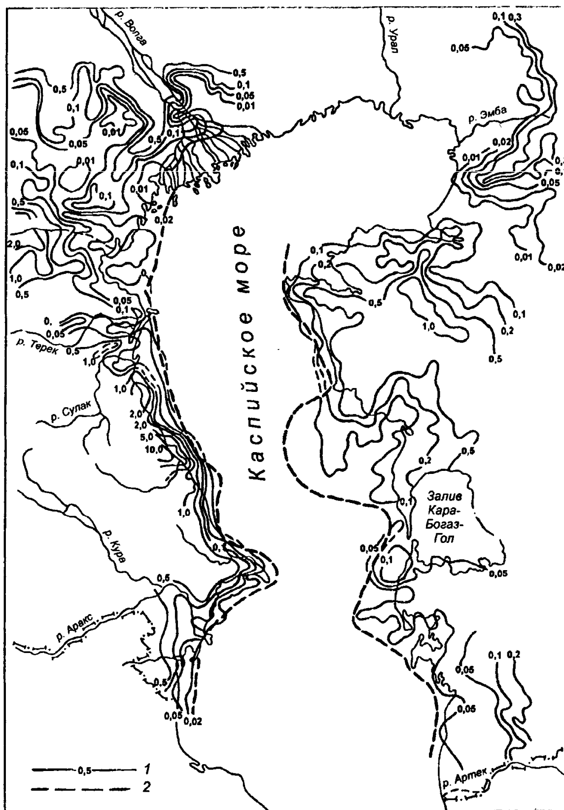
Рис. 4.4.1. Карта вертикальной разгрузки напорных вод
