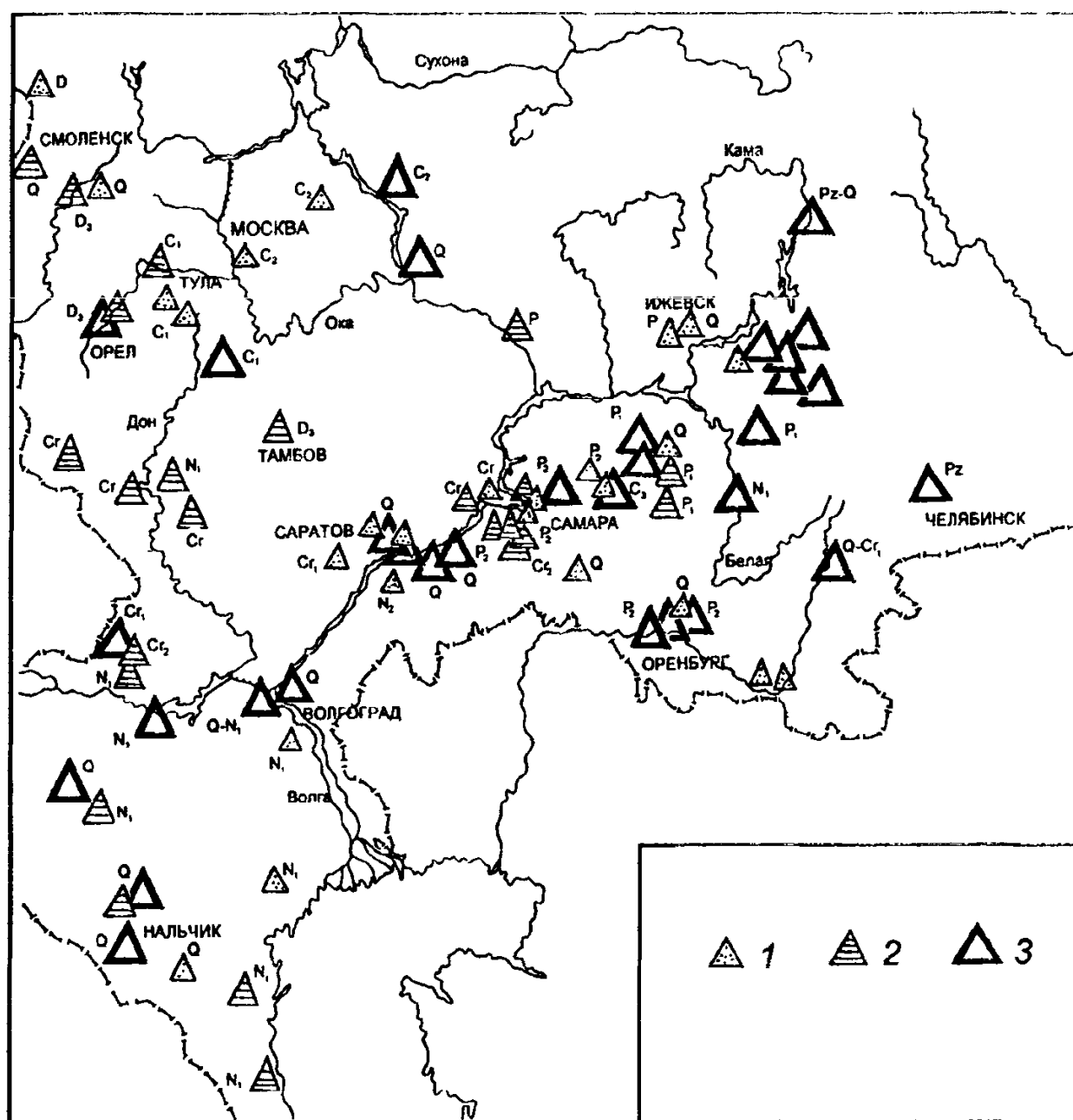
Рис. 5.2.5. Повышенная минерализация
