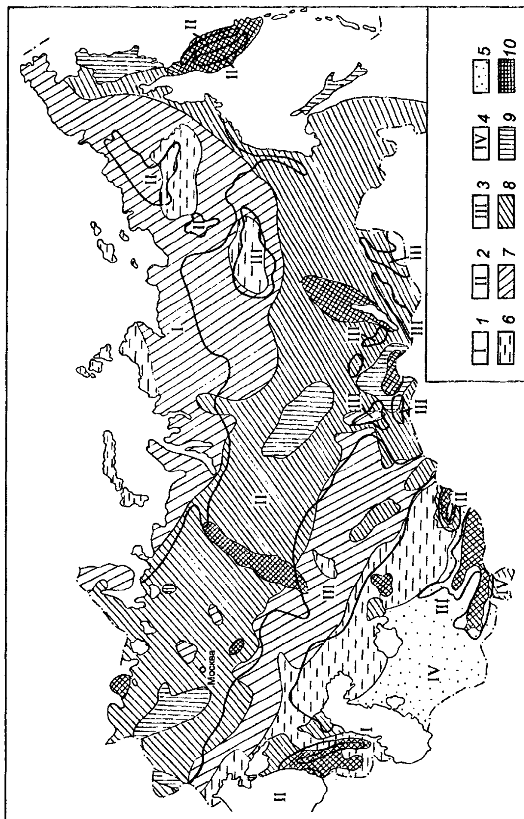
Рис. 2.4.2.1. Схематическая карта связи подземного стока с природно-климатическими зонами. Природно-климатические зоны: 1 – избыточно-влажная; 2 – влажная; 3 – недостаточно-влажная; 4 – сухая. Коэффициент подземного стока, %: 5 – <1, 6 – 1–3, 7 – 3–5, 8 – 5–10, 9 – 10–20, 10 – 20–50
