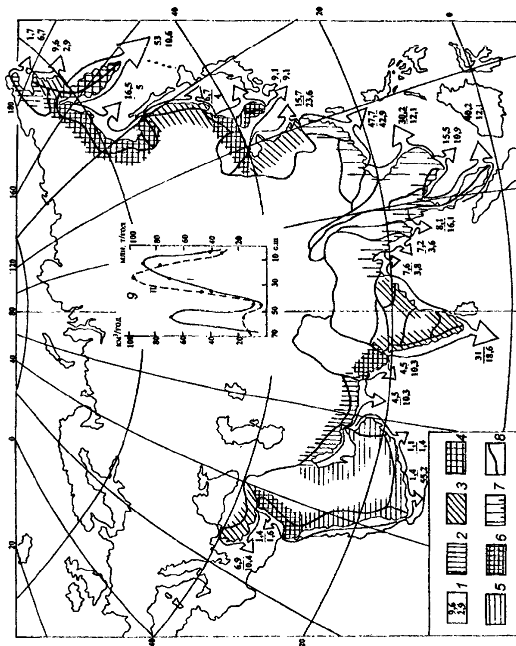
Рис. 4.3.1. Схематическая карта подземного стока в океан с территории Азии
