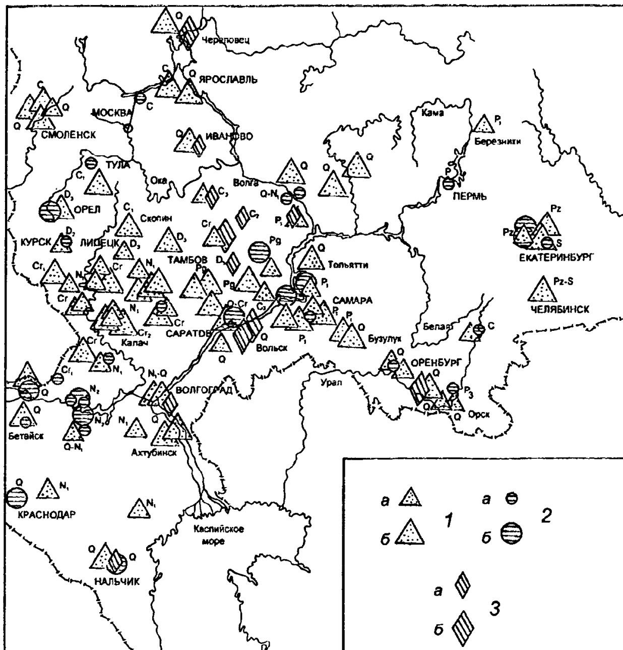
Рис. 5.2.8. Повышенные концентрации
