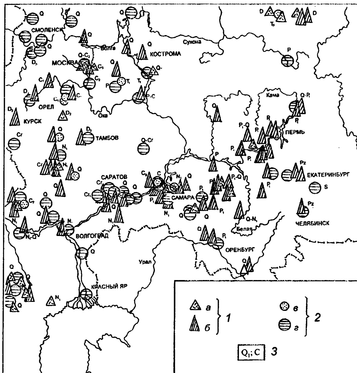
Рис. 5.2.4. Повышенные концентрации
