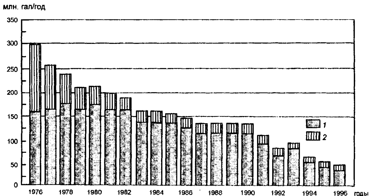
Рис. 2.2.2. Отбор подземных вод в районах проседания на территории Хьюстонского региона (из доклада по подземным водам, ХГССД, 1996)
