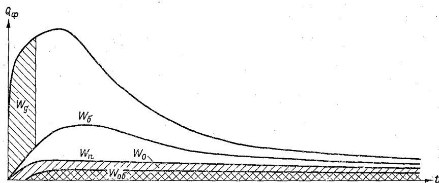
Рис. 3.3. Кривые, характеризующие изменение различных видов фильтрационных потерь из водохранилища во времени [151].
