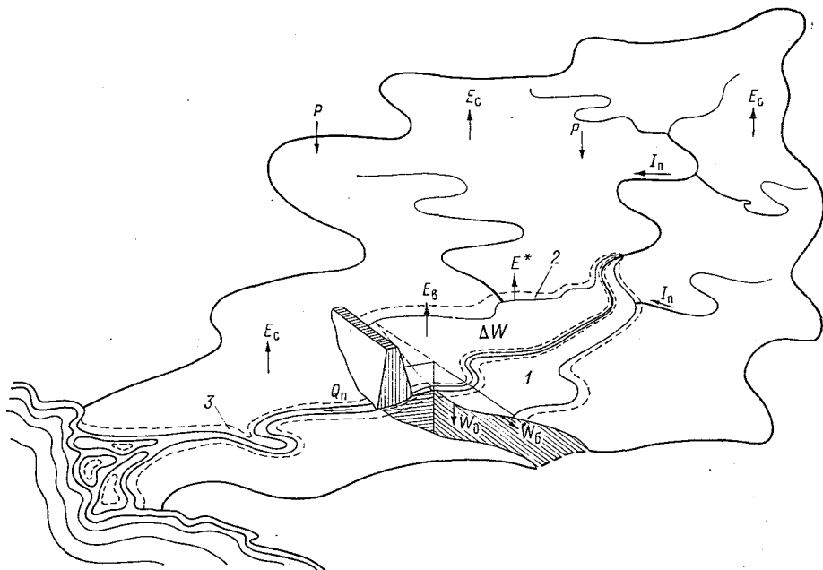
Рис. 2.1. Характерные зоны речного бассейна, в пределах которых изменяются элементы водообмена при создании водохранилища. 1 — зона затопления, 2 — зона подтопления, 3 — приустьевая зона реки ниже створа подпорного сооружения.
