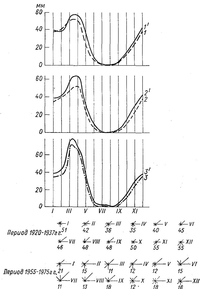
Рис. 2.2. Хронологические графики хода среднемесячных значений осадков по станциям Каттакурган (I—3) и Самарканд (I'—3') и розы ветров по ст. Каттакурган.
