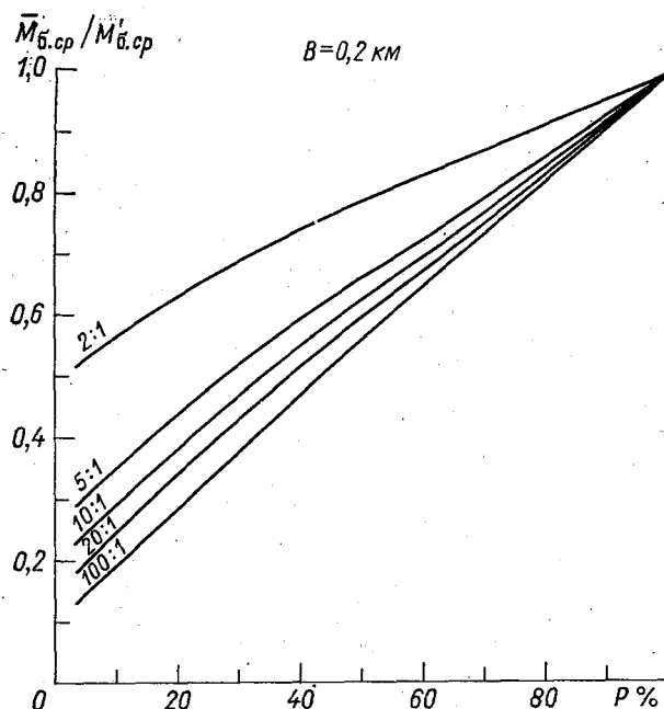
Рис. 4.4. Зависимость среднего значения коэффициента трансформации \bar{M}_{б. ср} от повторяемости ветра P , дующего в направлении длинной оси водоема, и значений M'_{б. ср} при различных соотношениях длины и ширины водохранилища.
