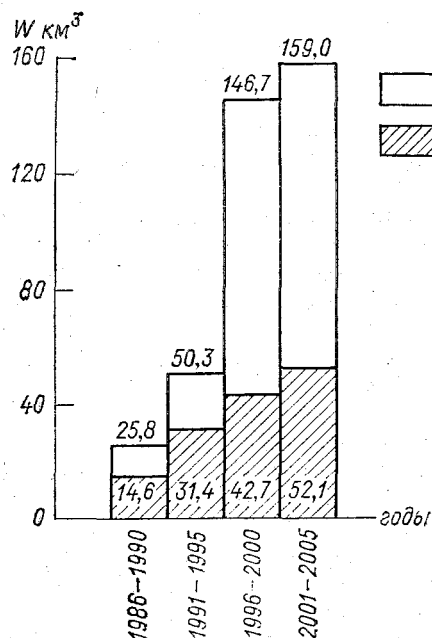
Рис. 7.5. Приращение полного (1) и полезного (2) объемов водохранилищ объемом более 0,1 км³.
