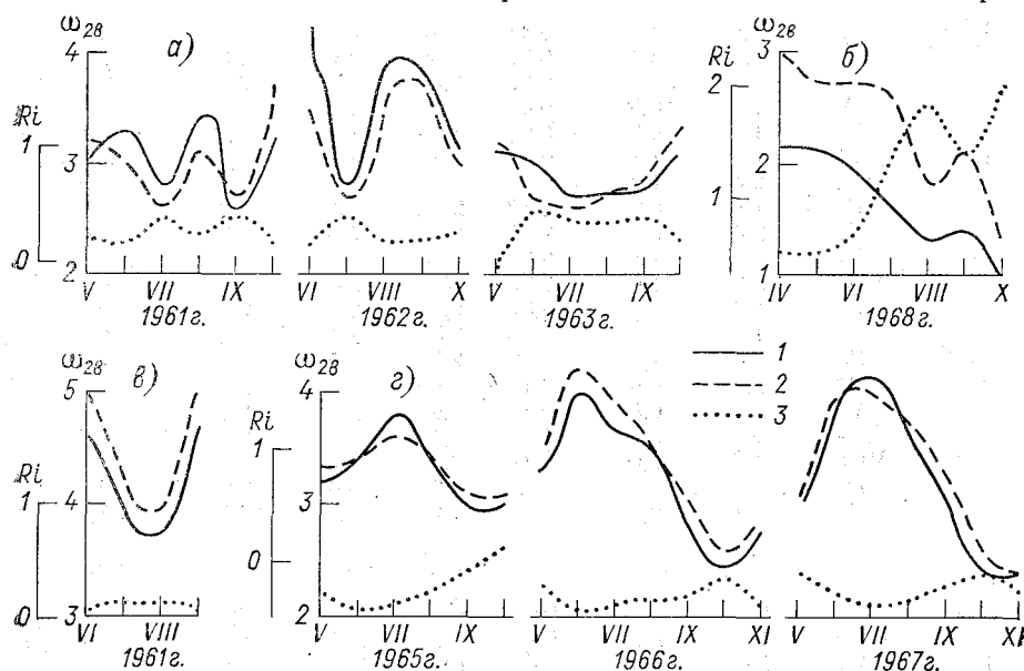
Рис. 4.2. Изменение среднемесячных значений скорости ветра над водной поверхностью \omega_2 и числа Ri .
