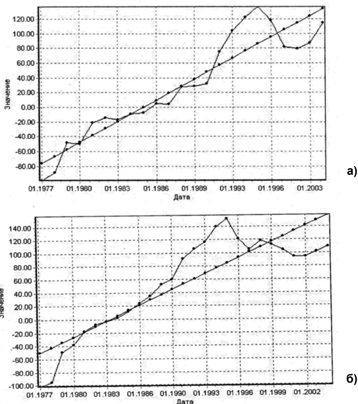
Рис. 3.11. Многолетний ход уровня моря и его тренд на ГМС: о. Тюлений (а); Махачкала (б).
