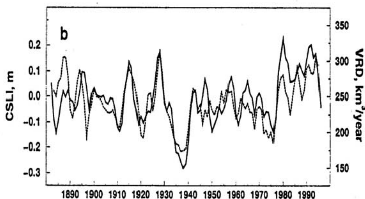
Рис. 8.25. Приращение уровня Каспийского моря за год (левая ось ординат, м) и годовой сток Волги (правая ось ординат, км³/год) [100].
