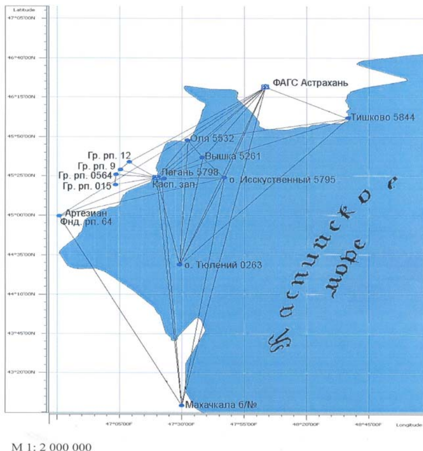
Рис. 3.4. Спутниковая сеть реперов морских уровенных постов на северо-западном побережье Каспийского моря: 5532 – номер пункта, репера; ФАГС Астрахань – пункт спутниковой сети; Гр. рп. – репер уровенной сети.
