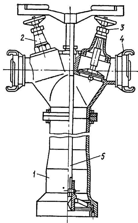
Рис. IV.20. Пожарная колонка
