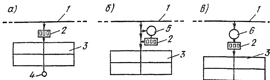
Рис. VIII.2. Схема подключения внутриводной сети к городскому водопроводу
