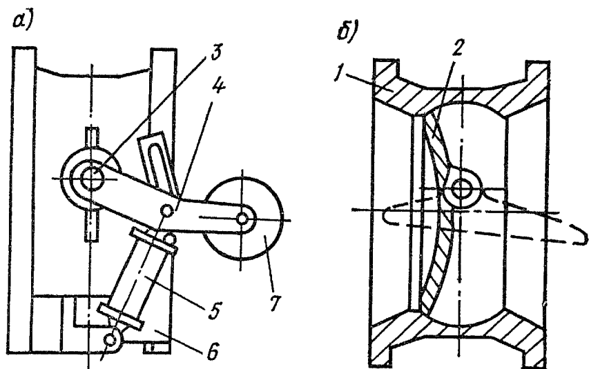
Рис. IV.10. Клапан обратный поворотный с регулируемым закрытием
