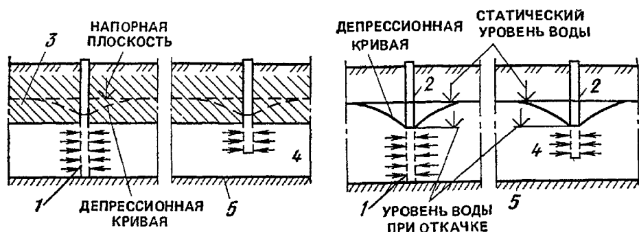
Рис. VII.12. Типы скважин
