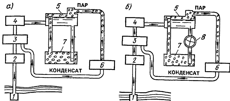
Рис. VIII 31. Система испарительного охлаждения с парообразованием внутри охлаждаемой детали
