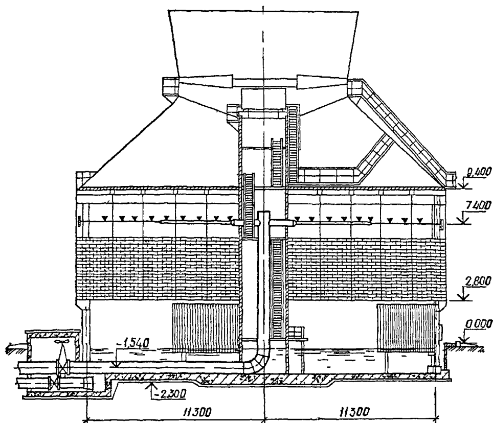
Рис. VIII 27 Одновентиляторная градирня площадью 400 м²
