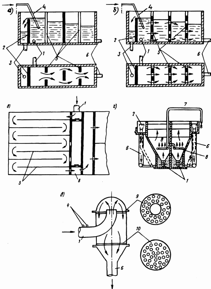
Рис. 5.6. Смесители гидравлического типа с разделением потока (а), дырчатый (б), перегородчатый (в), вихревой (г), напорный дырчатый (д):
