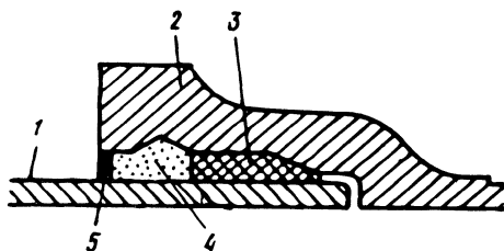
Рис. 3.9. Растровое соединение чугунных труб с уплотнениями пеньковой прядью
