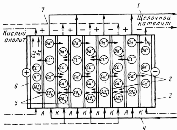
Рис. 5.31. Схема многокамерного электродиализного аппарата: 1, 4 — отвод обессоленной и подача исходной воды; 2, 5 — иононе- селективные катионитовые и анионитовые мембраны; 3 — катод; 6 — анод; 7 — отвод концентрата
