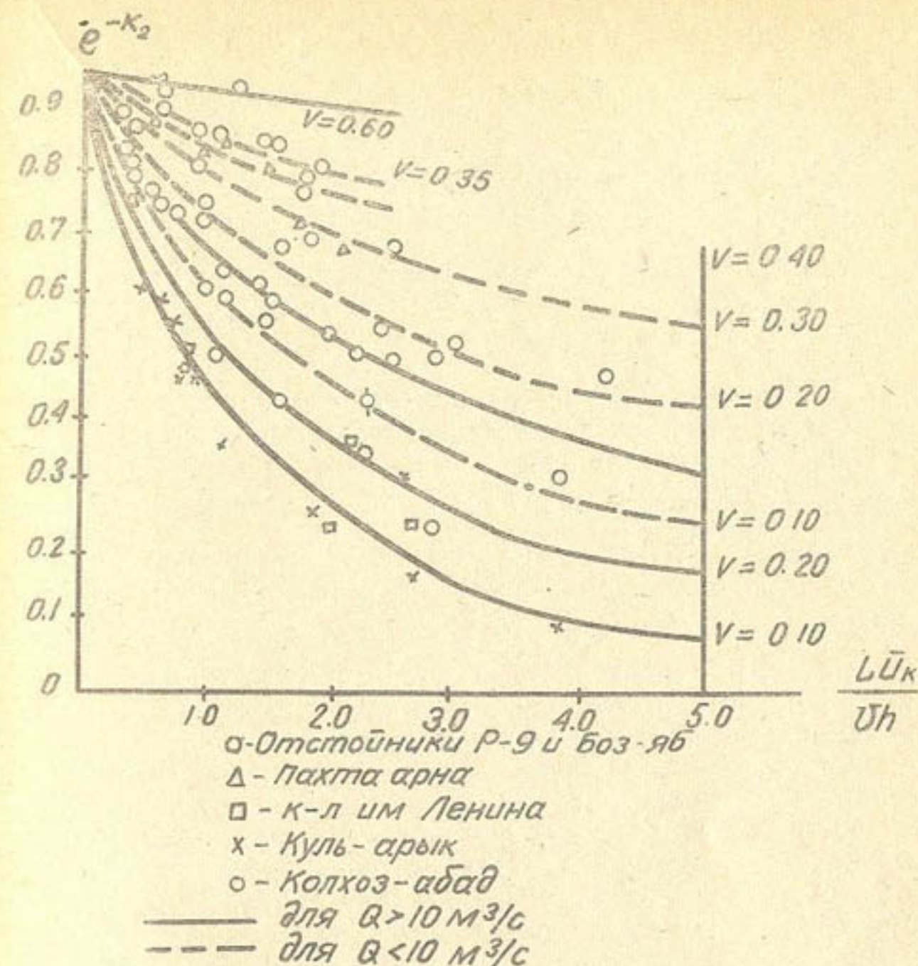
Рис. 17. Зависимость e^{-\kappa_2} = f\left(\frac{lu_k}{vh_{cp}}\right) для фракции наносов (2—0,02) мм/сек.
