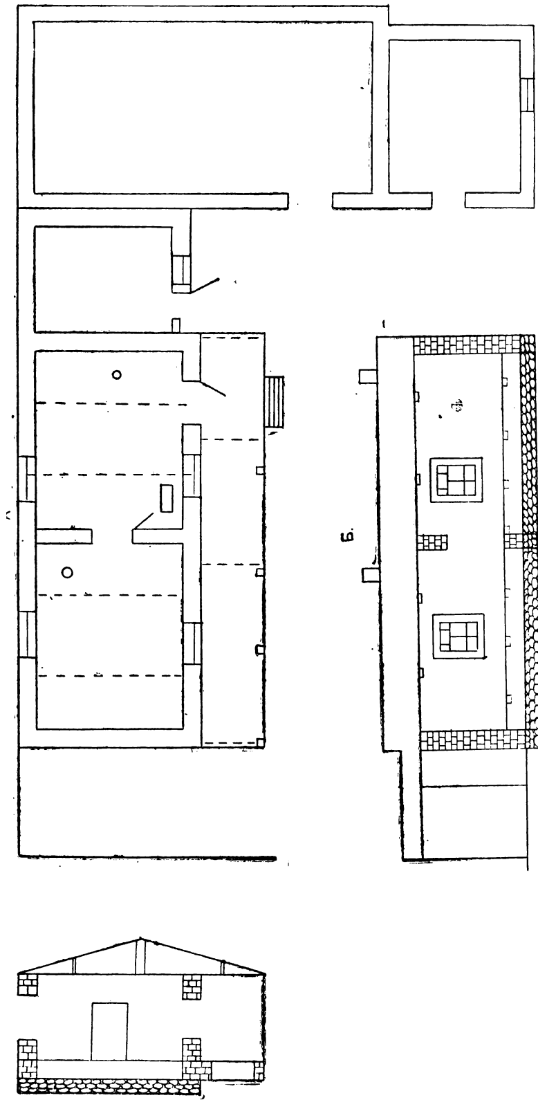
Рис. 34. План жилого дома из сырцового кирпича и с подворными постройками колхозника Шамирбекова. Колхоз им. Сталина, с. Ак-Булун, Ново-Вознесенского района. А—план дома, Б—фасад дома.
