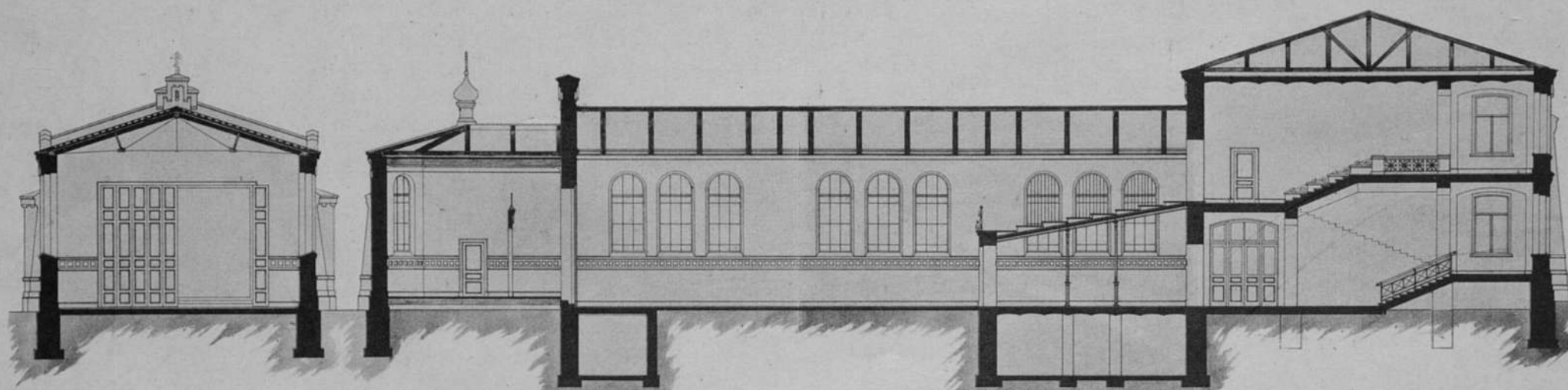
Разрѣзъ по аб. Coupe suiv. ab.
