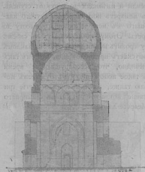
Разрѣзъ купола мечети Медресе-Ханымъ.
