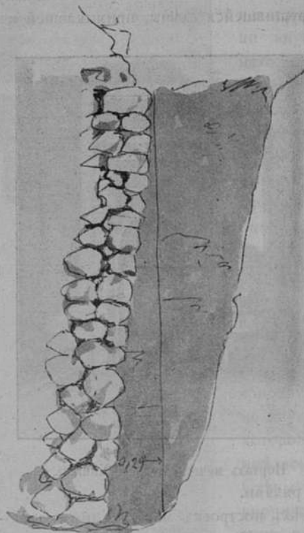
Фундаментъ минарета.
