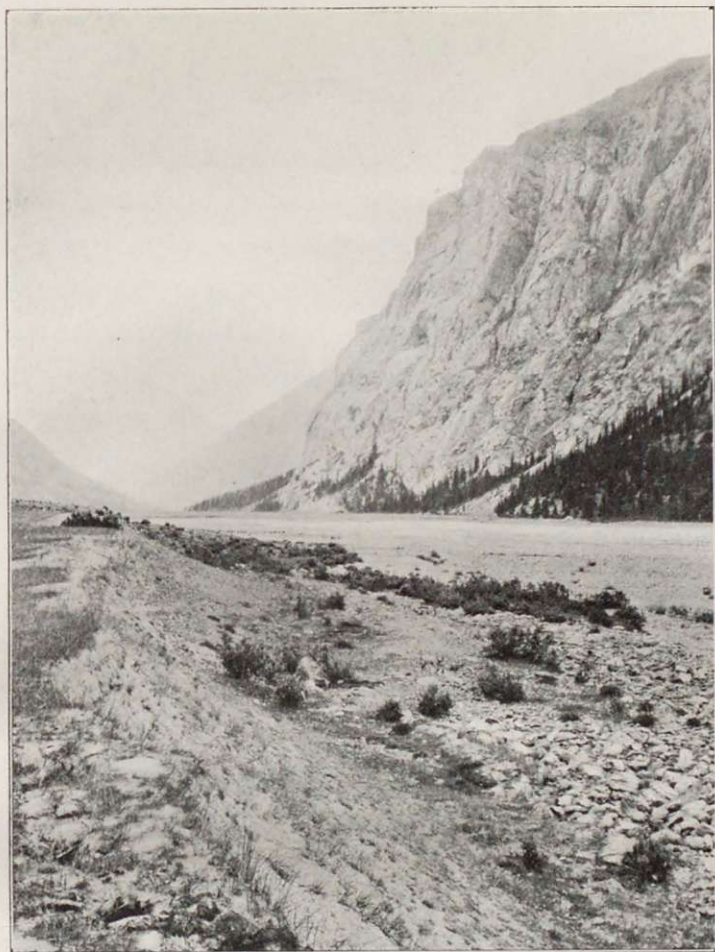
Рис. 7. Долина р. Каинды
