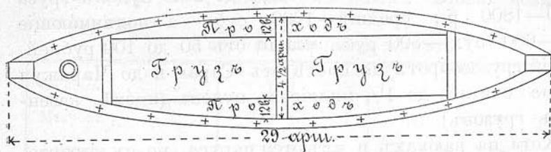
Соединеніе бруссовъ.
