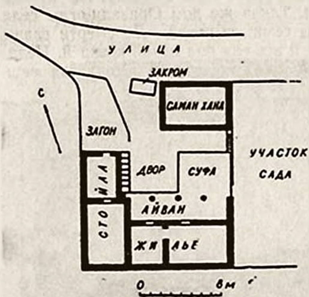
Рис. 40. Дом Косе Мурад-оглы. План
