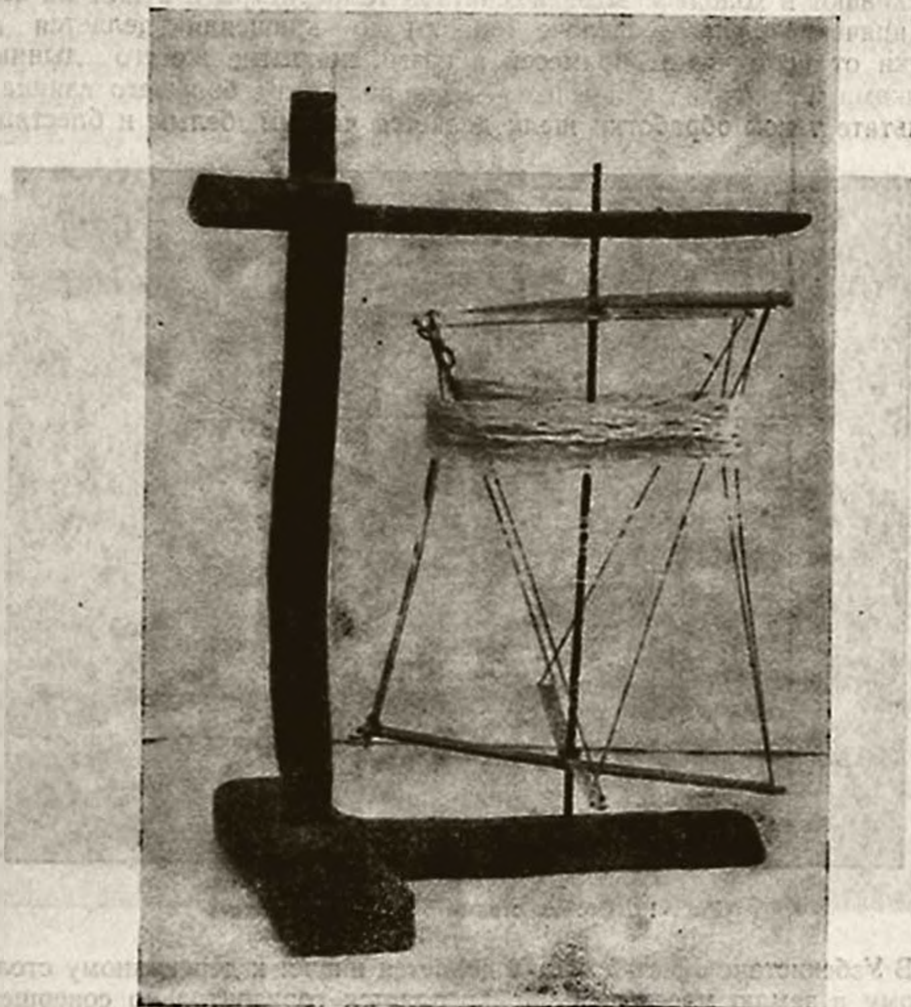
Рис. 18. Инструмент для обработки шелка „перрик“.
