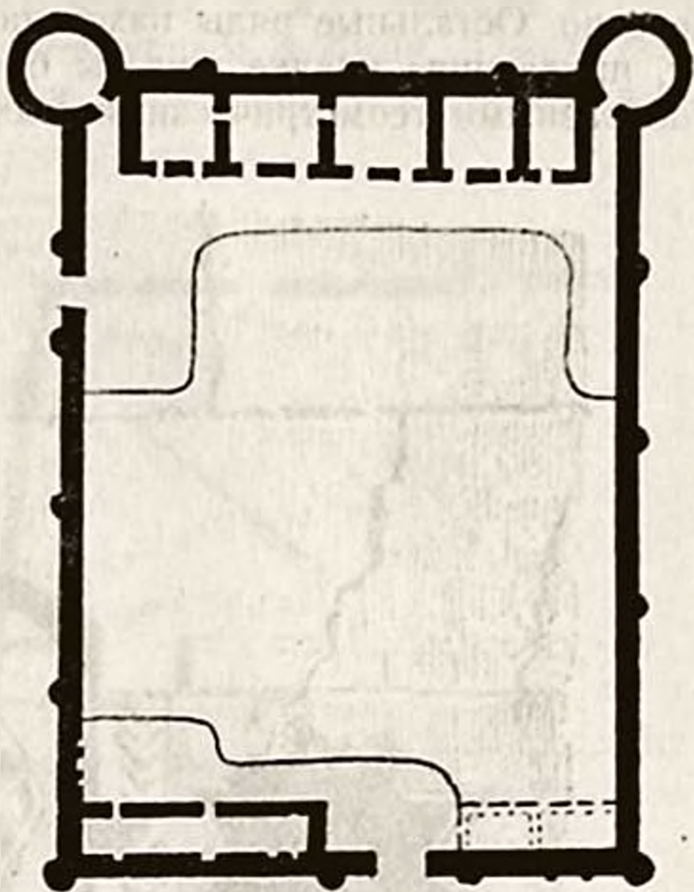
Рис. 21. Фараб. Ховаы Бабо-Назар-бая. План.
