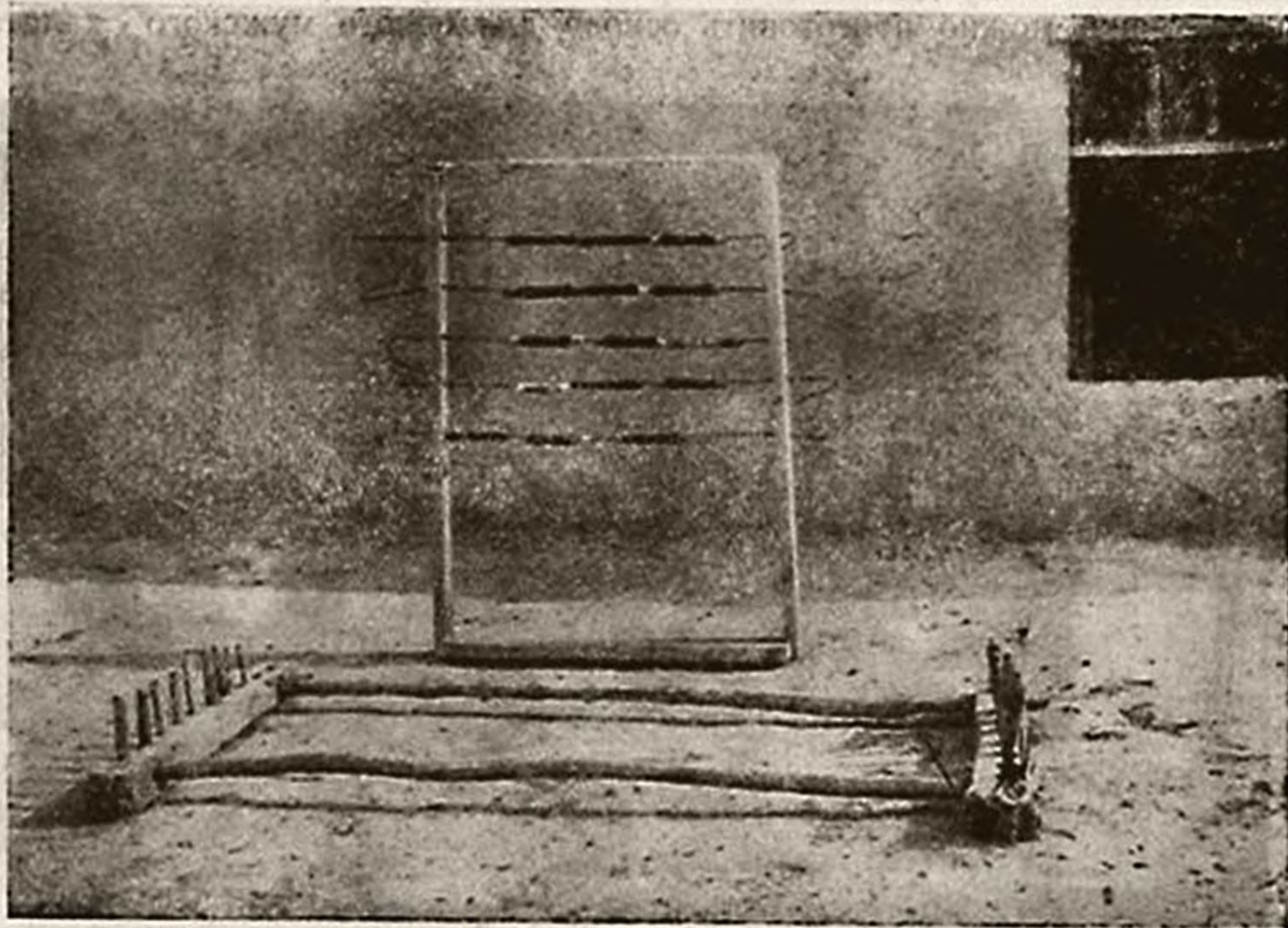
Рис. 23. Станок для подготовки основы тканья «тар-йувирден».
