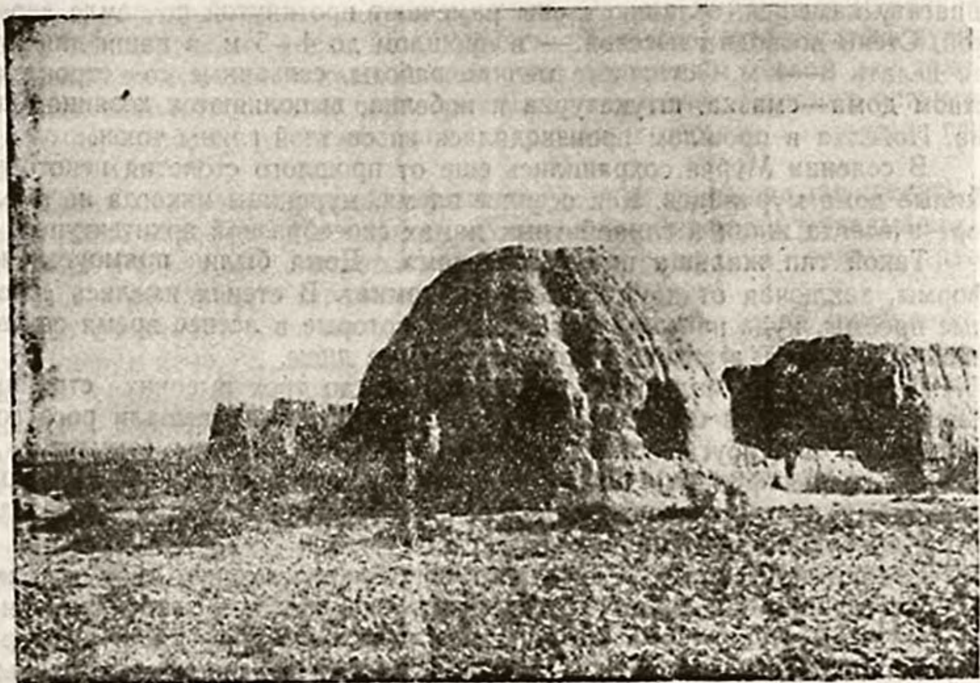
Рис. 34. Купальное перекрытие худжры Дез-кала.
