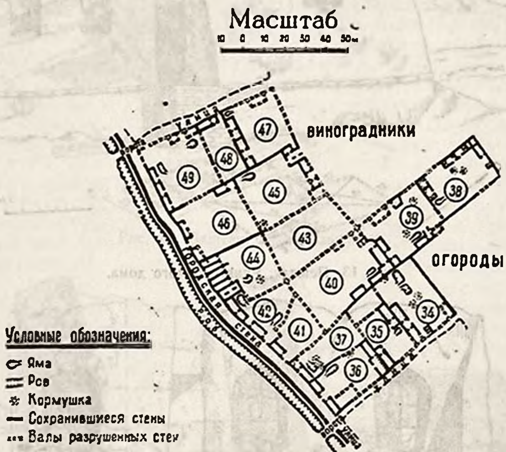
Рис. 12. Пештак. Планировка квартала.
