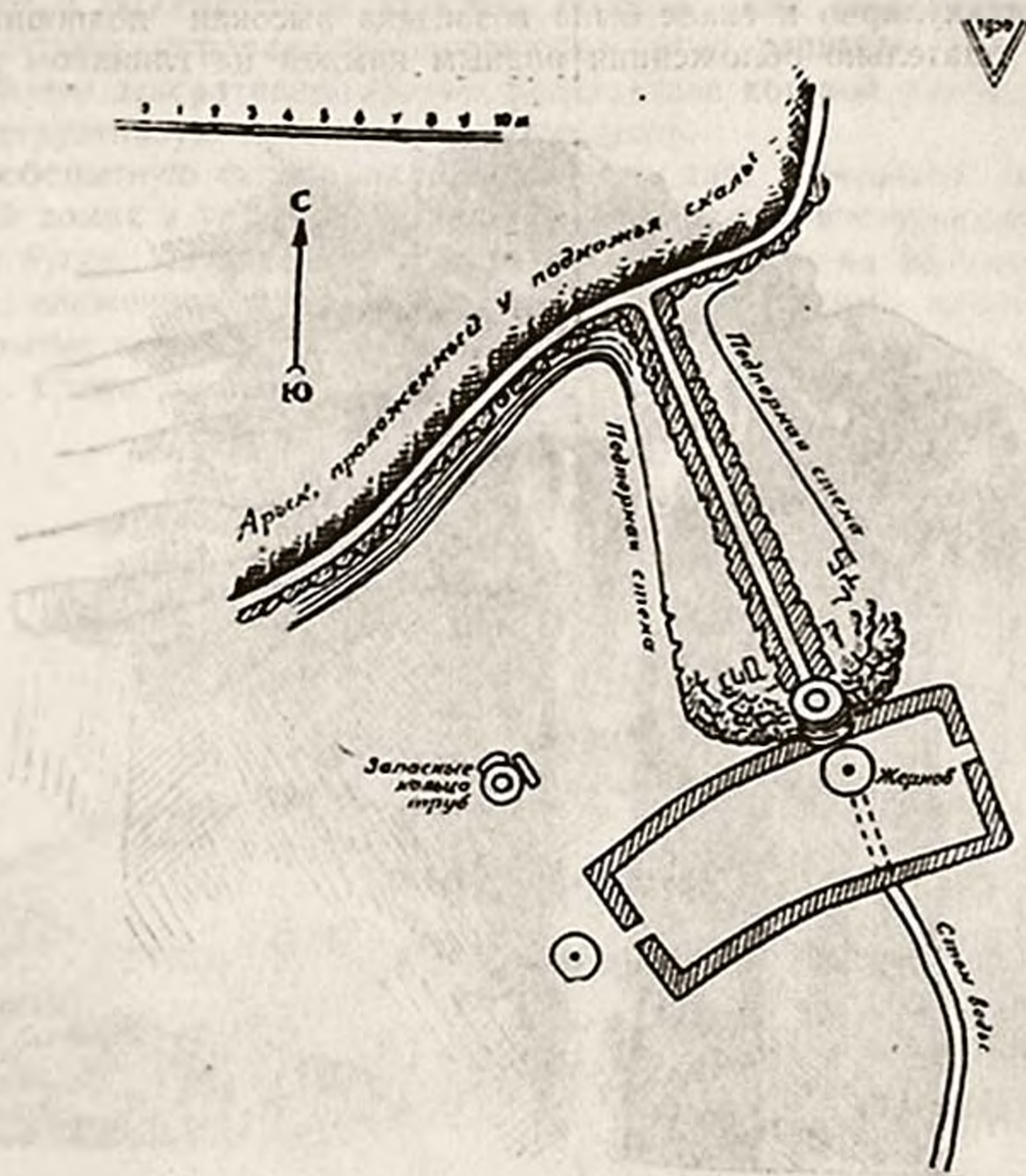
Рис. 10. План мельницы.
