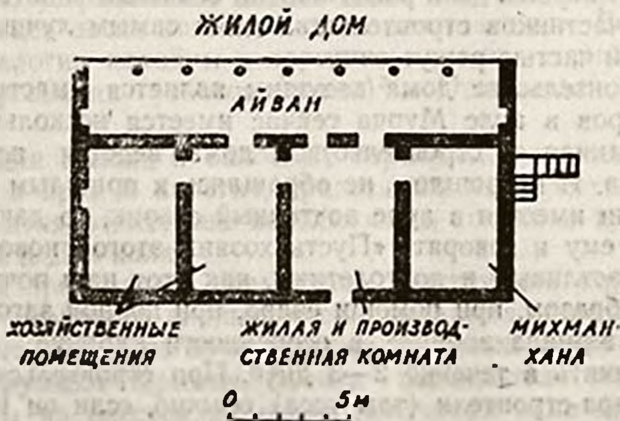
Рис. 32. Усадьба Девлет Юзбаша Оглы. Гялан.
