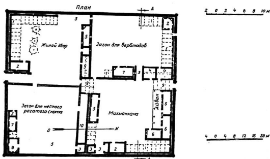
Рис. 50. Кувакский район. Ховлы Баба Нарзабая. План участка и разрез 1 — навес для лошадей; 2 — амбунчик; 3 — хозяйственный склад; 4 — амбар; 5 — жилое помещение хозяев; 6 — жилое помещение для гостей; 7 — жилое помещение для пастухов; 8 — маслобойка; 9 — крытый проход; 10 — коровник
