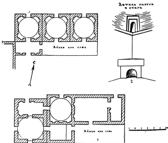
Рис. 28. Марыйская область. Старые жилые дома (сельсовет Чарлык-яб, колхоз им. Ворошилова)
