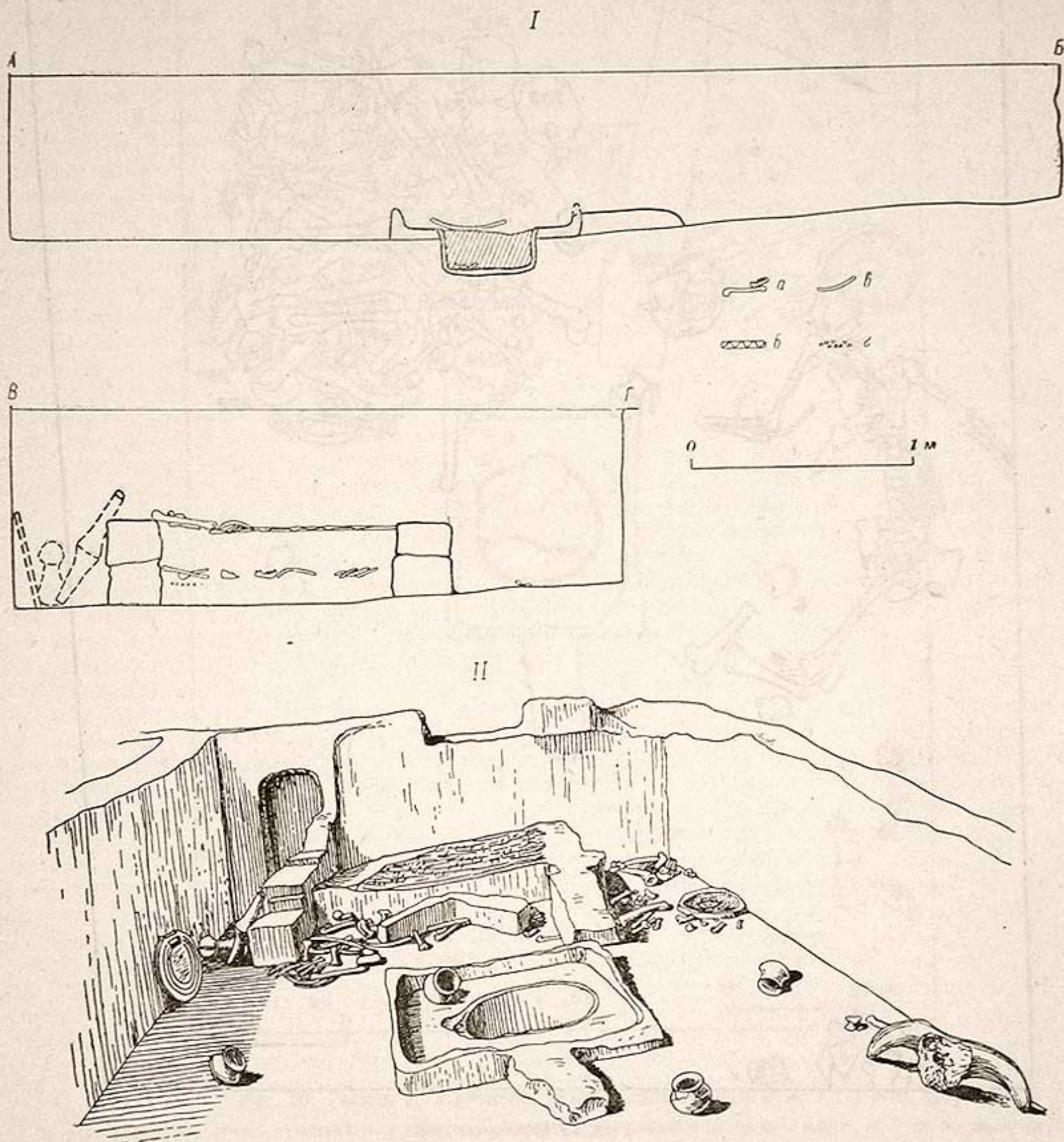
Рис. 21. Раскоп 7. Продольный и поперечный разрезы пом. 7 (I). Аксонометрия (II).
