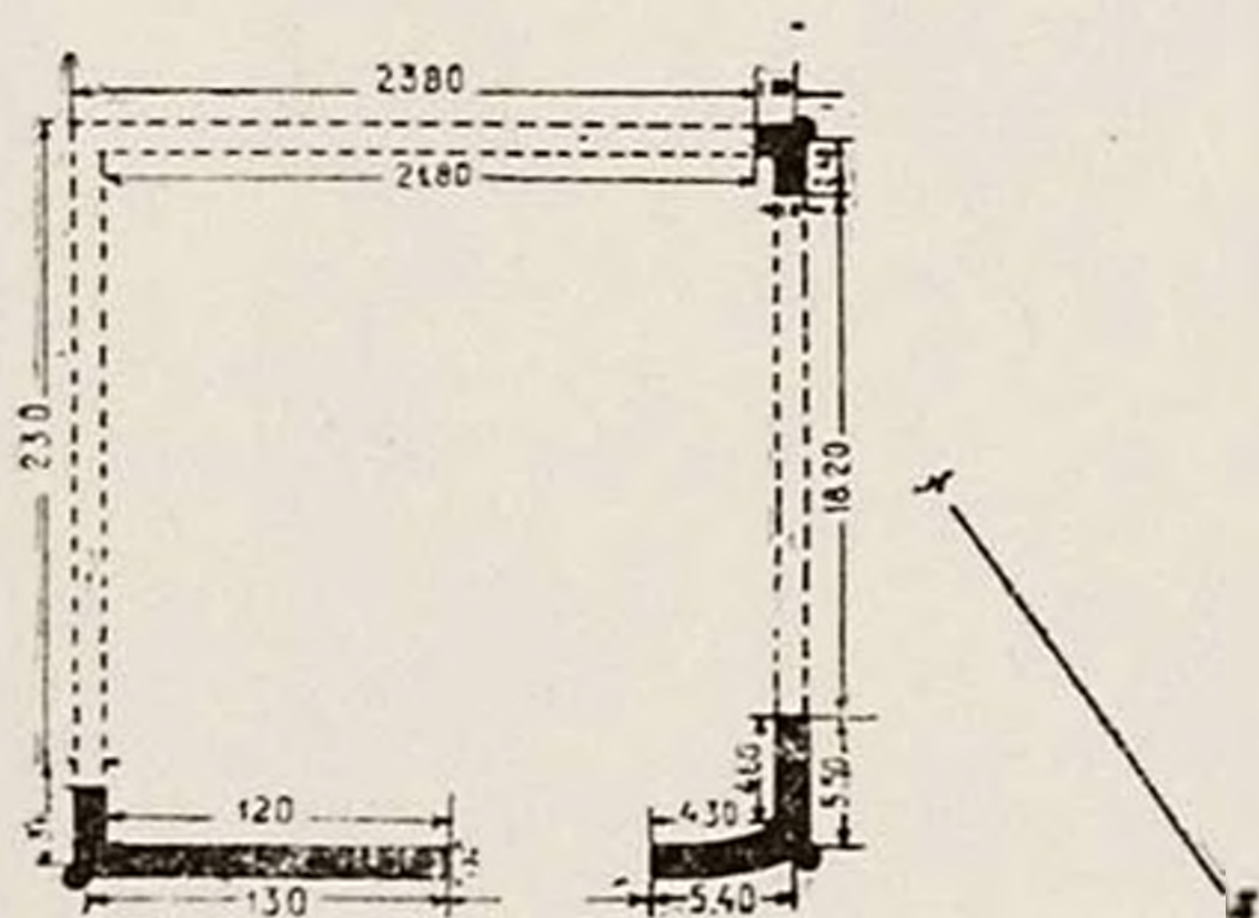
Рис. 5. Планы кала (обмеры М. С. Мерцисева).
