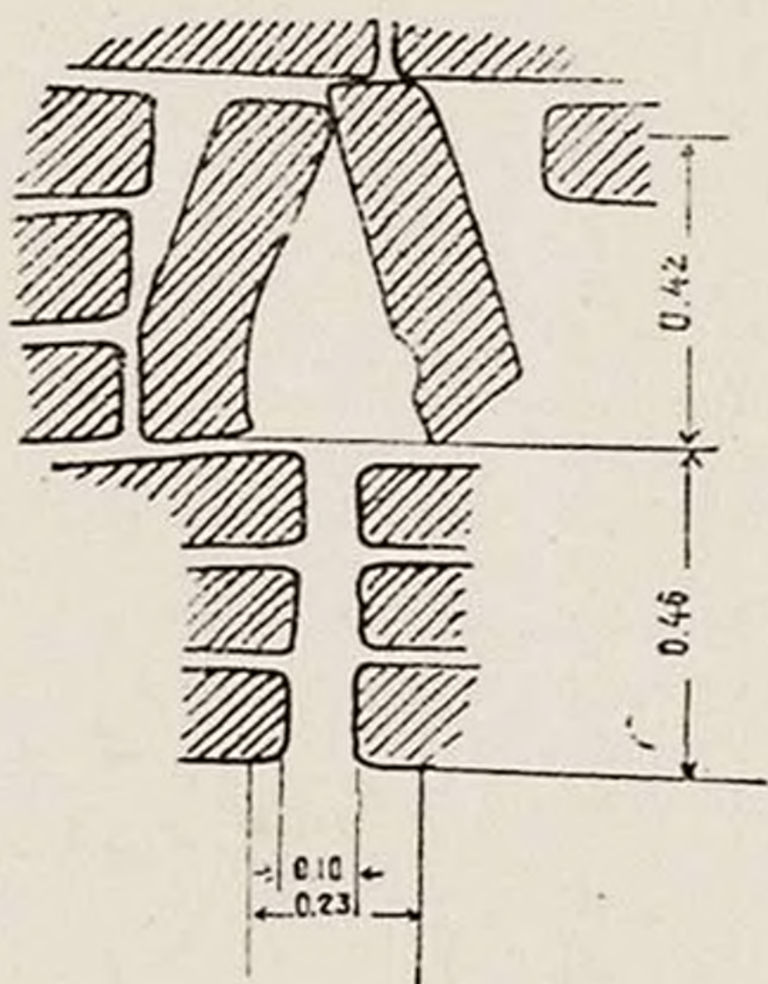
Рис. 9. Ложная бойница.
