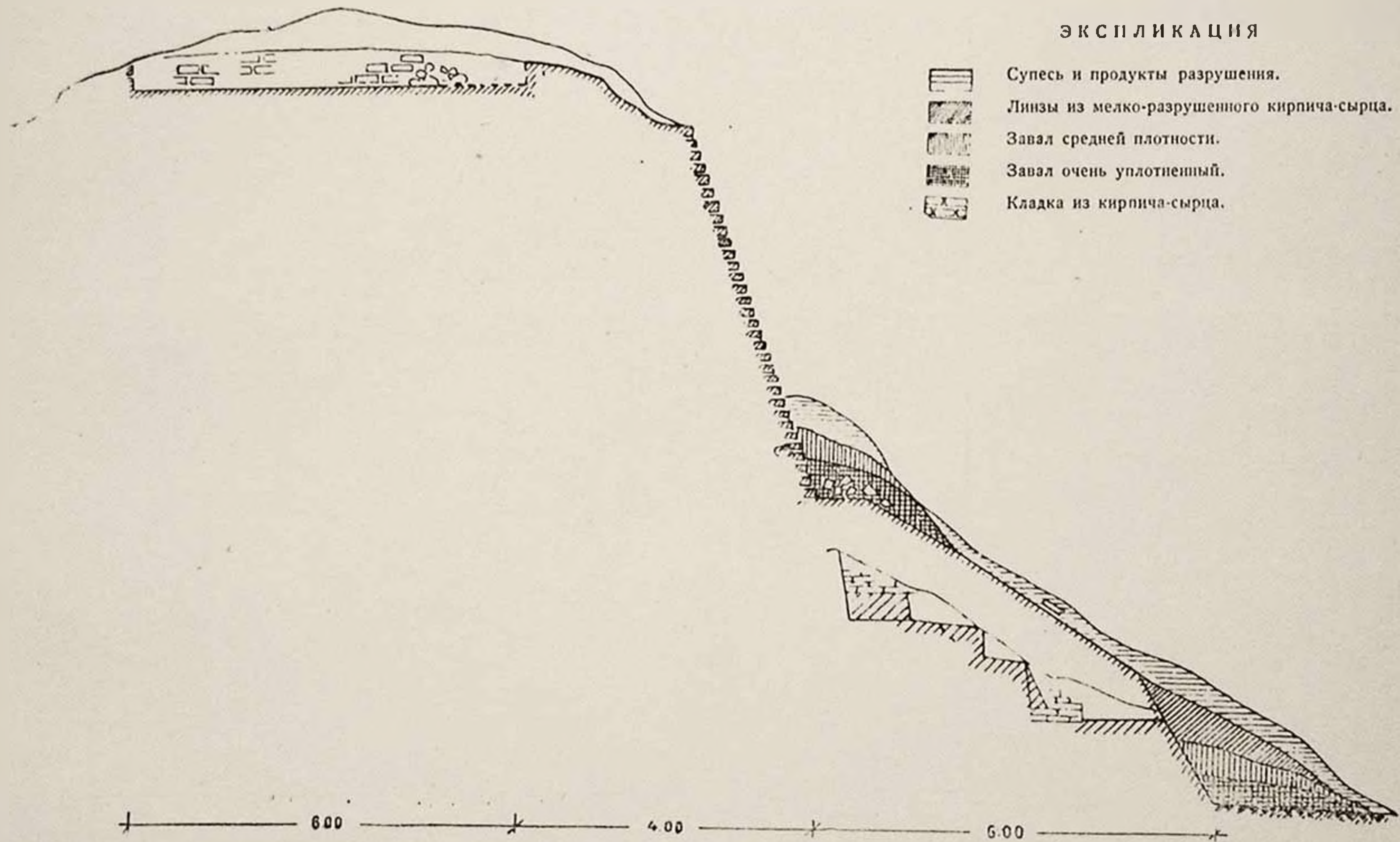
Рис. 7. Профиль баши № 1.
