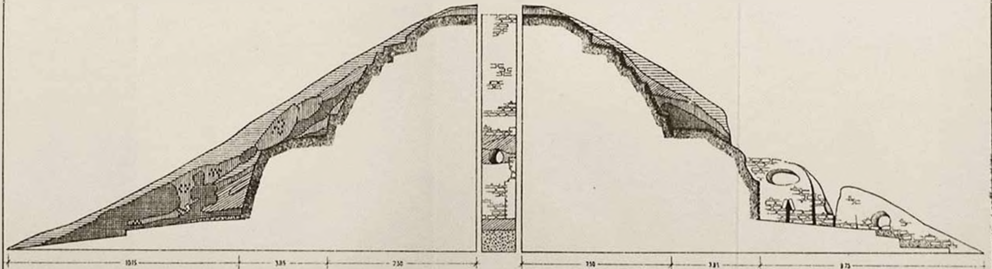
Развертка профилей разреза стены с восточной стороны
