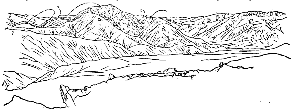
Рис. 12. Геологическое строение хребта Карнай-тарты. Рисовано на восток с водораздельного гребня к Сасыку Ак-байтальскому. Две вершины на горизонте между пунктиром и знаком Cr 2 — хребет Муз-таг-ата (на расстоянии около 130 км). (Рисовал А. В. Хабаков).
