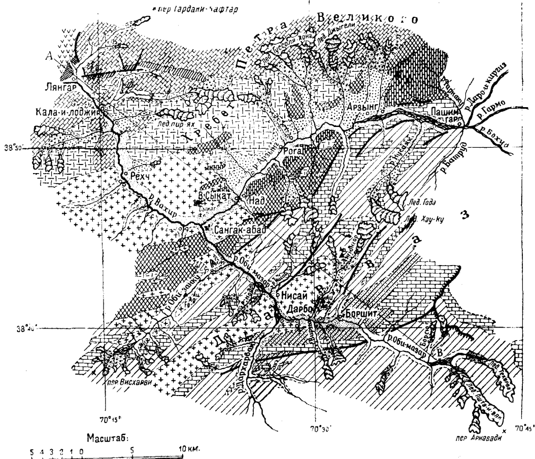
Геологическая карта Вахио-и-болё. (Составл. А. Г. Вологдин).
