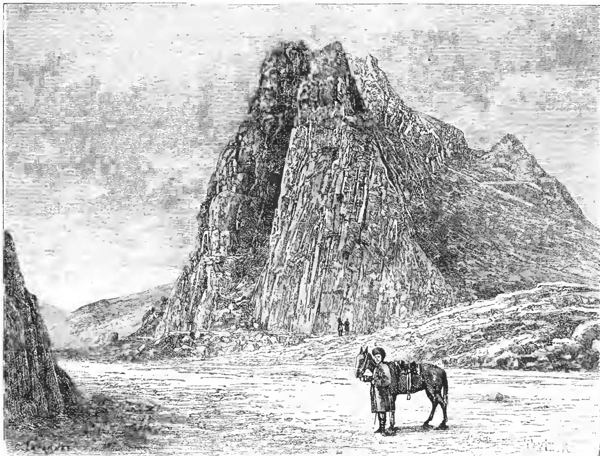
5. Тамерлановы ворота близъ г. Самаркандъ. Рис. Тайлоръ, грав. Лаплагтъ.
