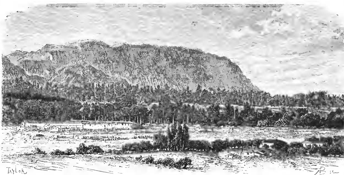
5. Русская стоянка въ укрѣпленіи Учъ (Конанъ). Рис. Тайлоръ, грав. Барбанъ.
