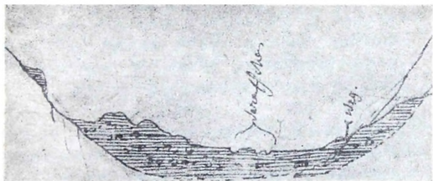
Рис. 7. Долина реки Зеравшан на восток от г. Пенджикента (рис. А. Лемана).
