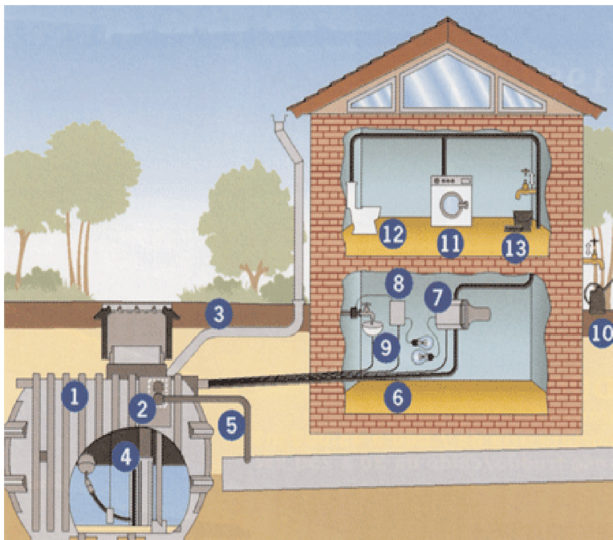
Рисунок 5. Схема системы регенерации дождевой воды
